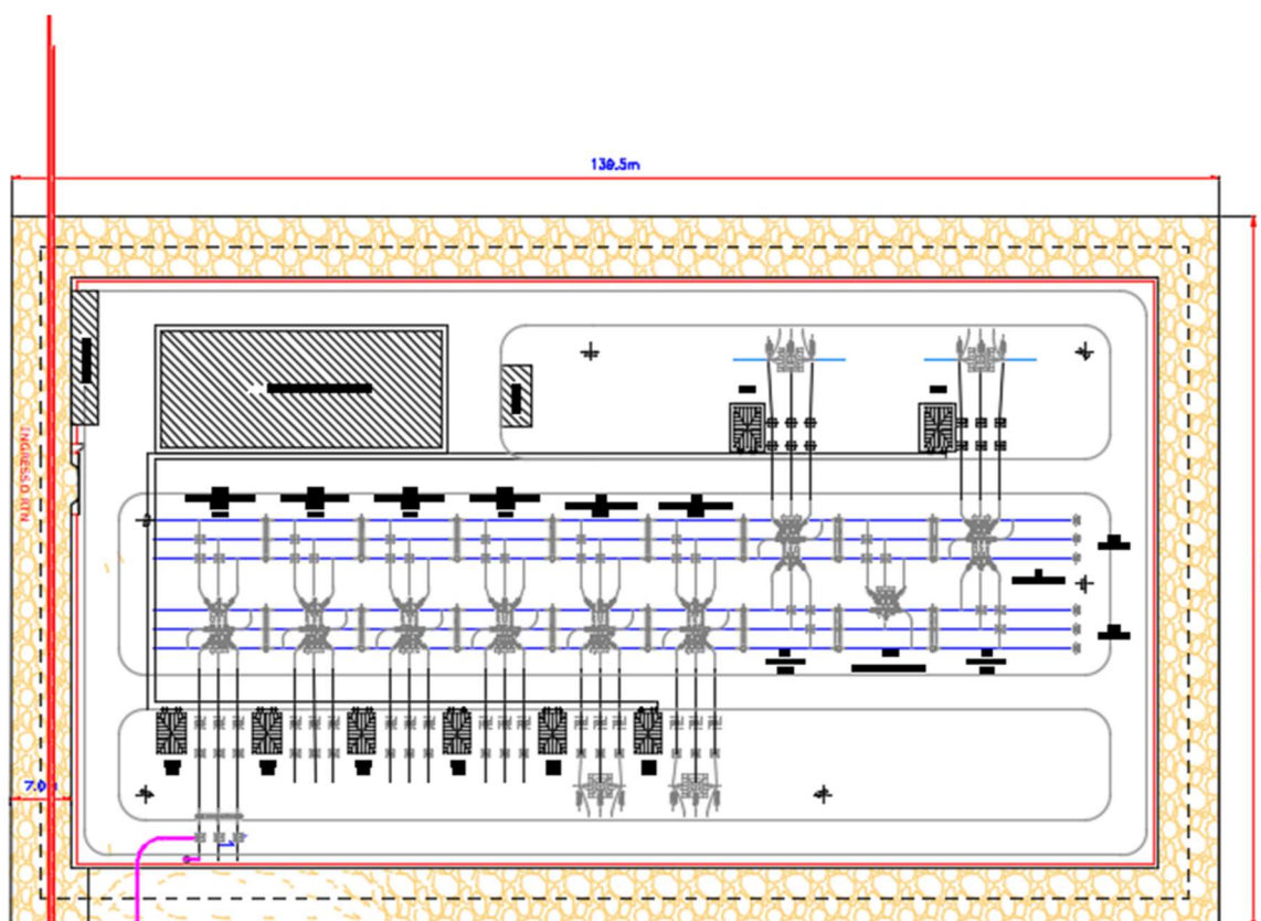
Planimetria sottostazione elettrica di utenza
