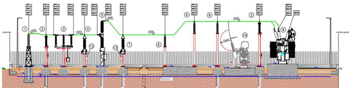
Sezione elettromeccanica della SSE produttore
