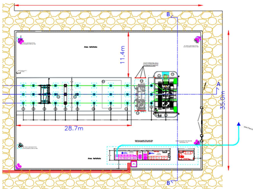
Planimetria elettromeccanica della SSE produttore
