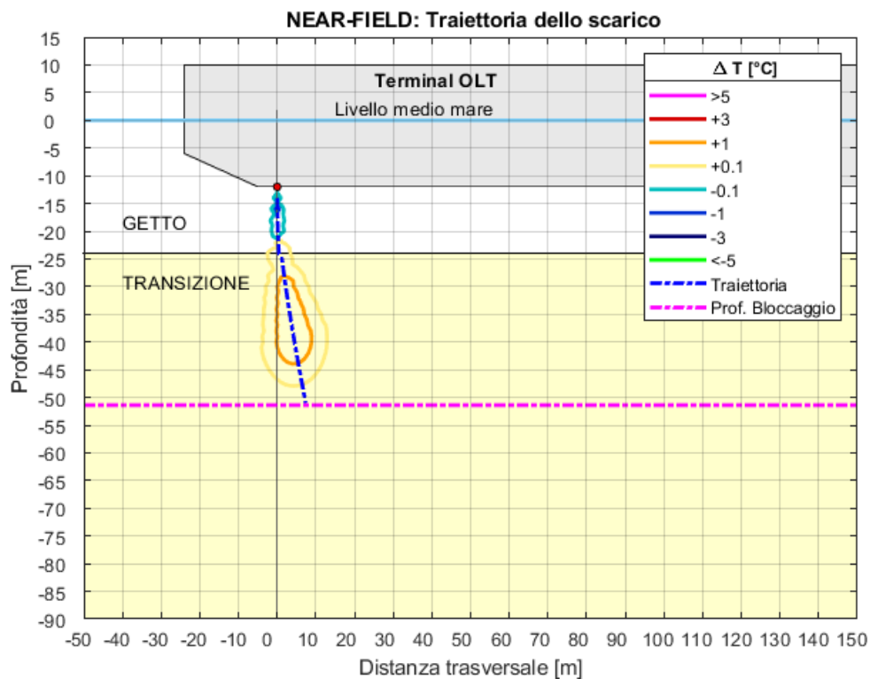
Figura 12 – Risultati Modello Dispensivo, Scenario Giugno 2023
