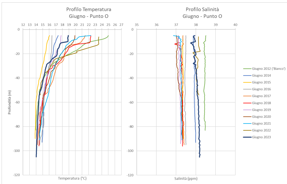
Figura 10 – Confronto tra Campionamenti effettuati nel Mese di Giugno 2012, 2014, 2015, 2016, 2017, 2018, 2019, 2020, 2021, 2022 e 2023 al Punto O
