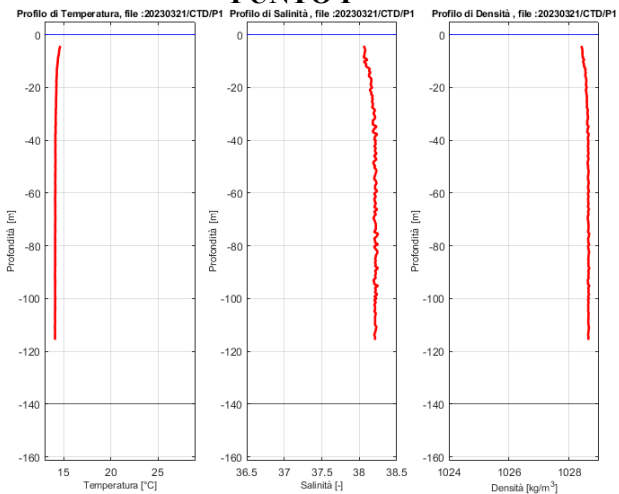
Figura 4 – Profili di Temperatura (sinistra), Salinità (centro) e Densità (destra) misurati in O in Marzo 2023
