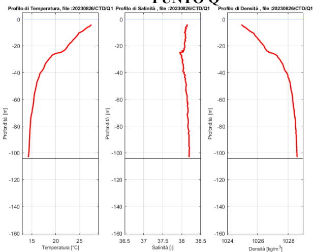
Figura 6 – Profili di Temperatura (sinistra), Salinità (centro) e Densità (destra) misurati in P e Q in Agosto 2023
