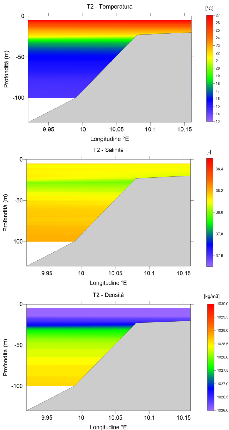
Figura 9 – Transetto T2 – Agosto 2023 – Valori Caratteristici della Temperatura (Sopra) Salinità (Centro) e Densità (Sotto)
