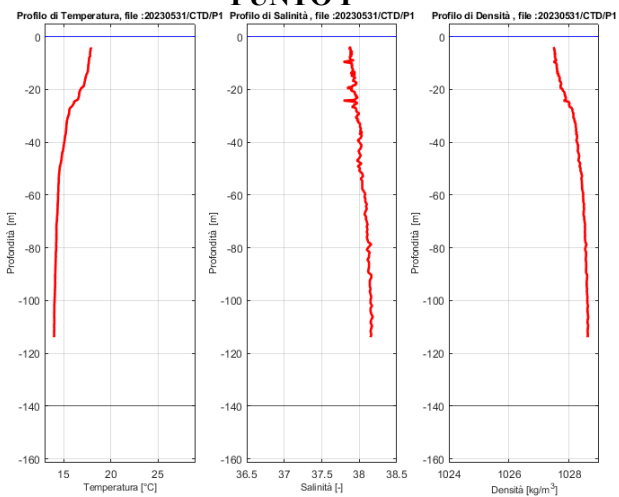
Figura 5 – Profili di Temperatura (sinistra), Salinità (centro) e Densità (destra) misurati in P e Q in Giugno 2023
