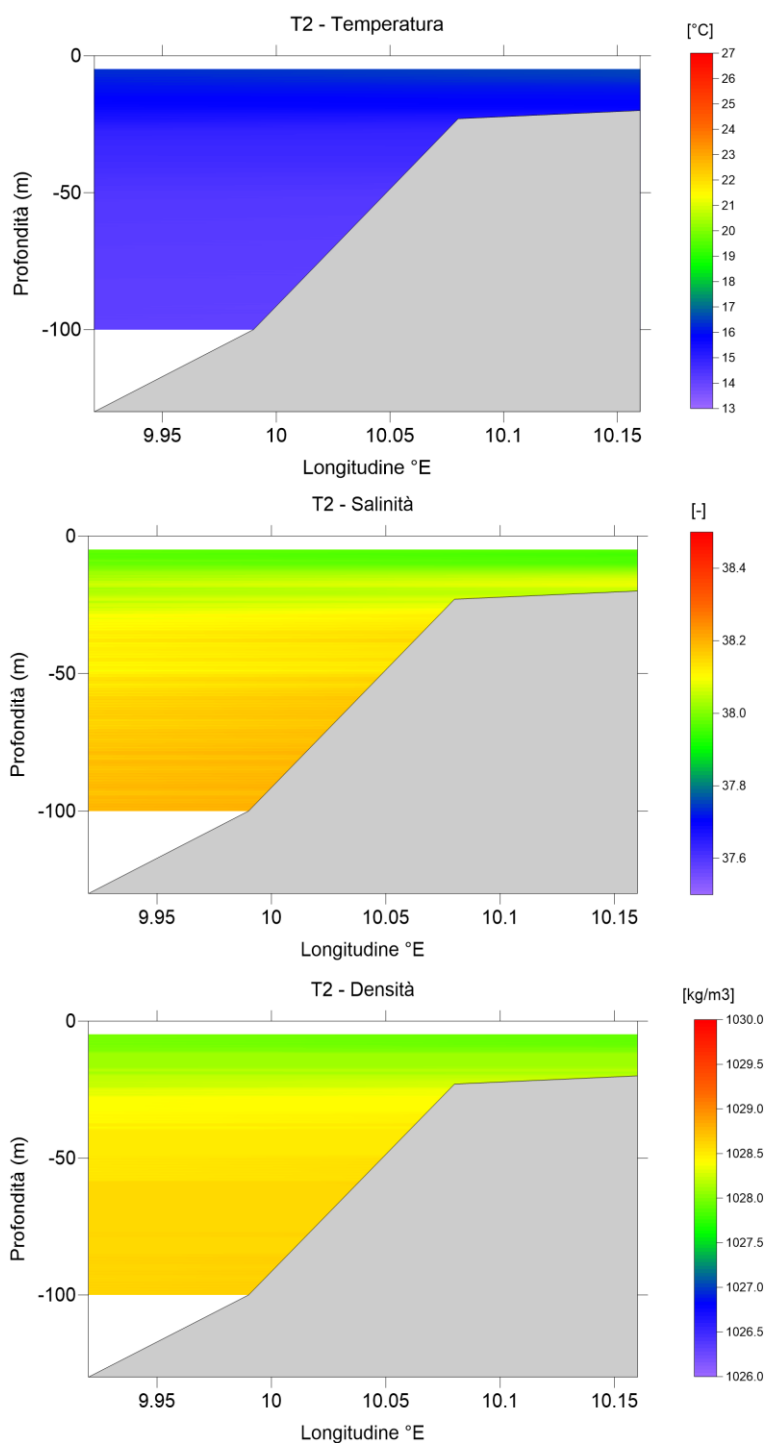
Figura 7 – Transetto T2 – Marzo 2023 – Valori Caratteristici della Temperatura (Sopra) Salinità (Centro) e Densità (Sotto)
