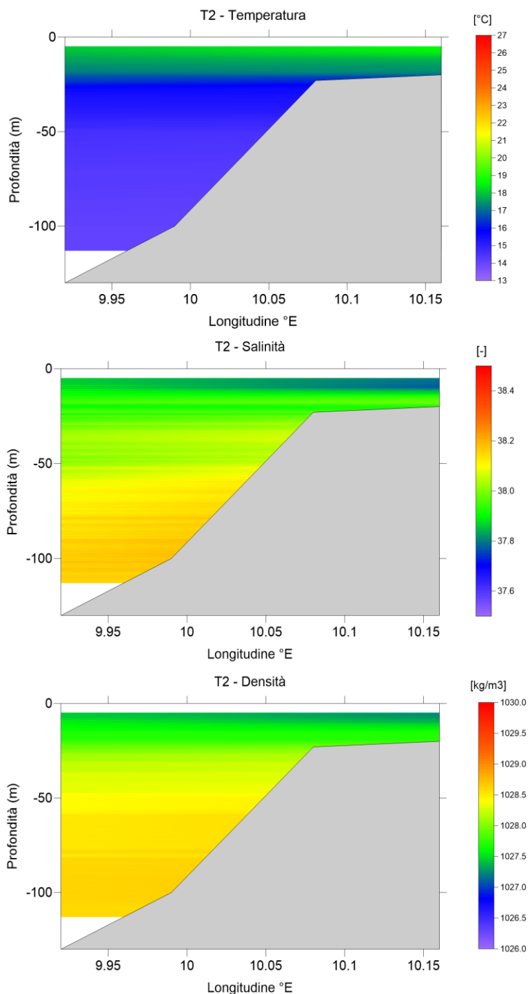
Figura 8 – Transetto T2 – Giugno 2023 – Valori Caratteristici della Temperatura (Sopra) Salinità (Centro) e Densità (Sotto)
