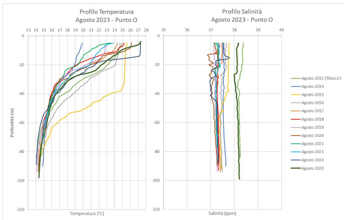
Figura 11 – Confronto tra Campionamenti effettuati nel Mese di Agosto 2012, 2014, 2015, 2016, 2017, 2018, 2019, 2020, 2021, 2022, e 2023 al Punto O
