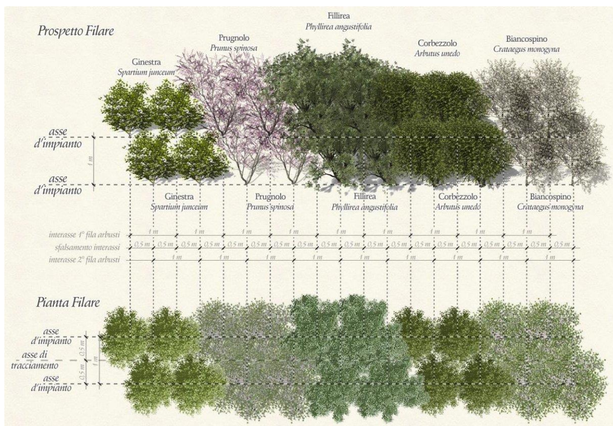
figura 4 stralcio sezione e planimetria siepe
