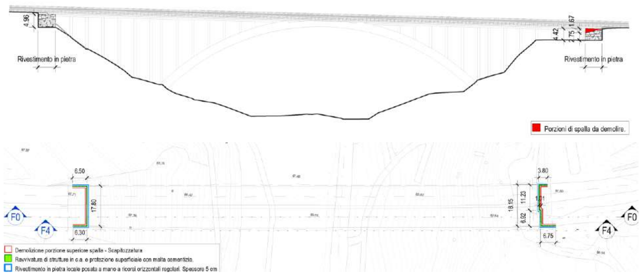
Figura 6.1: Individuazione aree da demolire Spalle e rivestimento in pietra
