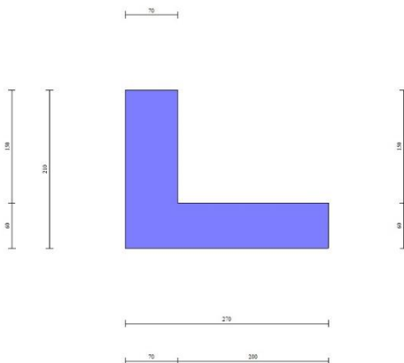
Fig. 1 - Sezione quotata del muro
