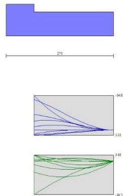
Fig. 9 - Fondazione (Inviluppo)
