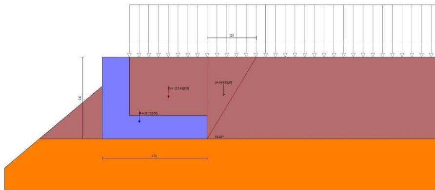
Fig. 10 - Cuneo di spinta (combinazione statica) (Combinazione n° 1)
