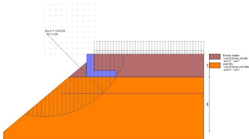
Figura 20: Stabilità fronte di scavo - Cerchio critico (Combinazione n° 4)_FS=2.294
