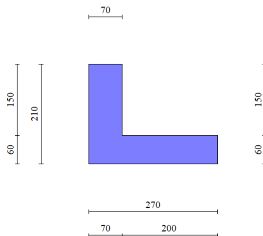
Figura 15: Geometria del muro di sostegno: sezione trasversale
