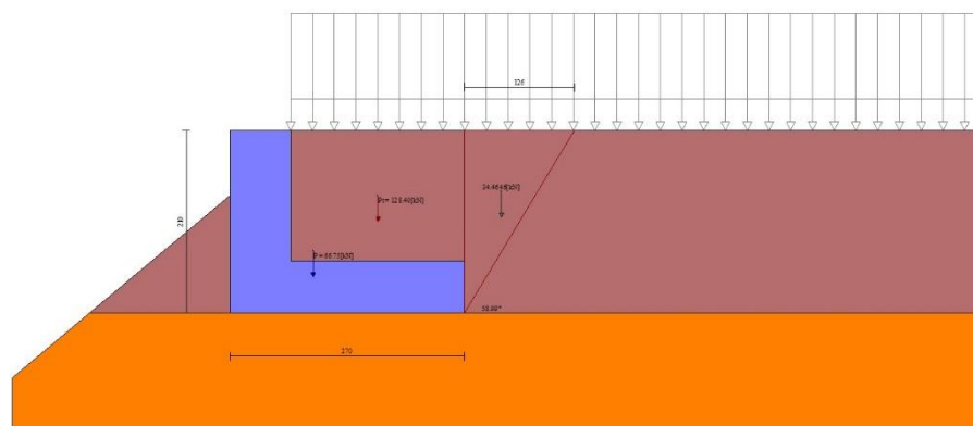
Fig. 3 - Cuneo di spinta (combinazione statica) (Combinazione n° 1)
