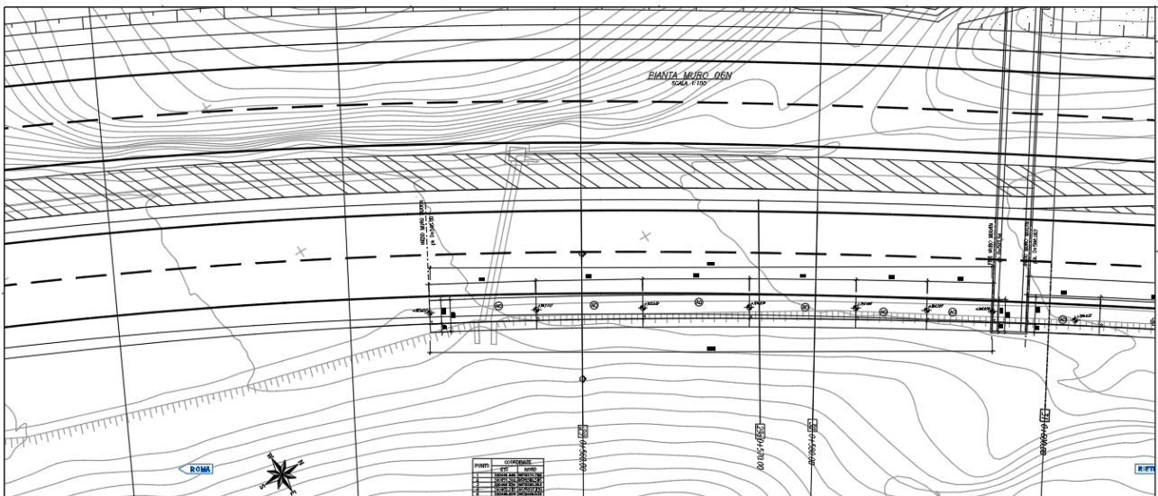
Figura 2: planimetria di progetto
