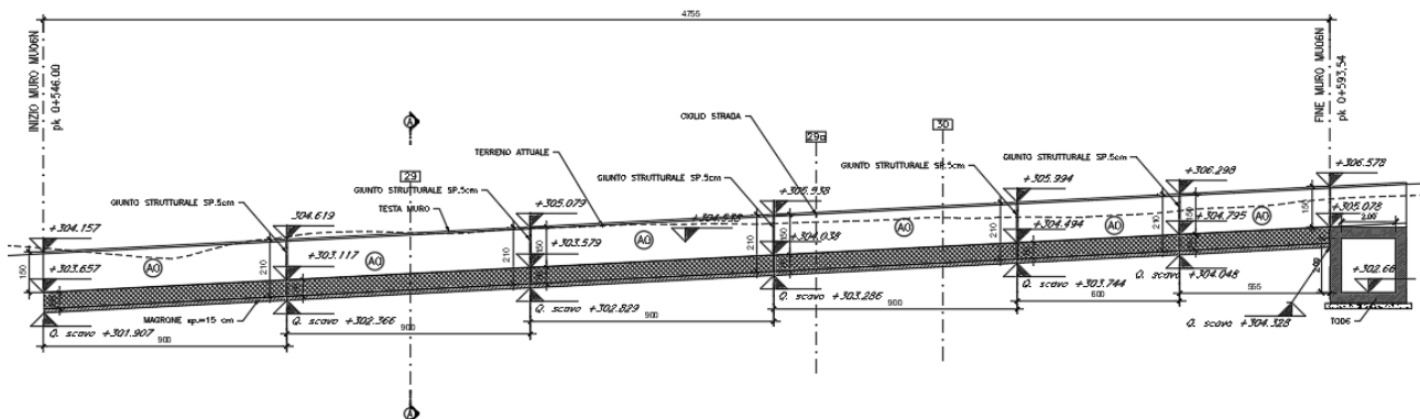
Figura 3: profilo longitudinale
