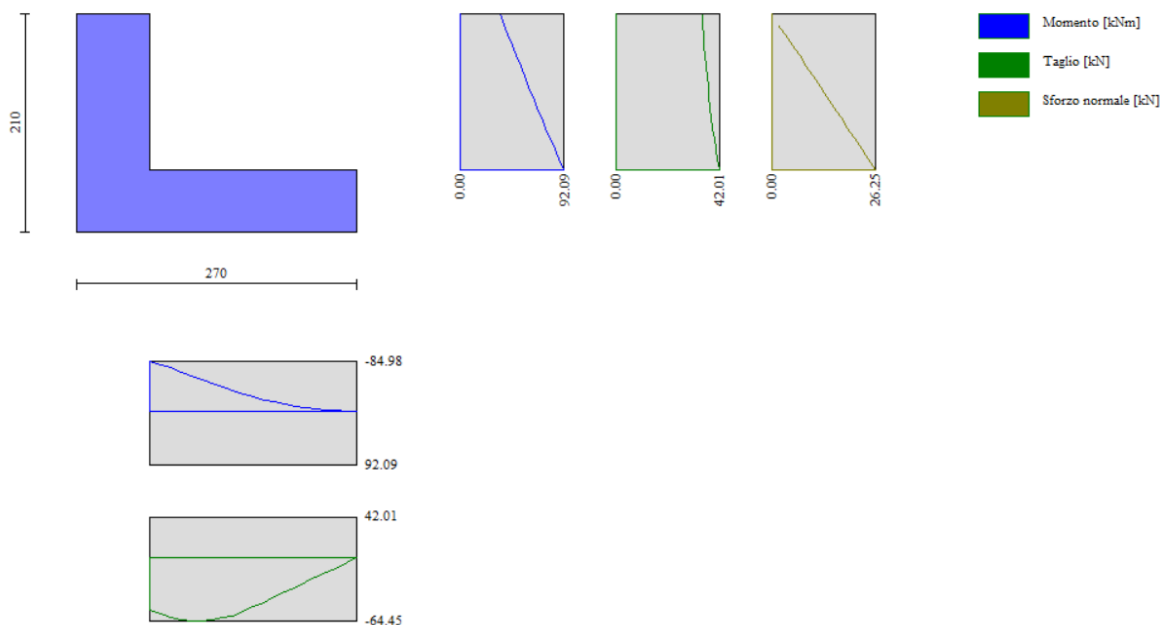
Figura 19: Involuppo diagrammi sollecitazioni – condizione urto
