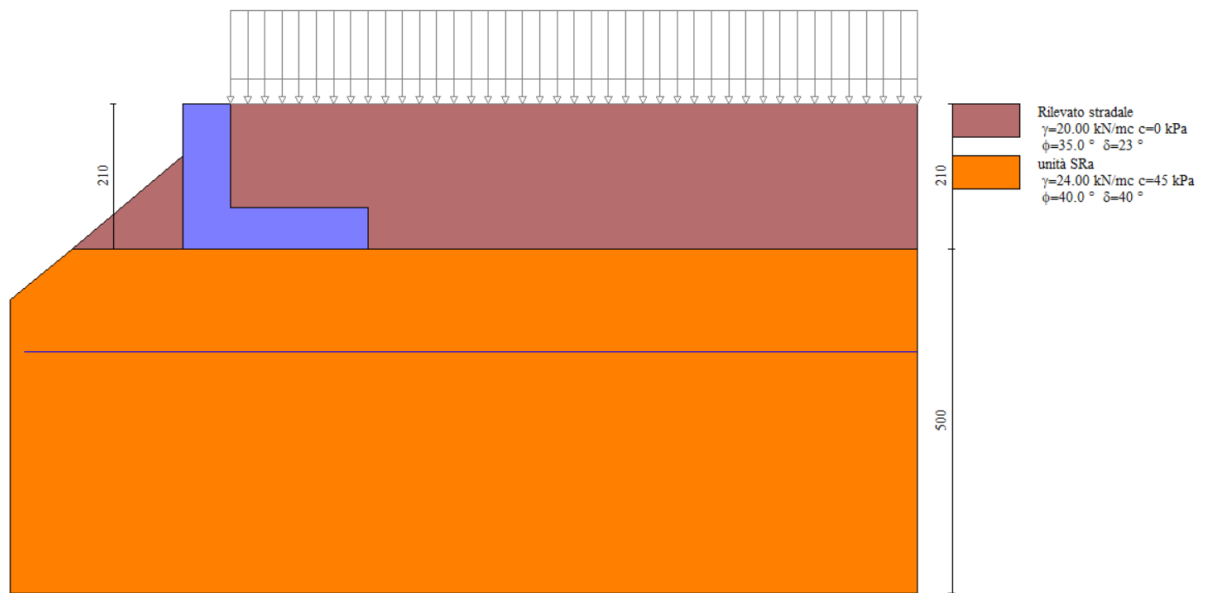
Figura 14: modello di calcolo muro tipologico A0
