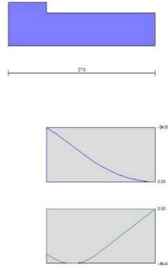
Fig. 7 - Fondazione (Inviluppo)
