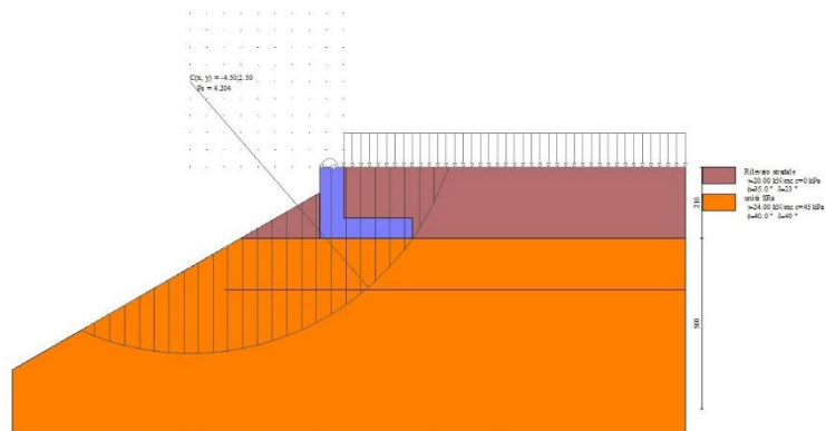
Fig. 10 - Stabilità fronte di scavo - Cerchio critico (Combinazione n° 2)
