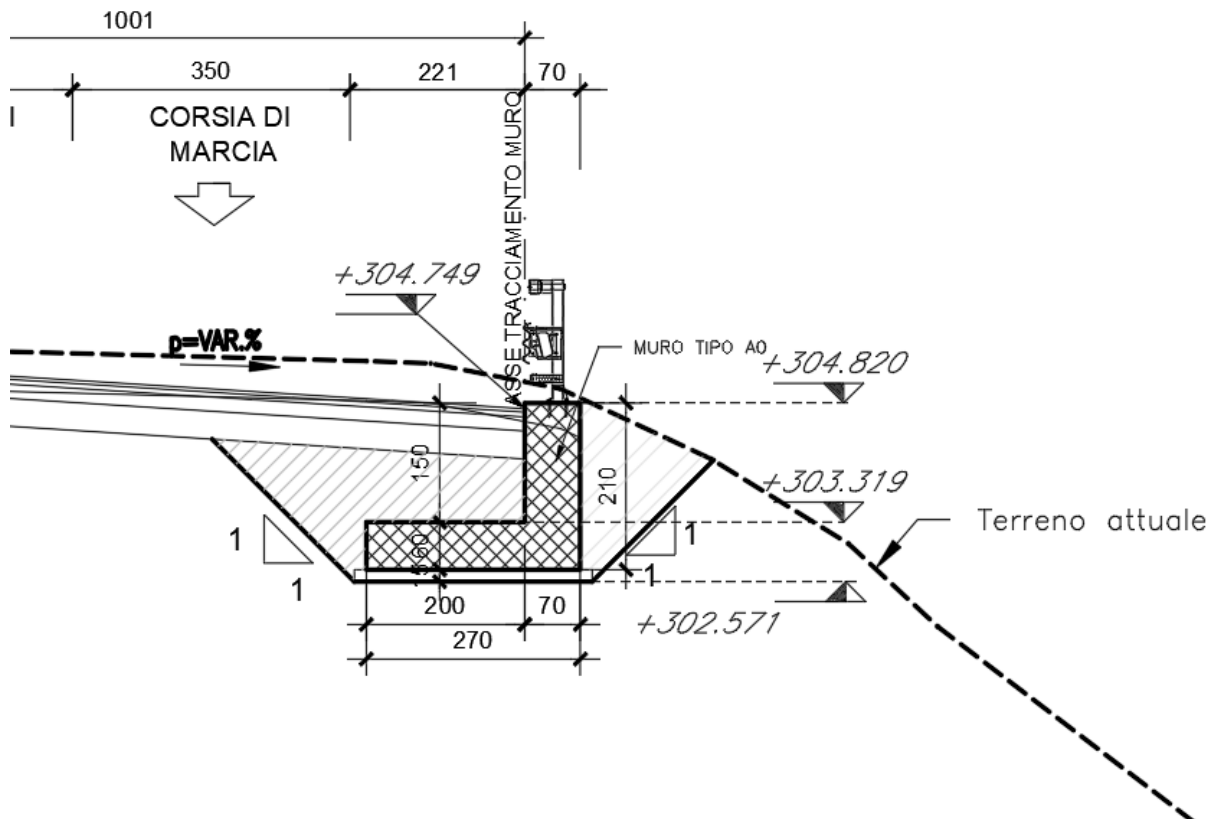
Figura 4: sezione trasversale muro tipologico A0
