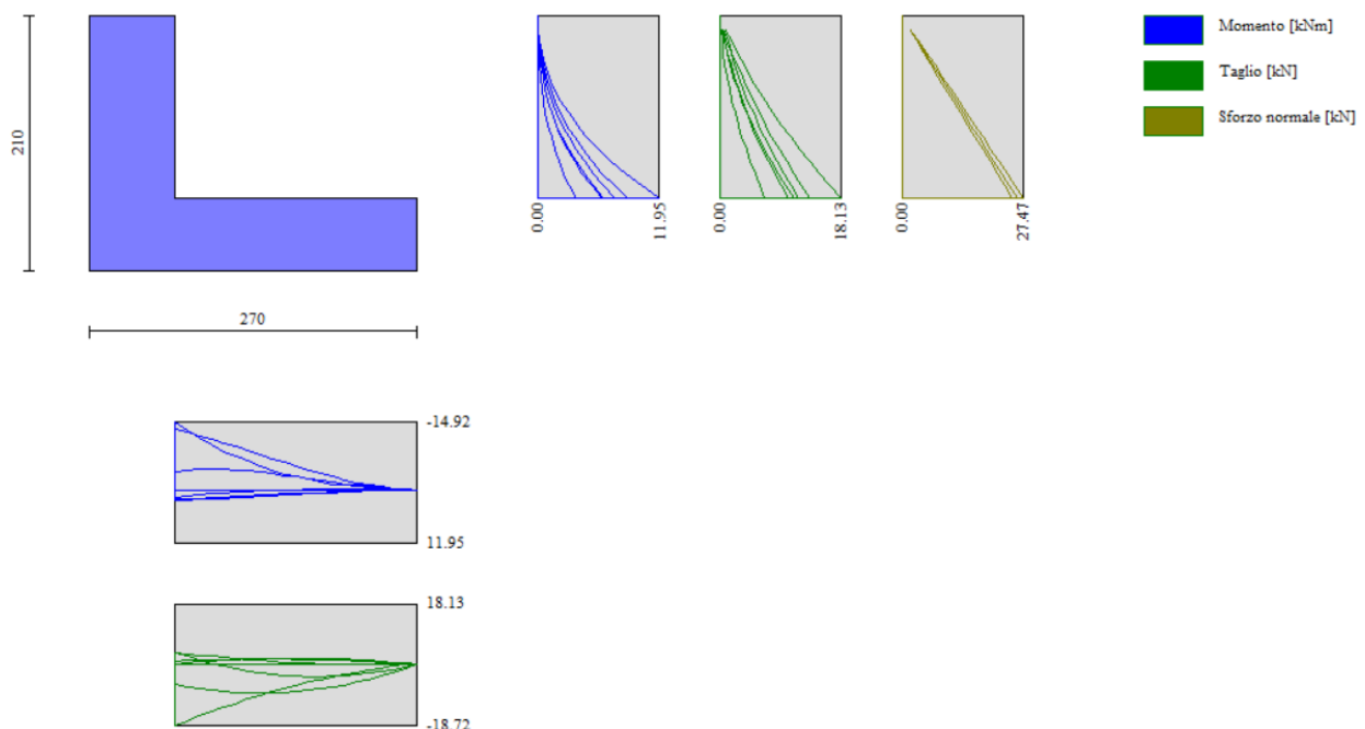
Figura 18: Involuppo diagrammi sollecitazioni- condizioni statiche e sismiche
