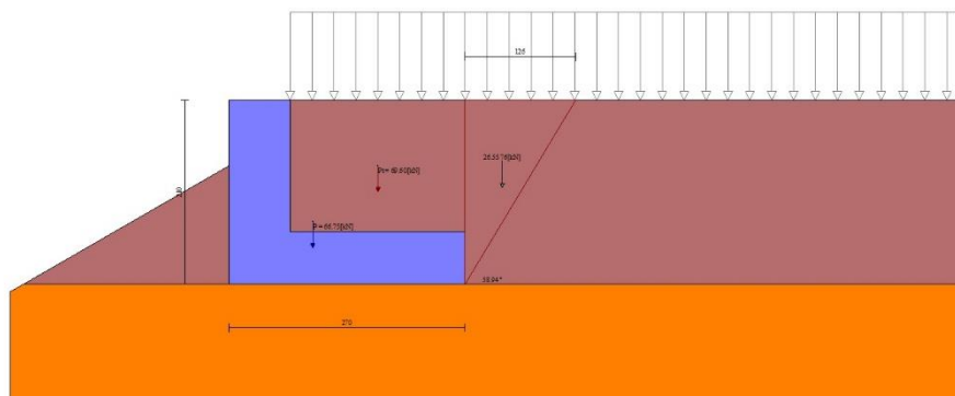
Fig. 8 - Cuneo di spinta (combinazione statica) (Combinazione n° 1)
