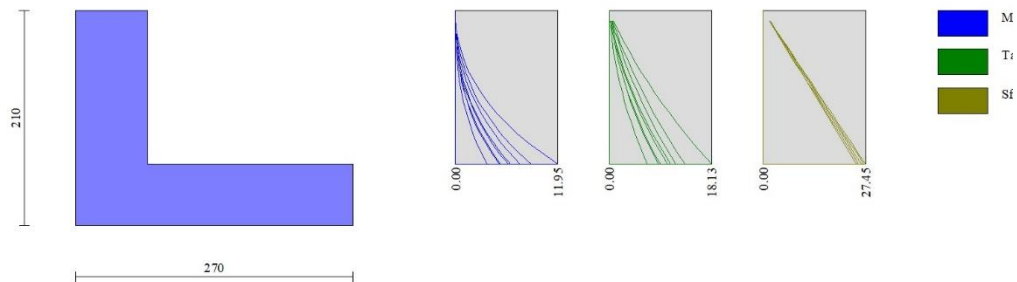
Fig. 8 - Paramento (Inviluppo)
