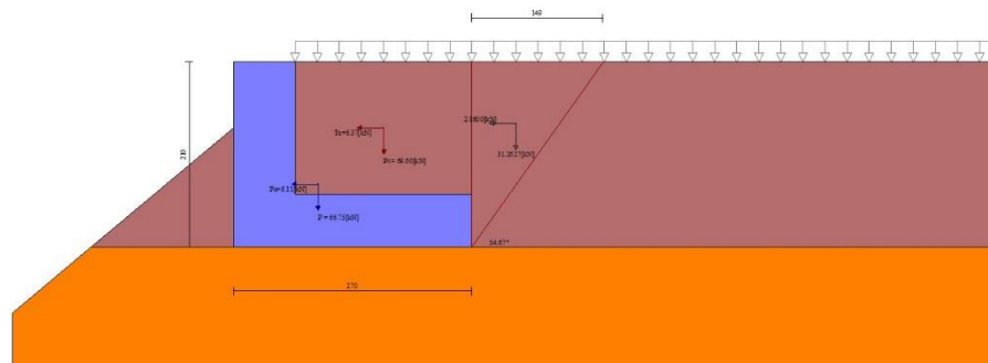
Fig. 5 - Cuneo di spinta (combinazione sismica) (Combinazione n° 2)
