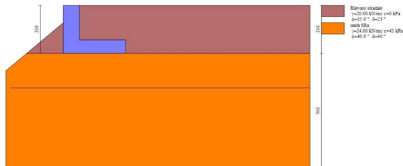
Fig. 2 - Stratigrafia
