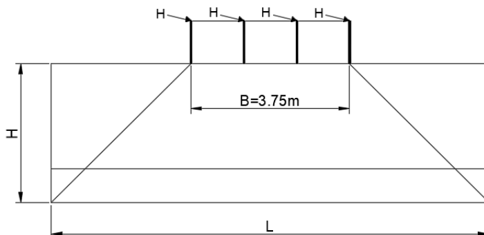
Figura 12: schema di redistribuzione del carico d'urto
