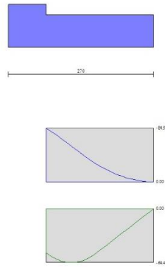
Fig. 12 - Fondazione
