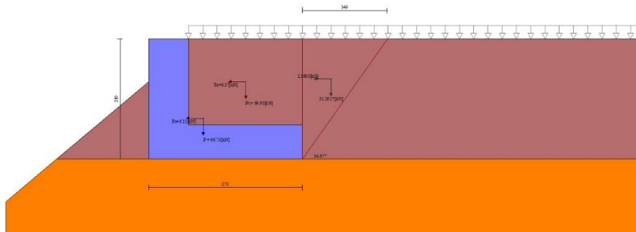
Fig. 12 - Cuneo di spinta (combinazione sismica) (Combinazione n° 2)
