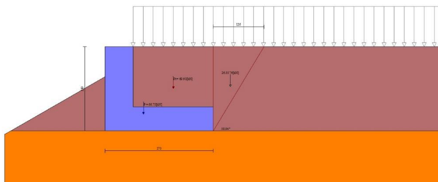
Fig. 3 - Cuneo di spinta (combinazione statica) (Combinazione n° 1)
