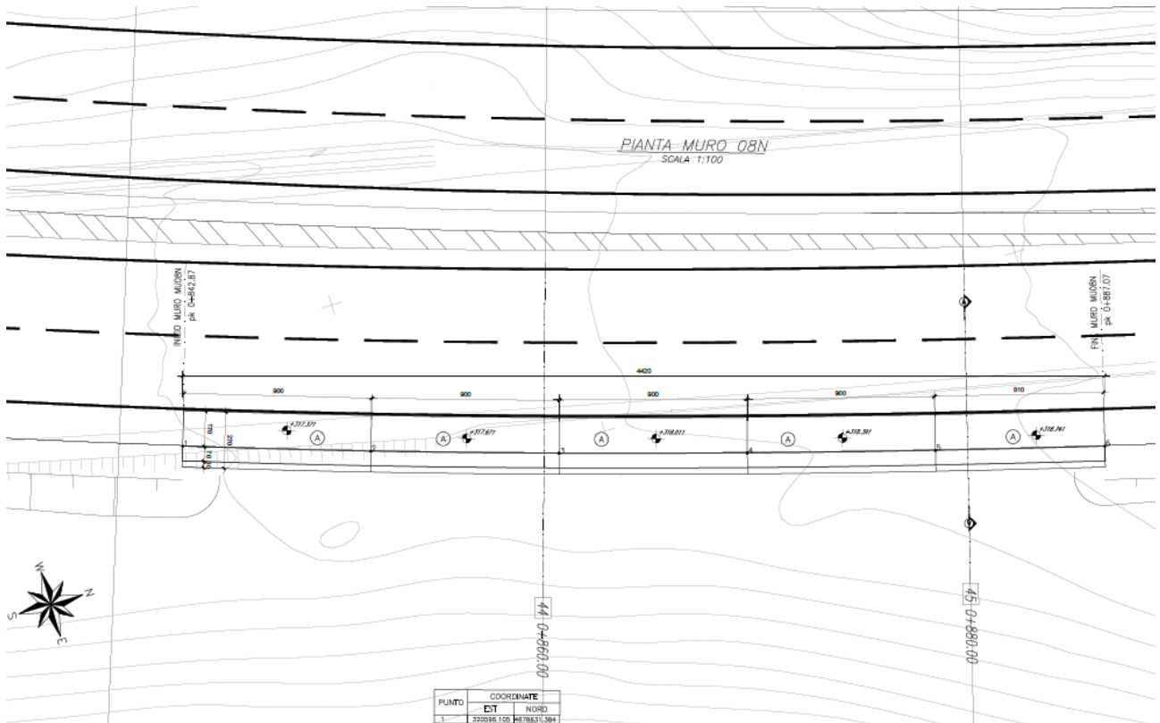
Figura 3: planimetria di progetto
