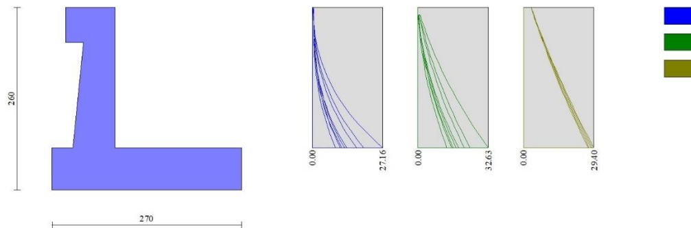
Fig. 8 - Paramento (Inviluppo)
