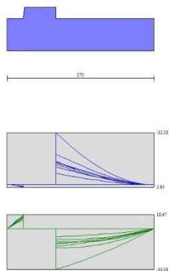
Fig. 18 - Fondazione
