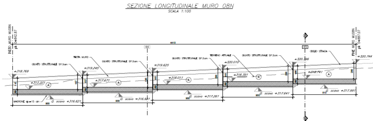
Figura 2: profilo longitudinale muro di sostegno
