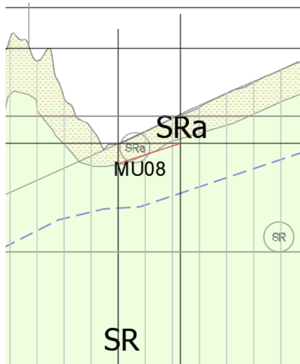
Figura 5: Stralcio profilo geotecnico con ubicazione dell'opera
