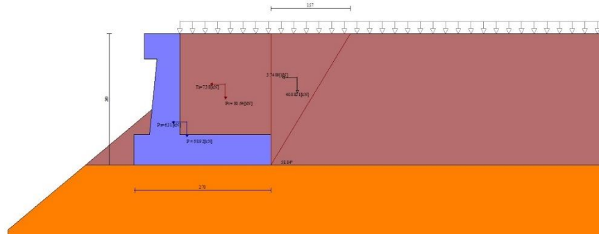
Fig. 13 - Cuneo di spinta (combinazione sismica) (Combinazione n° 2)
