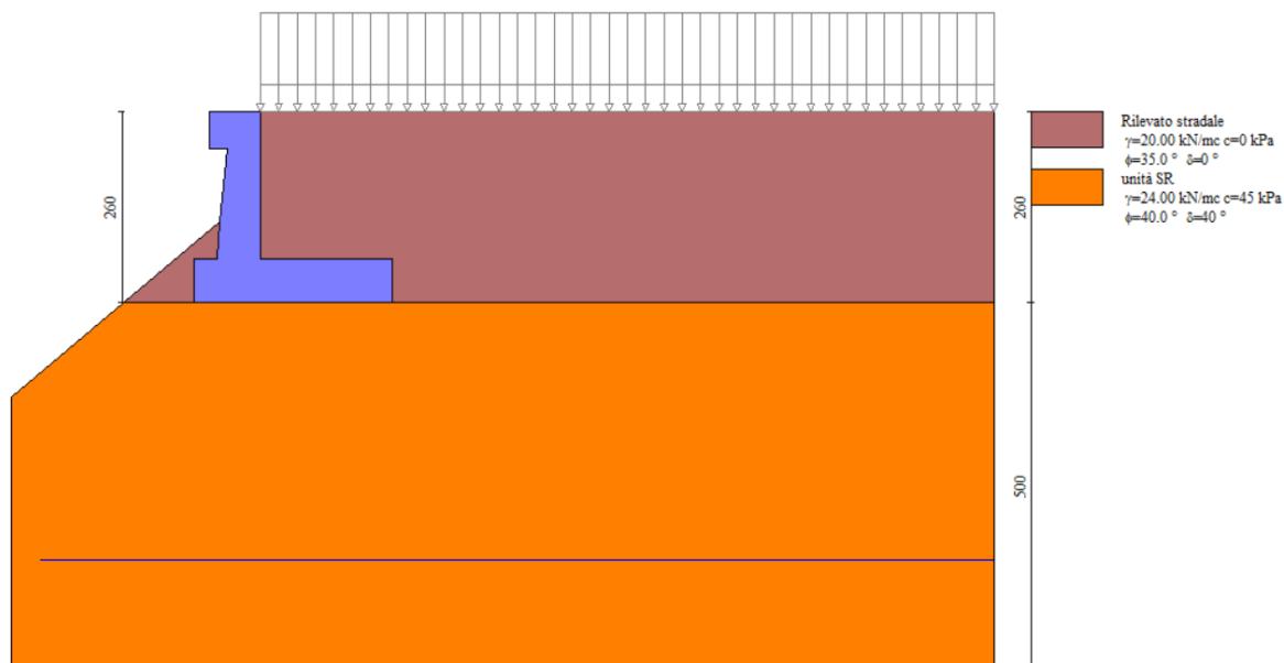
Figura 14: modello di calcolo muro tipologico A
