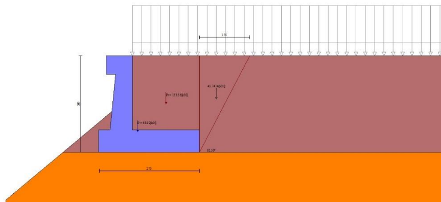
Fig. 11 - Cuneo di spinta (combinazione statica) (Combinazione n° 1)
