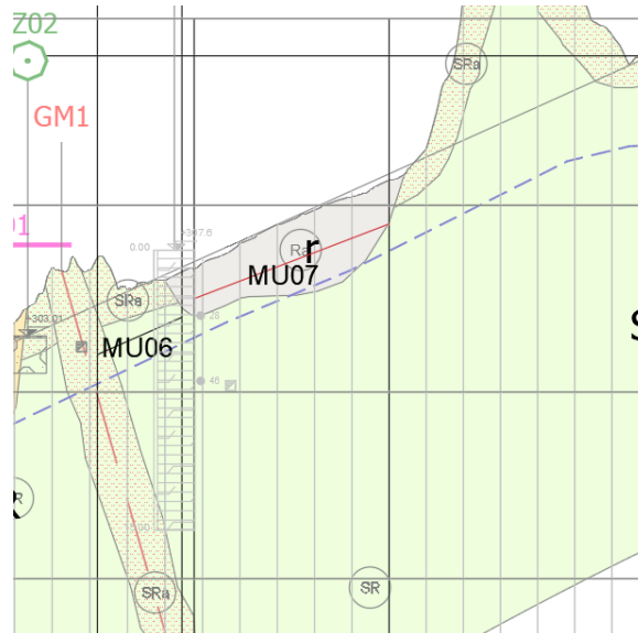
Figura 5: Stralcio profilo geotecnico con ubicazione dell'opera
