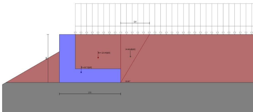
Fig. 10 - Cuneo di spinta (combinazione statica) (Combinazione n° 1)
