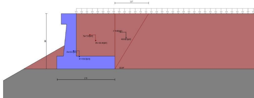
Fig. 13 - Cuneo di spinta (combinazione sismica) (Combinazione n° 2)
