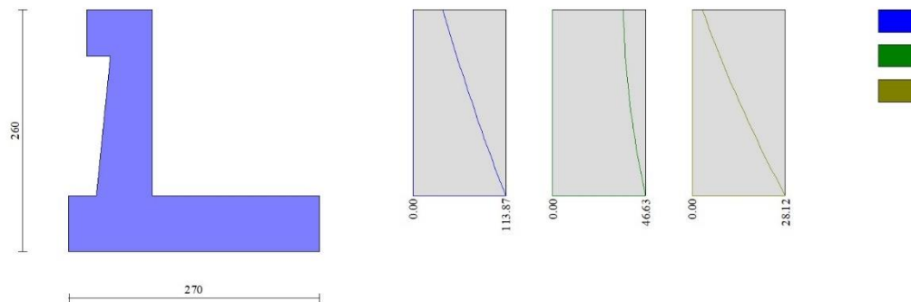
Fig. 12 - Paramento
