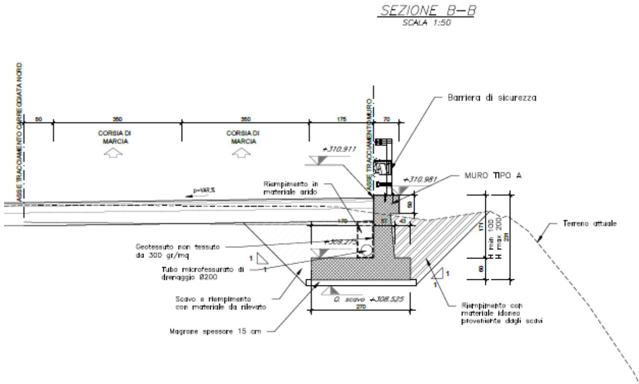
Figura 4: sezione trasversale muro tipologico A
