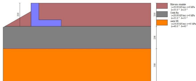
Fig. 2 - Stratigrafia
