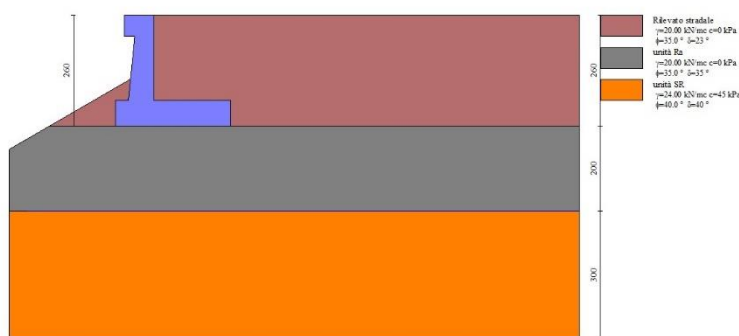
Fig. 2 - Stratigrafia
