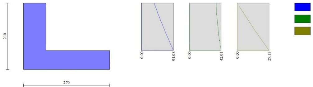
Fig. 6 - Paramento (Inviluppo)
