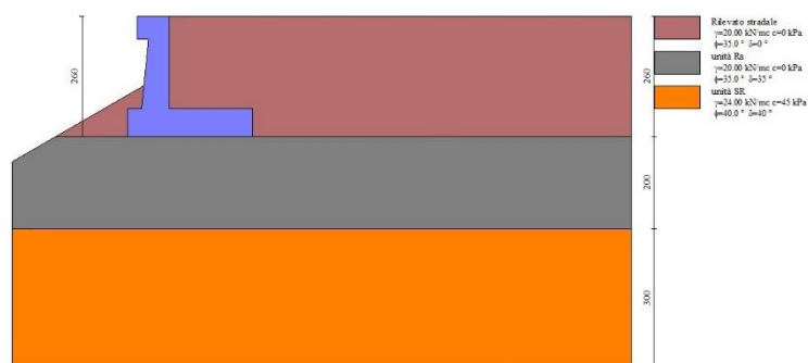
Fig. 2 - Stratigrafia
