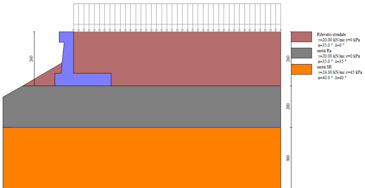
Figura 23: modello di calcolo muro tipologico A
