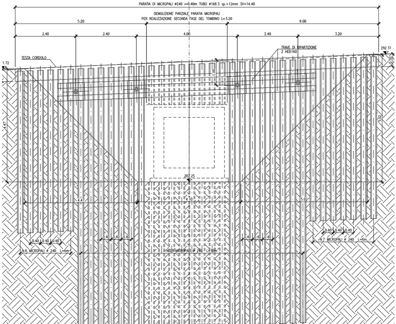
Fig. 2- prospetto fase realizzazione tombino
