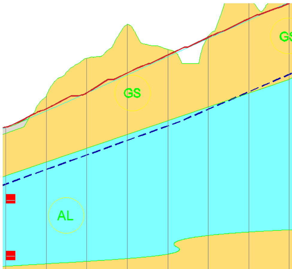
Fig. 3 stratigrafia di progetto
