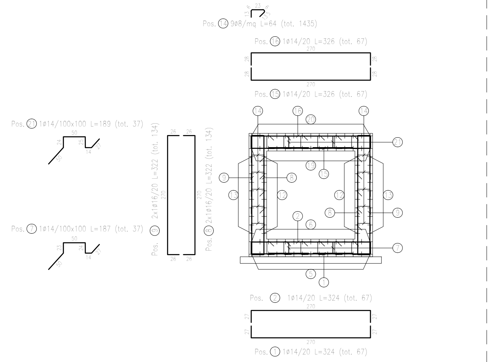
STRALCIO Pianta COPERTURA - Scala 1:50 -
