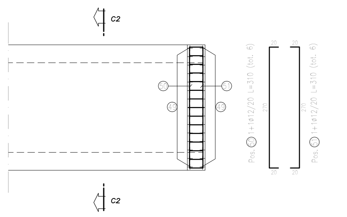
STRALCIO Pianta COPERTURA - Scala 1:50 -
