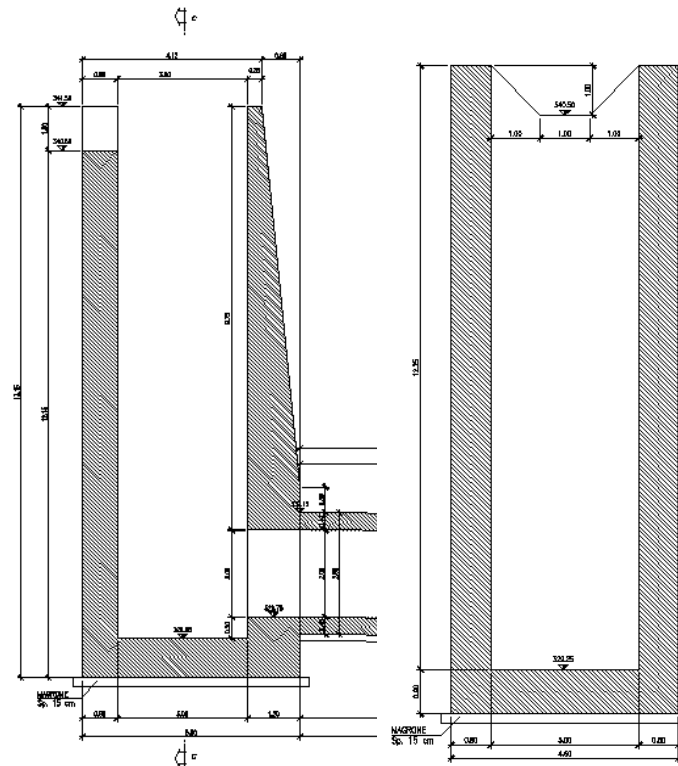
Figura 3- sezioni pozzetto
