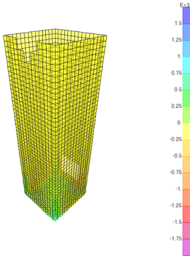
Figura 20 - involuopo azioni assiali F22 sle rara
