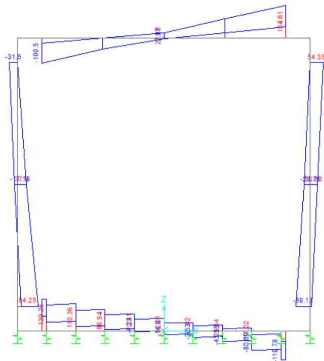
Figura 31– Involuppo sforzi taglienti SLU-SLV
