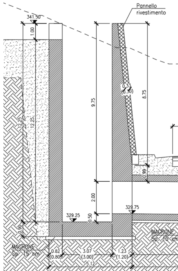
Figura 6 – sezione longitudinale
