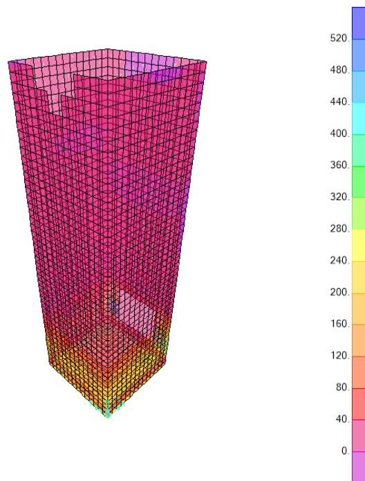
Figura 13– Involuppo momenti flettenti M_{22} SLU-SLV
