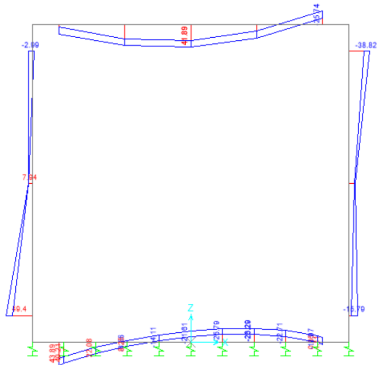
Figura 33- Involuppo momenti flettenti SLE rara
