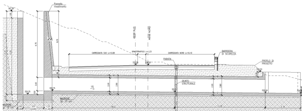
Figura 1- Profilo longitudinale
