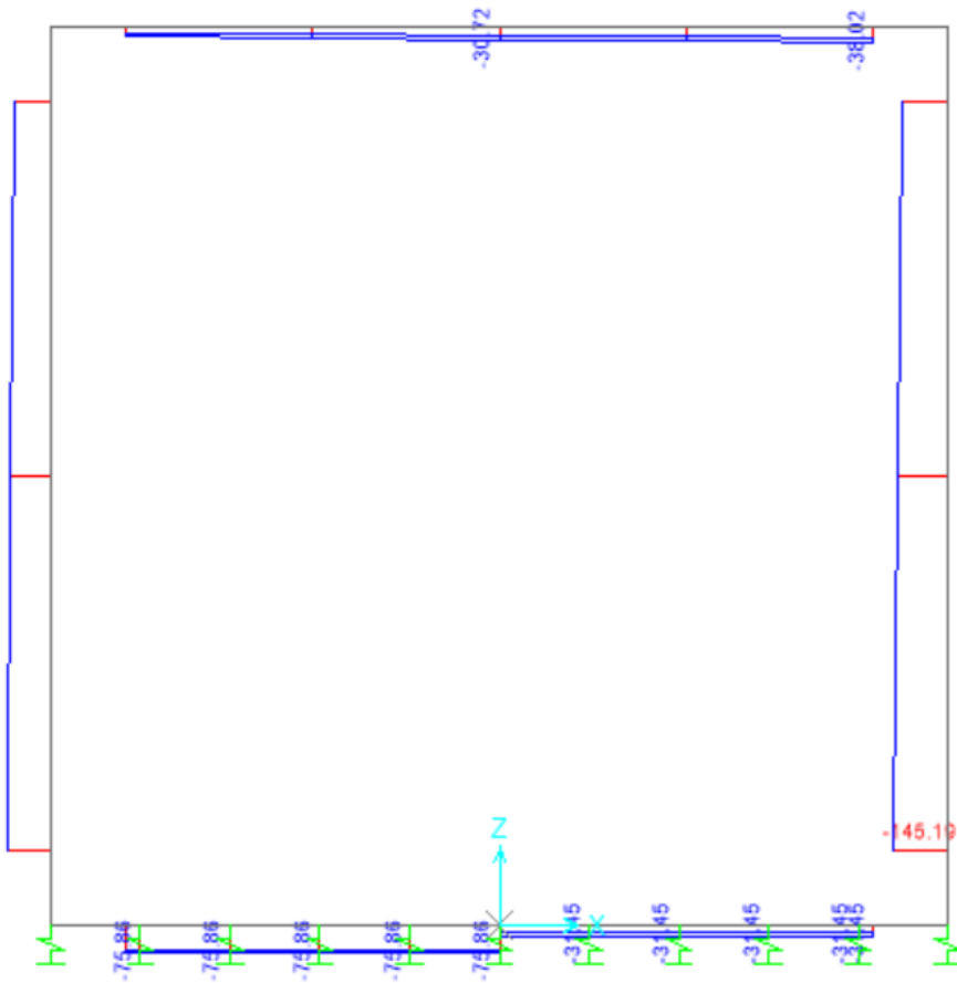
Figura 34– Involuppo azioni assiali SLE rara
