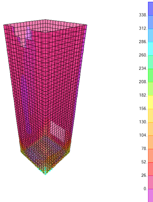
Figura 12 – Involuppo momenti flettenti M_{11} SLU-SLV
