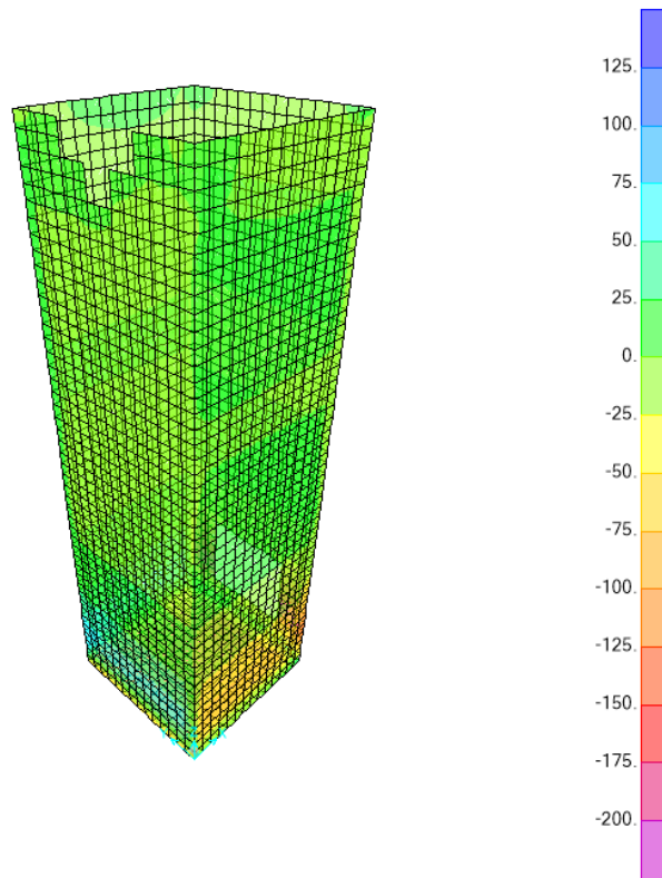
Figura 18– Involuppo momenti flettenti M22 SLE rara
