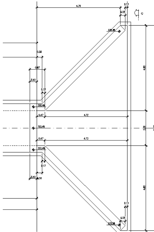
Figura 4- pianta muro
