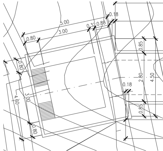
Figura 7 – pianta
