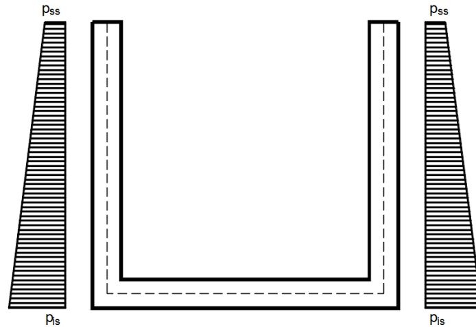
Figura 38 – Schema tipo spinta terreno su pareti
