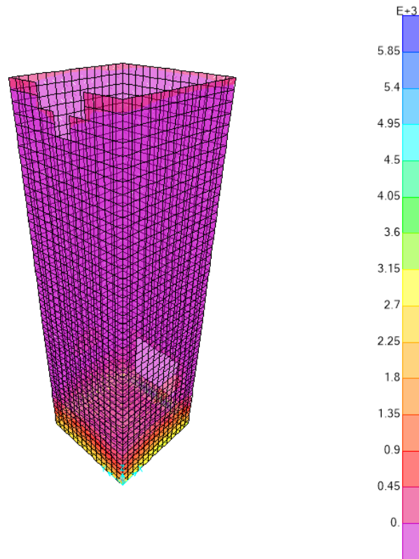
Figura 16– Involuppo azioni assiali F11 SLU-SLV
