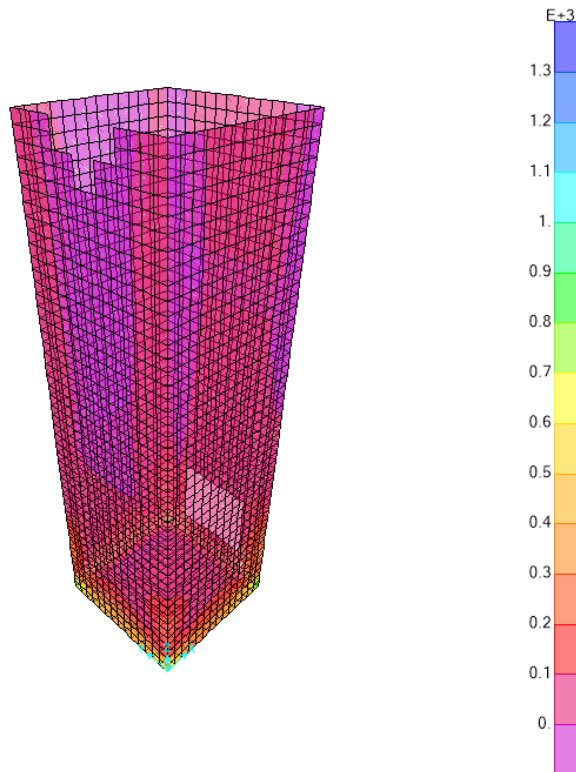
Figura 15 - Inviluppo sforzi taglienti V23 SLU-SLV
