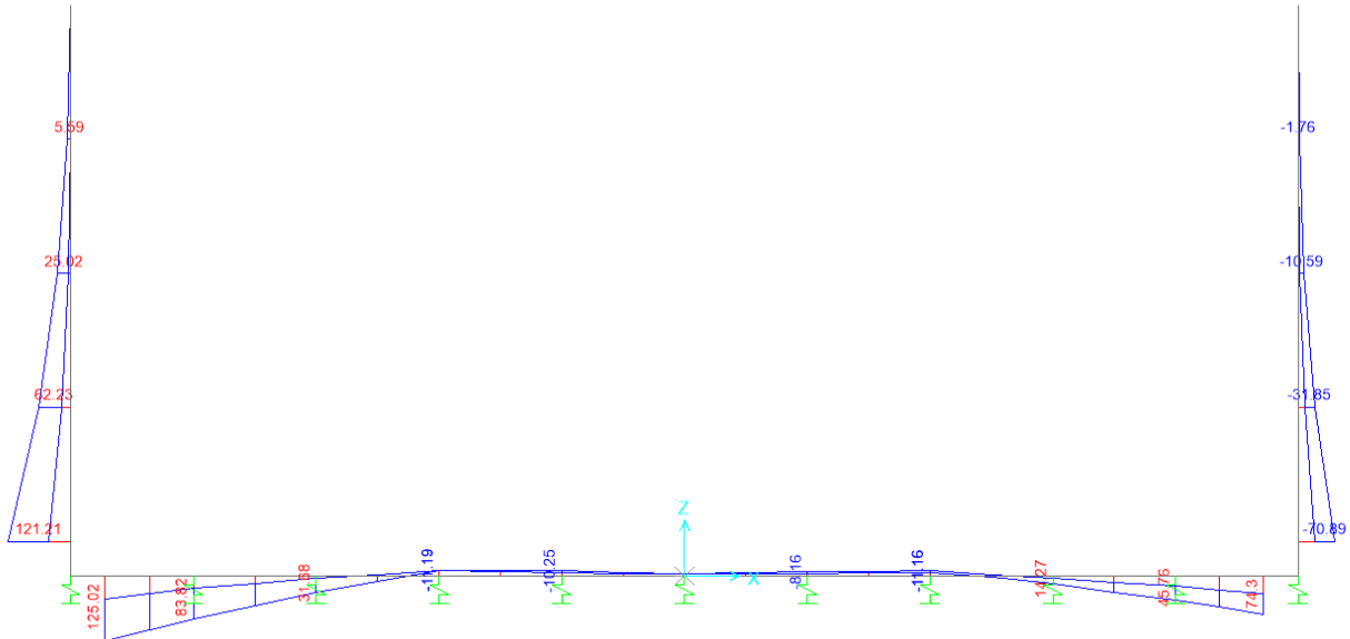
Figura 42– Involuppo momenti flettenti SLU-SLV
