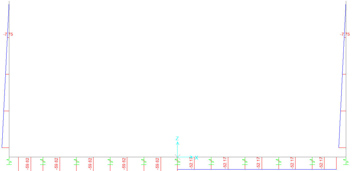
Figura 46– Involuppo azioni assiali SLE rara
