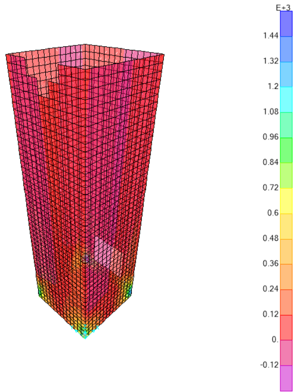
Figura 14 Inviluppo sforzi taglienti V13 SLU-SLV
