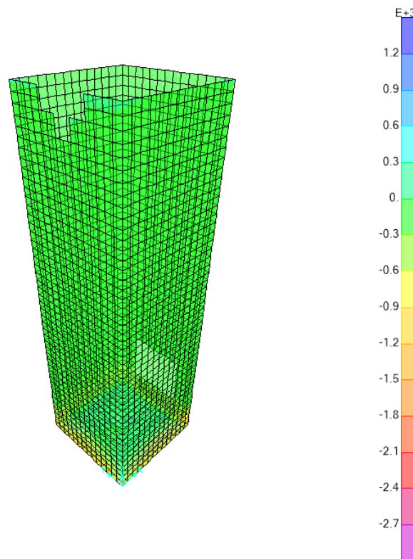
Figura 19 – involuppo azioni assiali F11 sle rara
