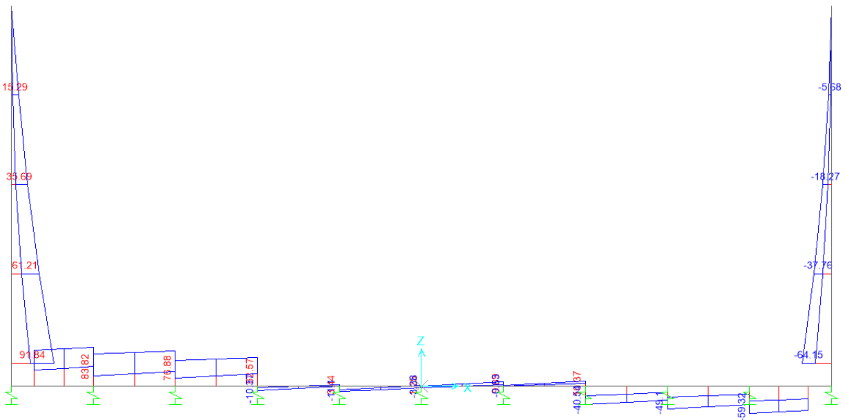
Figura 43– Involuppo sforzi taglianti SLU-SLV
