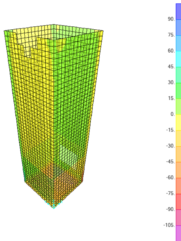
Figura 17– Involuppo momenti flettenti M11 SLE rara
