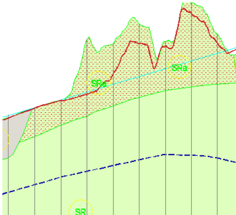
Figura 5 - stratigrafia di progetto
