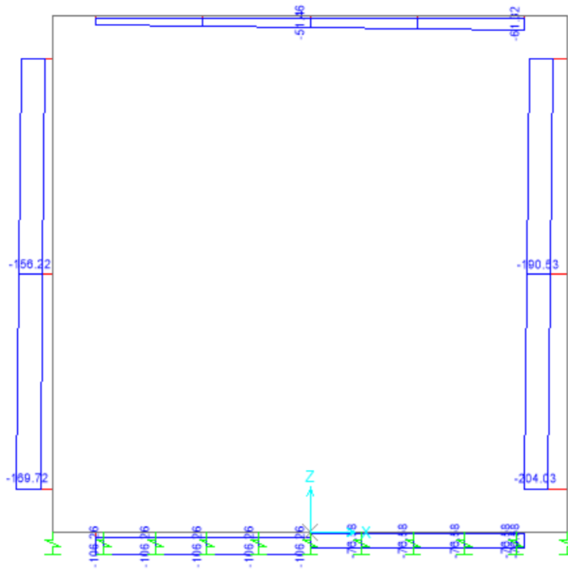
Figura 32- Involuppo azioni assiali SLU-SLV
