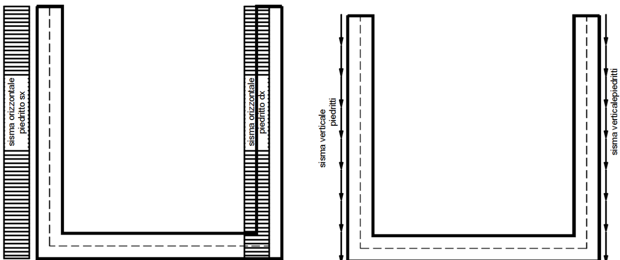
Figura 41– Schema tipo azioni sismiche orizzontali e verticali
