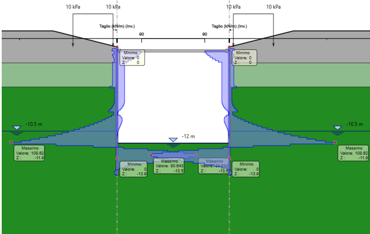
Figura 46: Involuppo Taglio Condizioni Statiche
