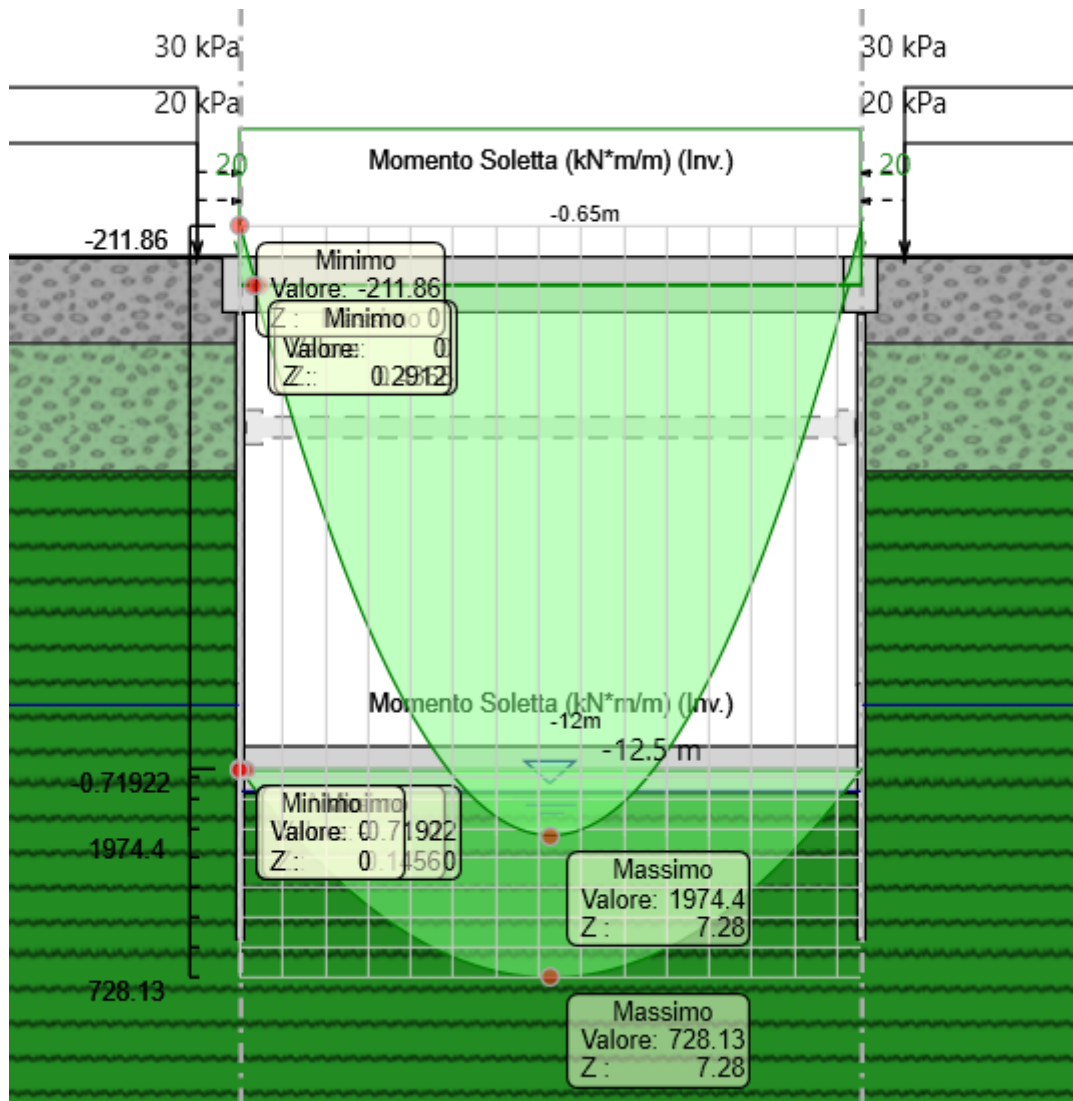
Figura 38: Involuppo momento sollecitante solettone SLE [kNm/m]
