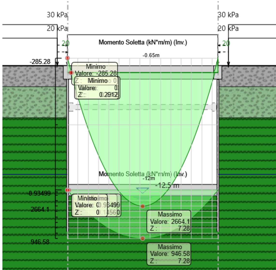
Figura 37: Involuppo momento sollecitante solettone SLU [kNm/m]
