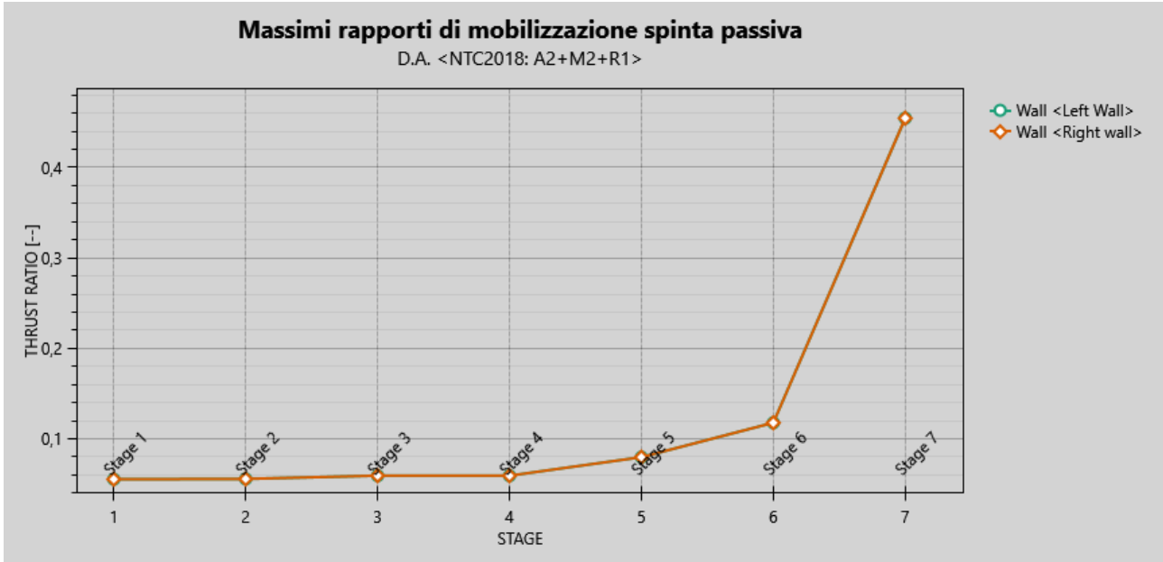
Figura 47: Massimi rapporti di mobilitazione della spinta passiva combinazione A2+M2+R1
