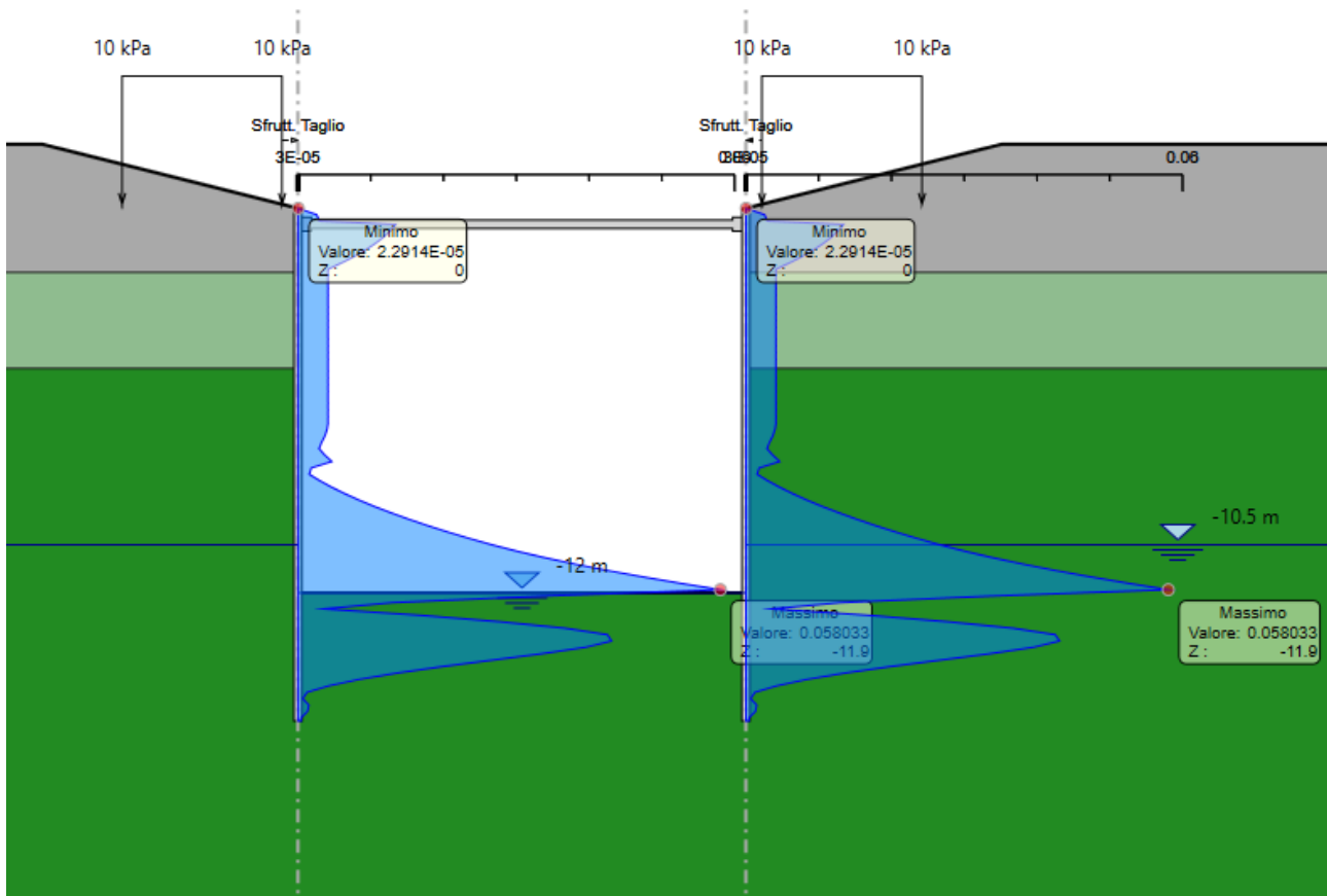
Figura 49: Involuppo coefficiente di sfruttamento a taglio.
