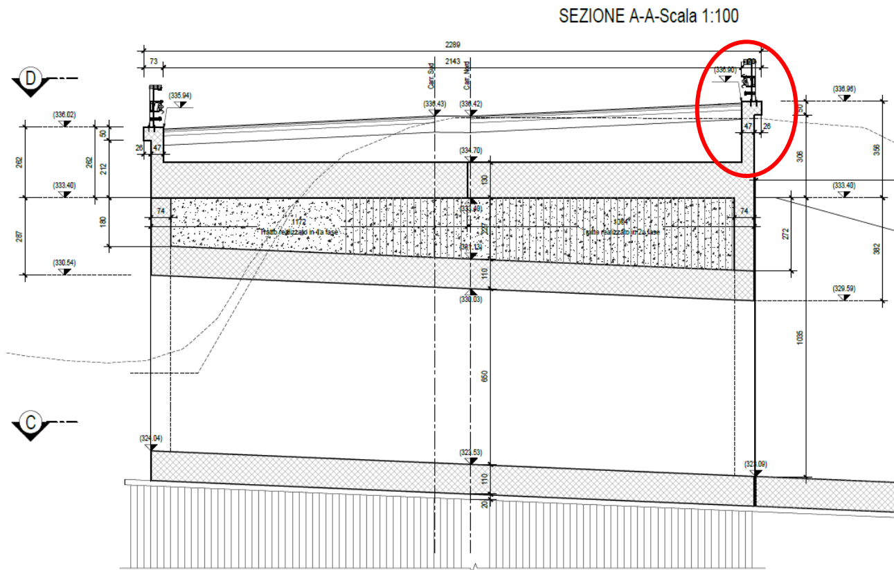
Figura 51: Sezione A-A con indicazione del muro strada.
