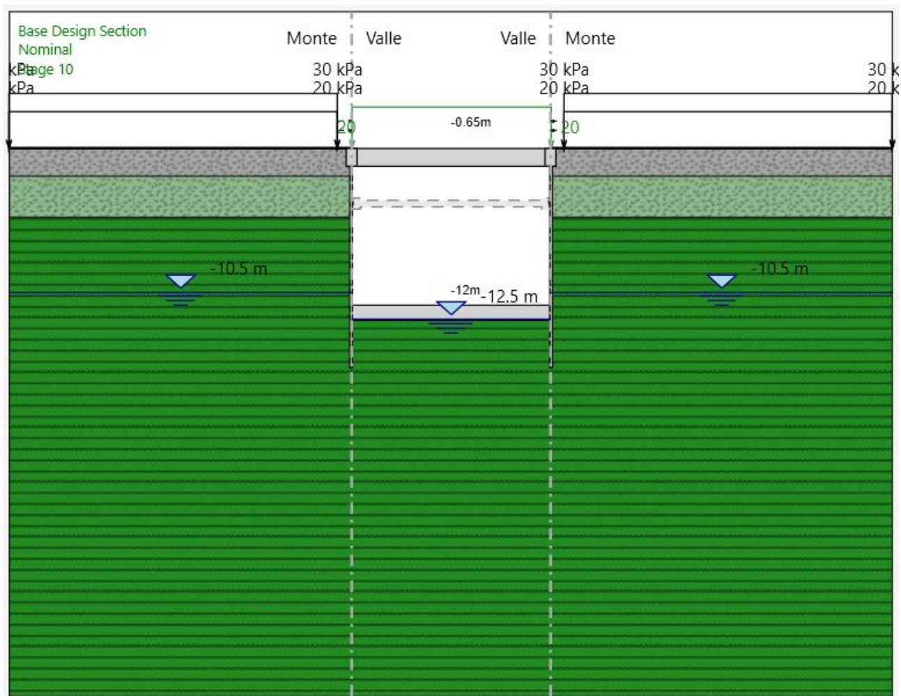
Figura 24 – Modello Paratia (Fase finale)
