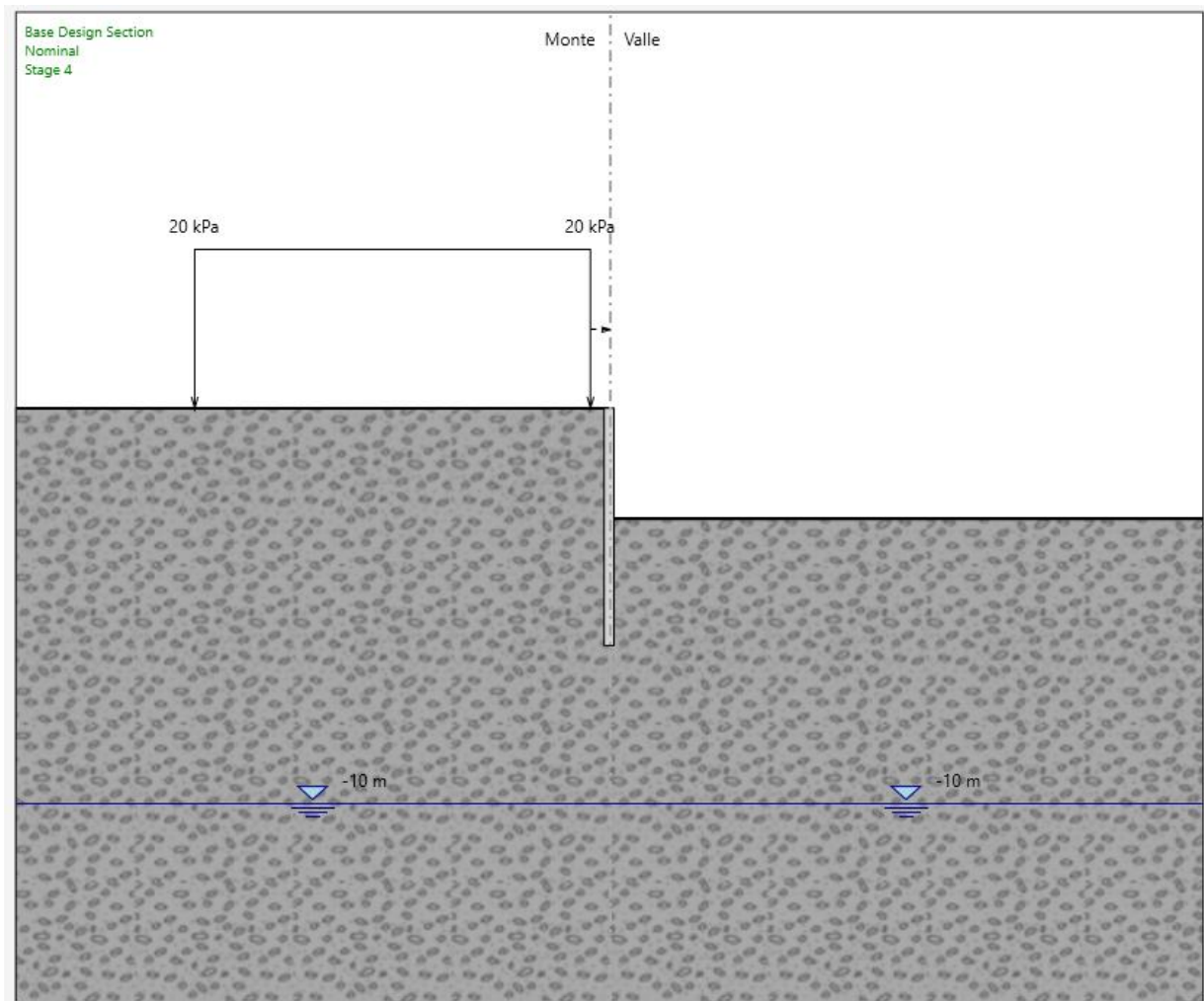
Figura 7 – Modello Paratia (Fase finale)
