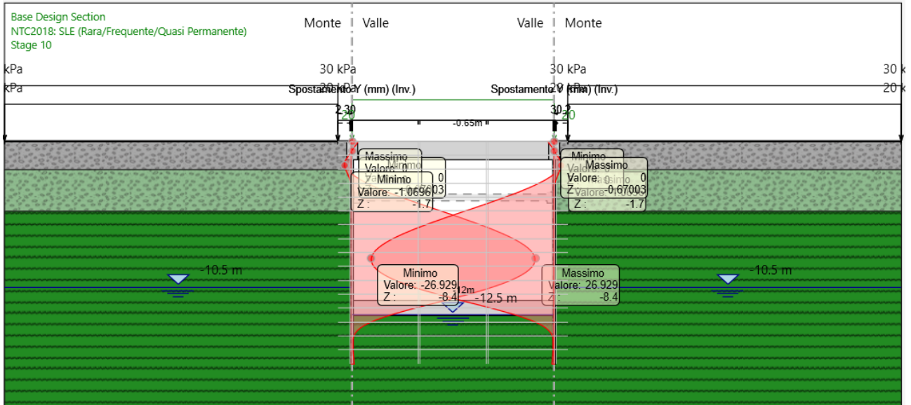
Figura 32: Spostamenti paratia allo SLE (mm)- max 26.93 mm
