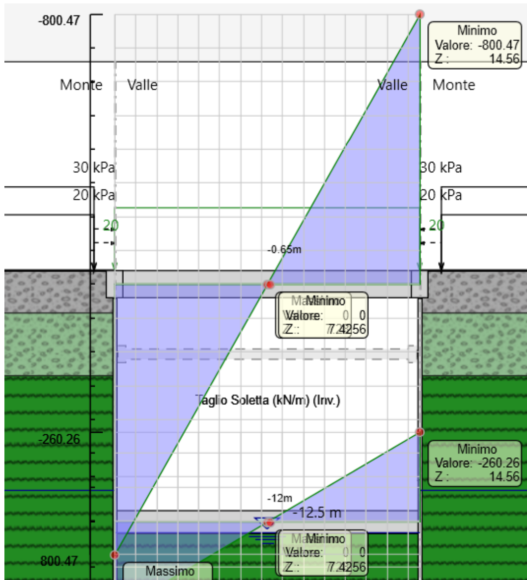
Figura 39: Inviluppo Taglio sollecitante solettone SLU [kN/m]
