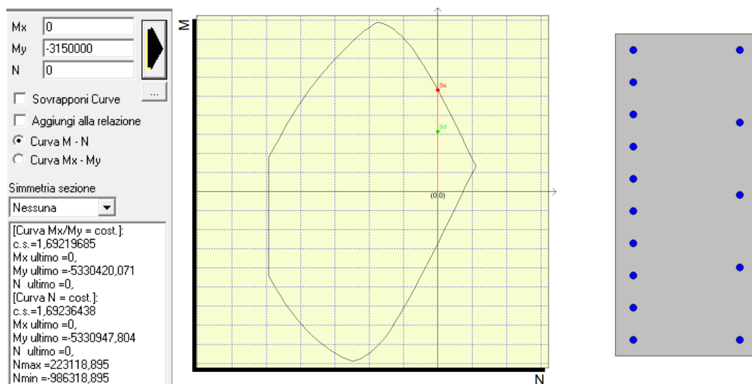
Figura 57: Verifica a flessione Muro – FS=1,69
