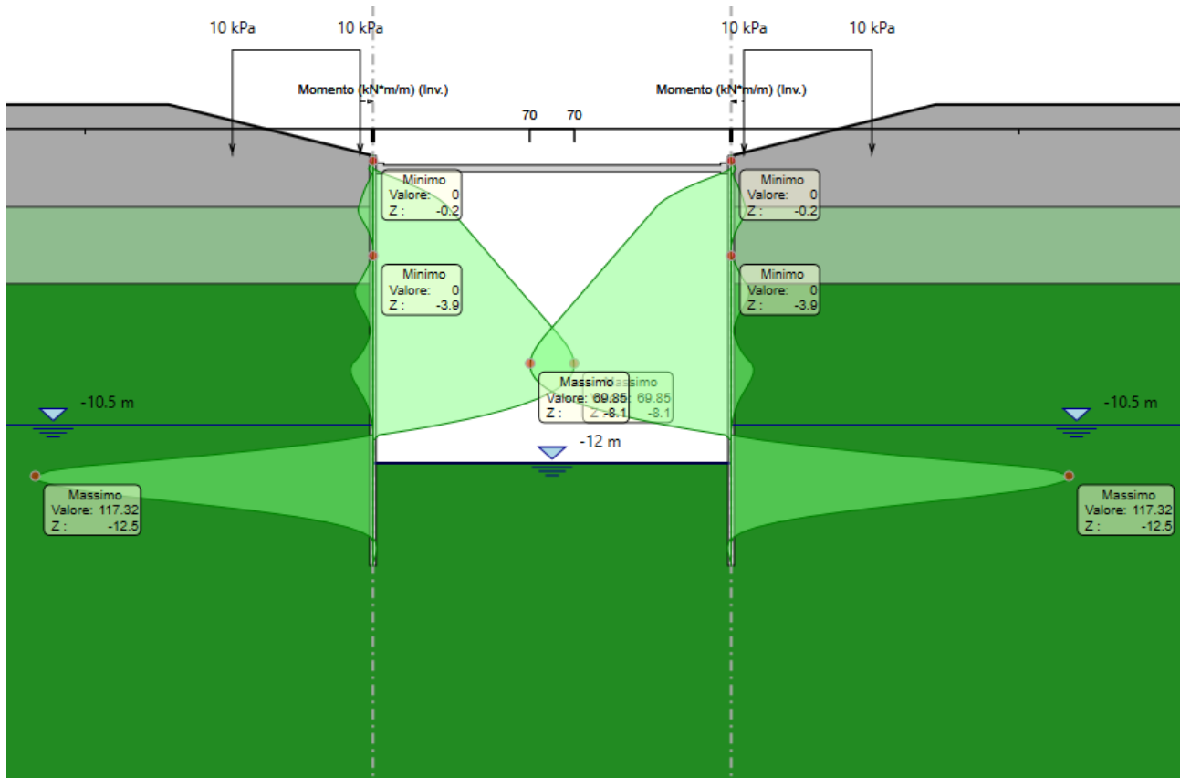
Figura 45: Involucro Momento Flettente Condizioni Statiche
