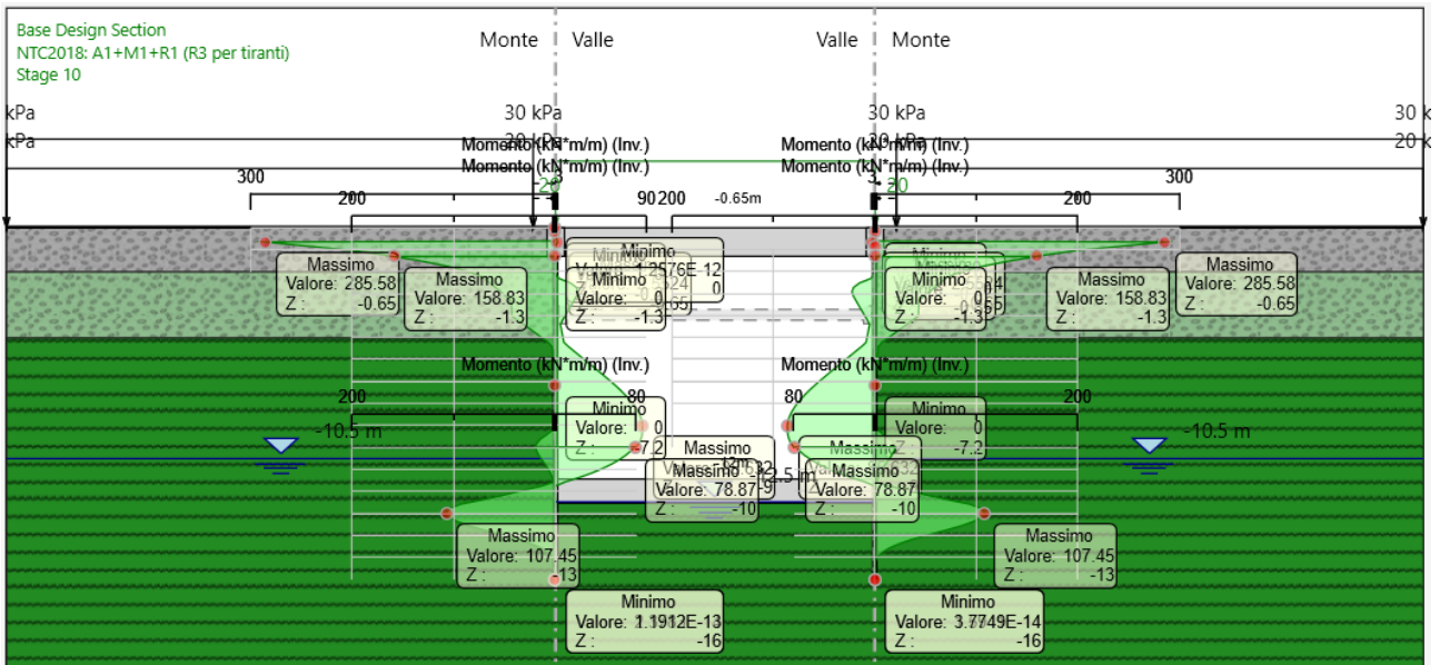
Figura 33: Involuppo momento sollecitante paratia SLU [kNm/m]
