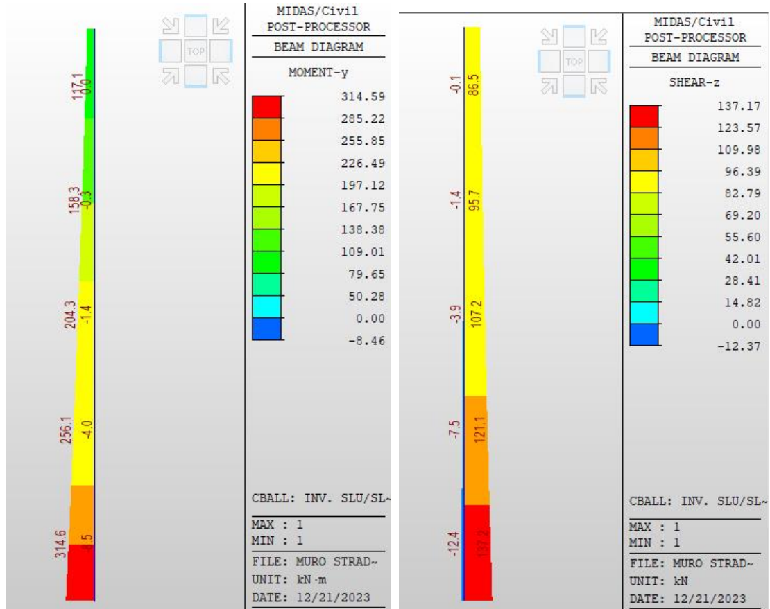
Figura 55: Momento flettente e Taglio (Involuppo SLU/SLV)
