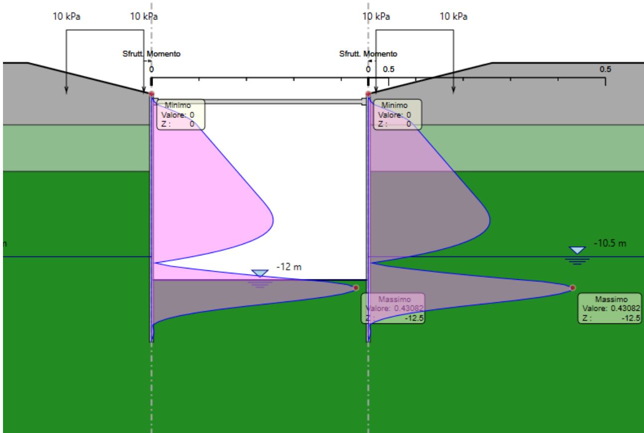
Figura 48: Inviluppo coefficiente di sfruttamento a flessione.
