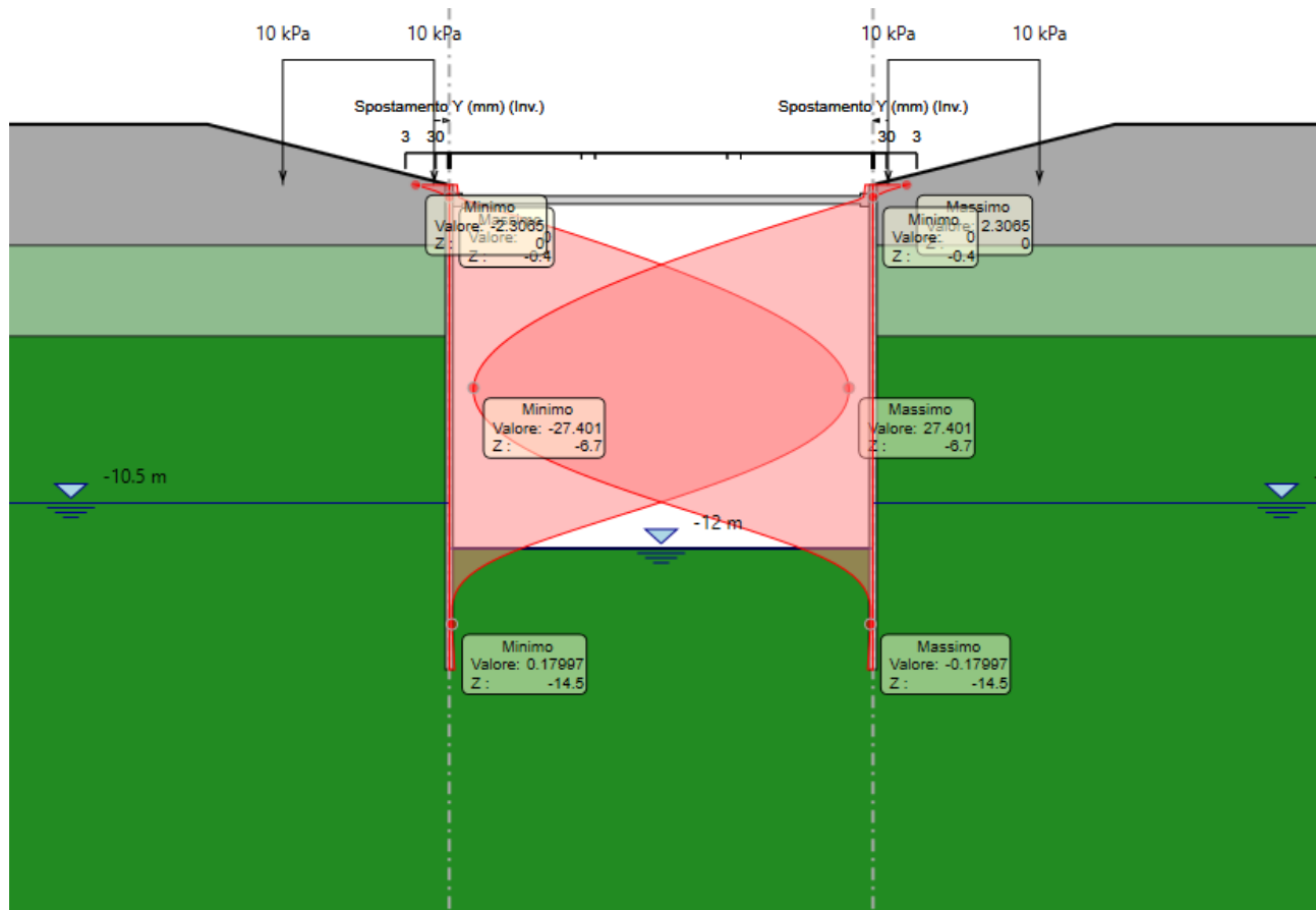
Figura 44: Involuppo Spostamenti SLE
