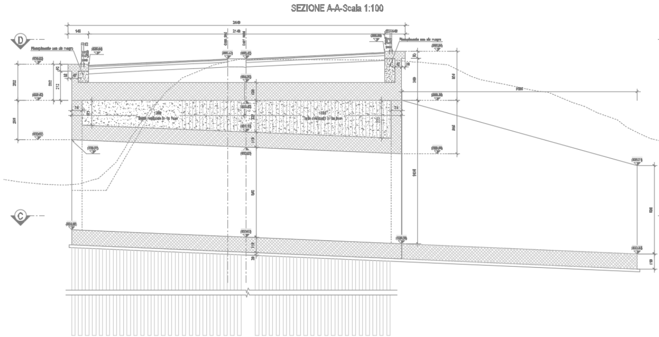
Figura 3 – Sezione Longitudinale TM10
