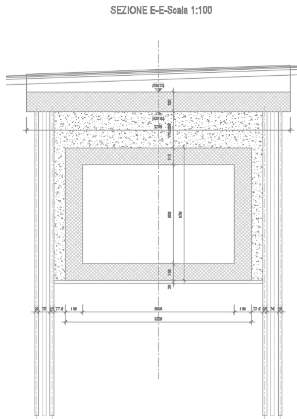
Figura 4 – Sezione Trasversale TM10
