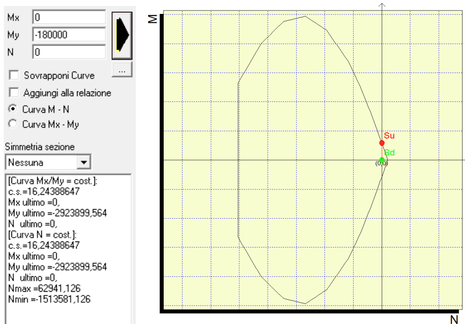
Figura 50 – Verifica a Flessione FS=16 - SLU
