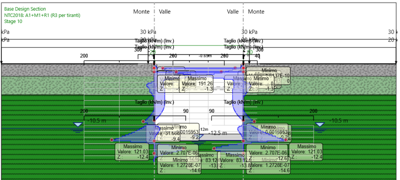
Figura 34: Involuppo Taglio sollecitante paratia SLU [kN/m]
