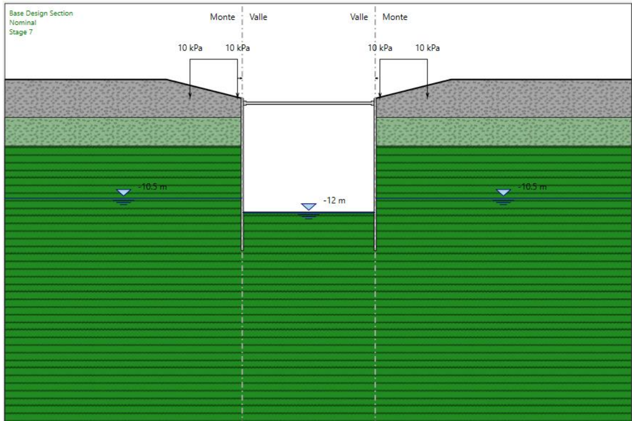
Figura 42 – Modello Paratia (Fase finale)
