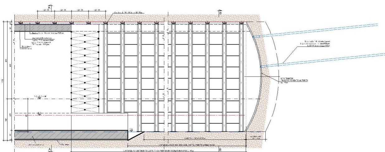
Sezione tipo B1 – Interventi – Sezione longitudinale
