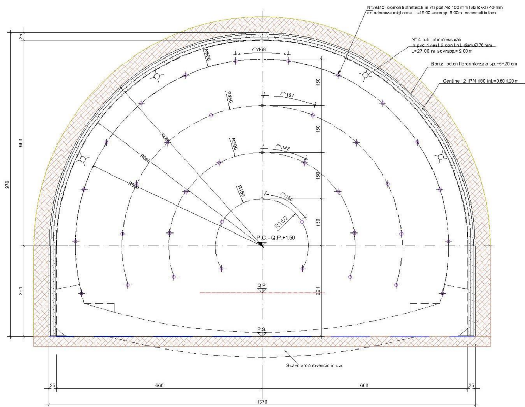
Sezione tipo B1b – Interventi – Sezione trasversale
