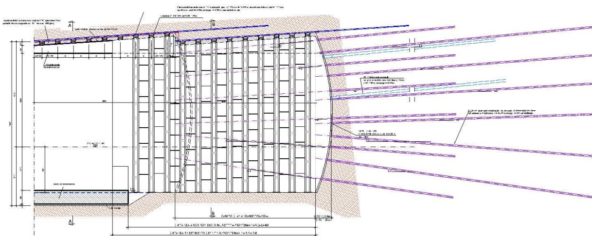
Sezione tipo B2b – Interventi – Sezione longitudinale
