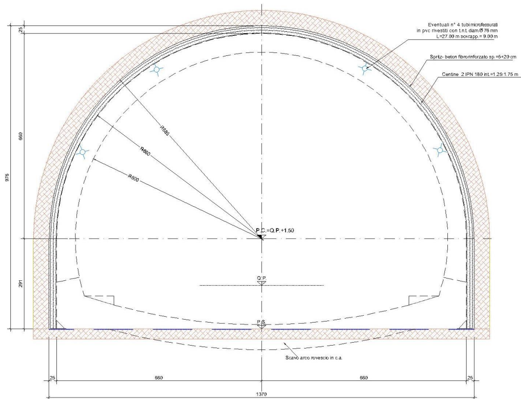
Sezione tipo B1 – Interventi – Sezione trasversale
