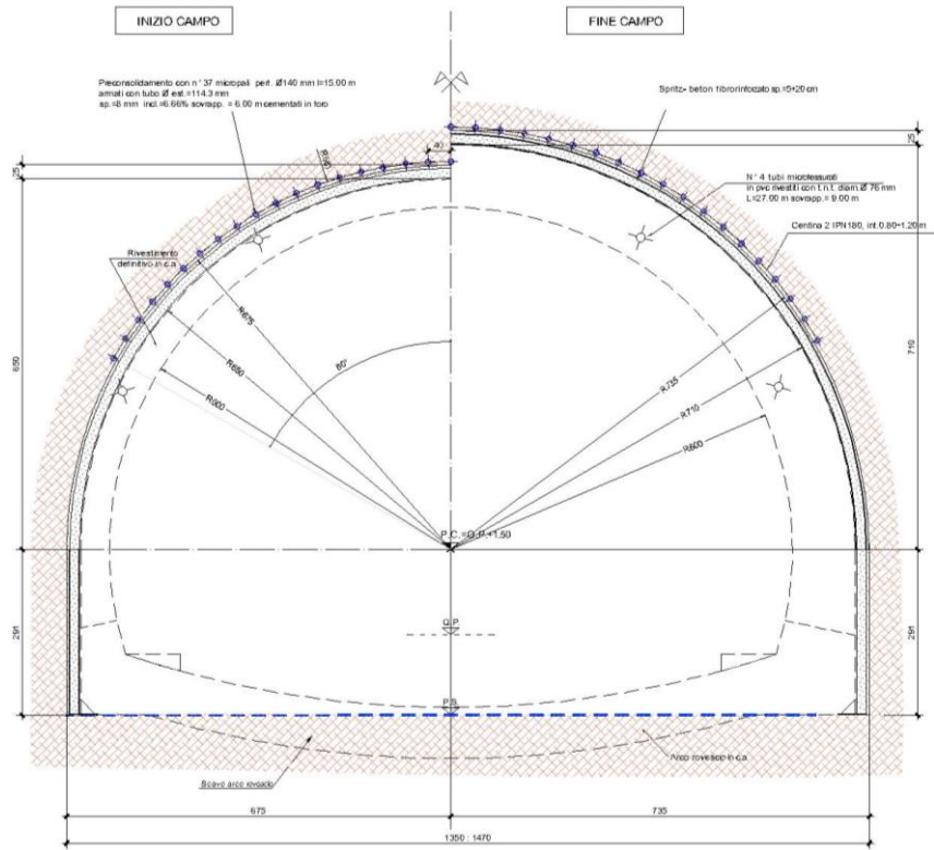
Sezione tipo B2 – Interventi – Sezione trasversale
