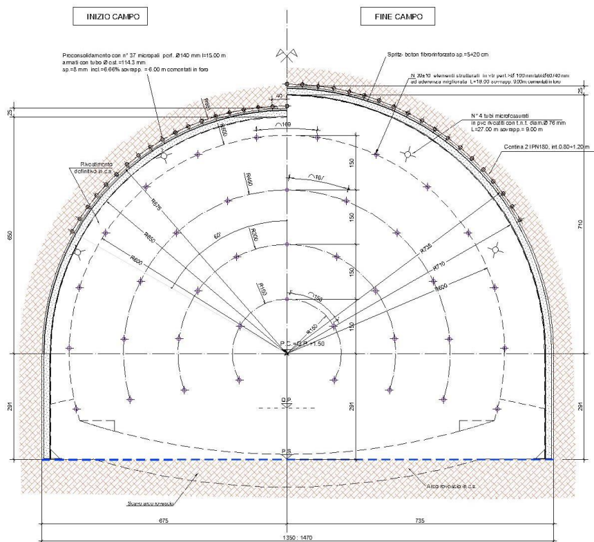
Sezione tipo B2b – Interventi – Sezione trasversale
