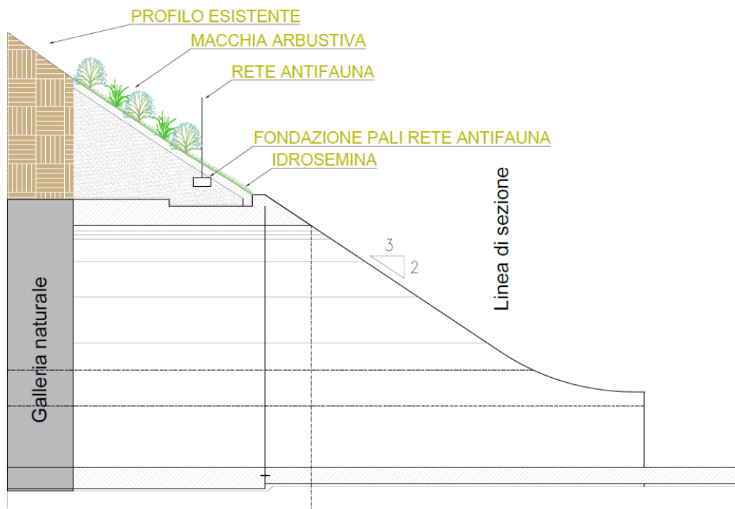
Sezione longitudinale e frontale, scala 1:100
