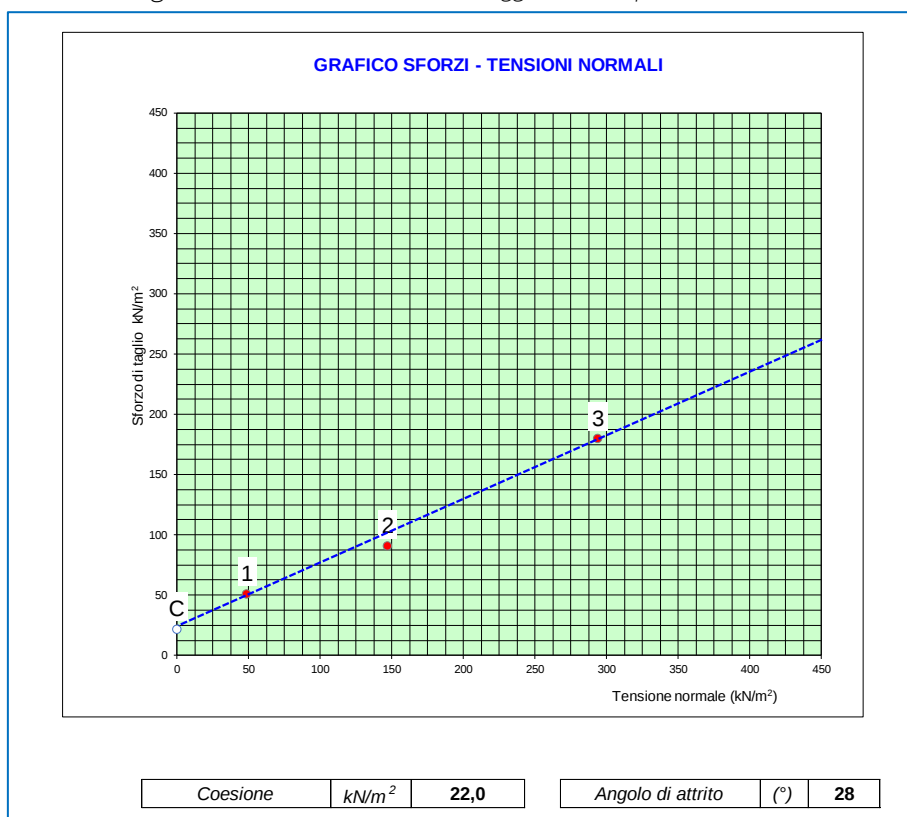
Figura 10.3 – Prova di TD - Sondaggio S.3 Campione C1 (m 2,00 – 2,50)
