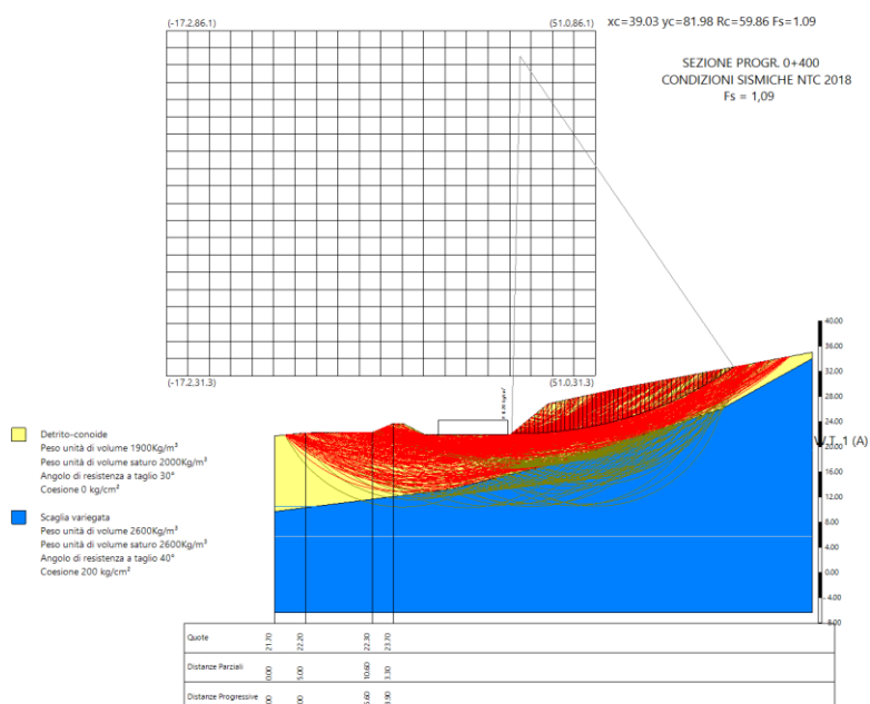
Figura 11.20 – Verifica sismica Progr. 0+400
