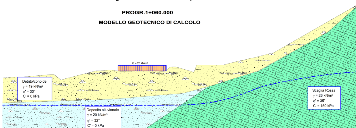
Figura 11.22 – Modello geotecnico di calcolo
