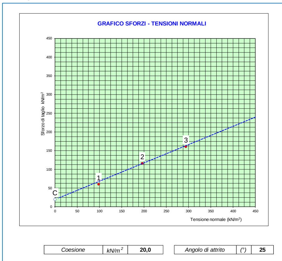
Figura 10.1 – Prova di TD - Sondaggio S.1 Campione CR1 (m 11,20 – 11,70)
