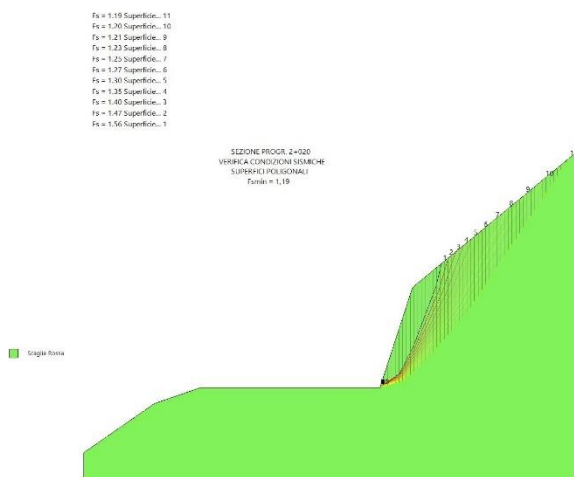
Figura 11.25 – Progressiva Km 2+020 – Verifica con Hoeck & Bray
