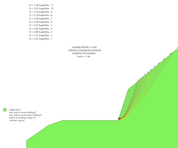
Figura 11.26 – Progressiva Km 2+020 – Verifica con Bishop
