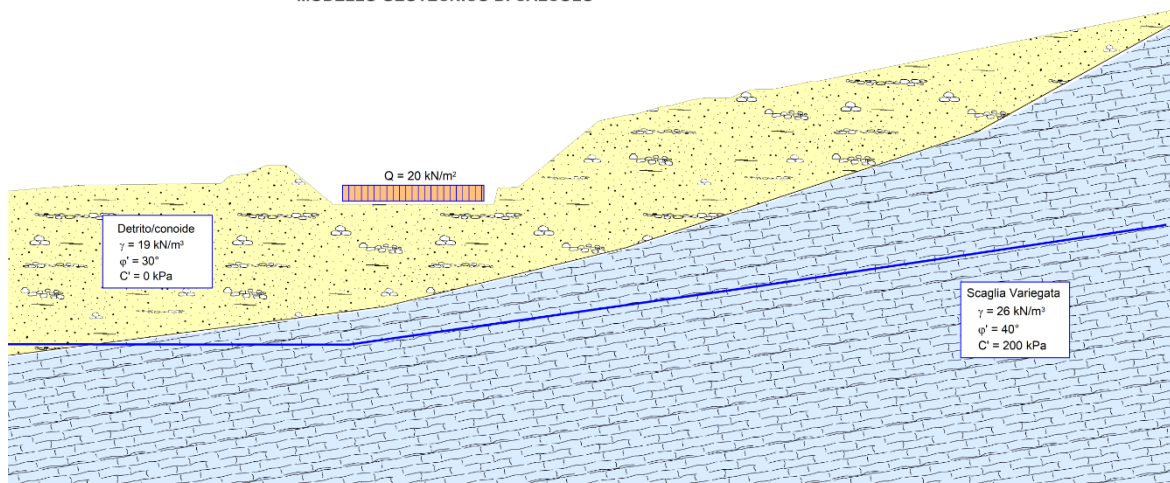
Figura 11.19 – Modello geotecnico di calcolo
