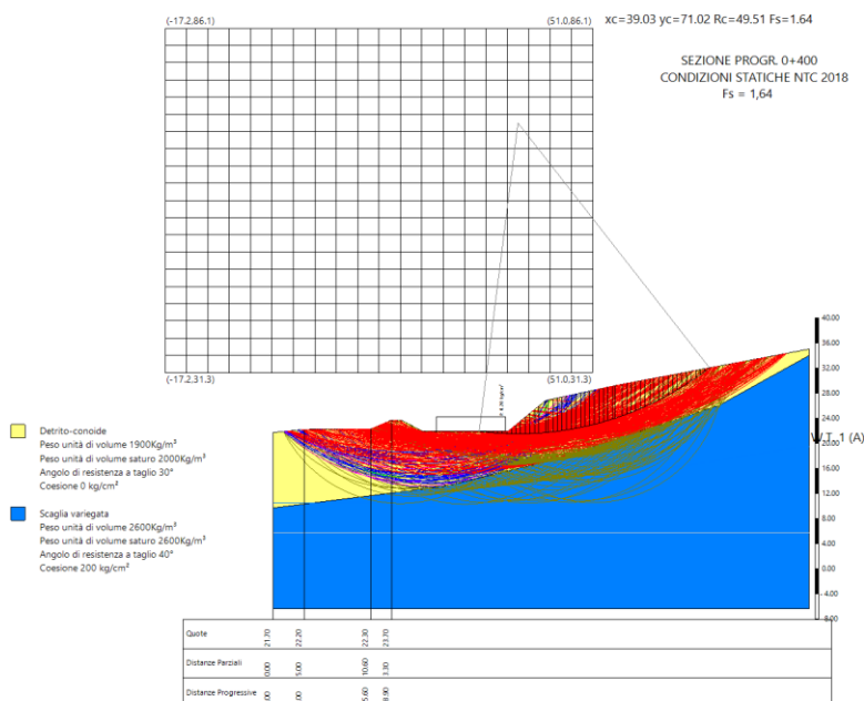
Figura 11.21 – Verifica statica Progr. 0+400
