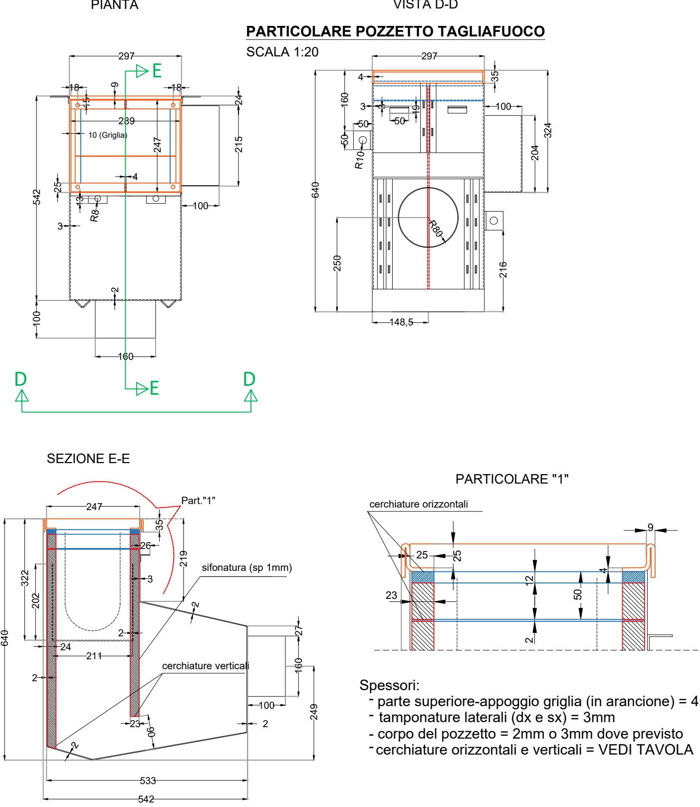
PARTICOLARE POZZETTO TAGLIAFUOCO SCALA 1:20
