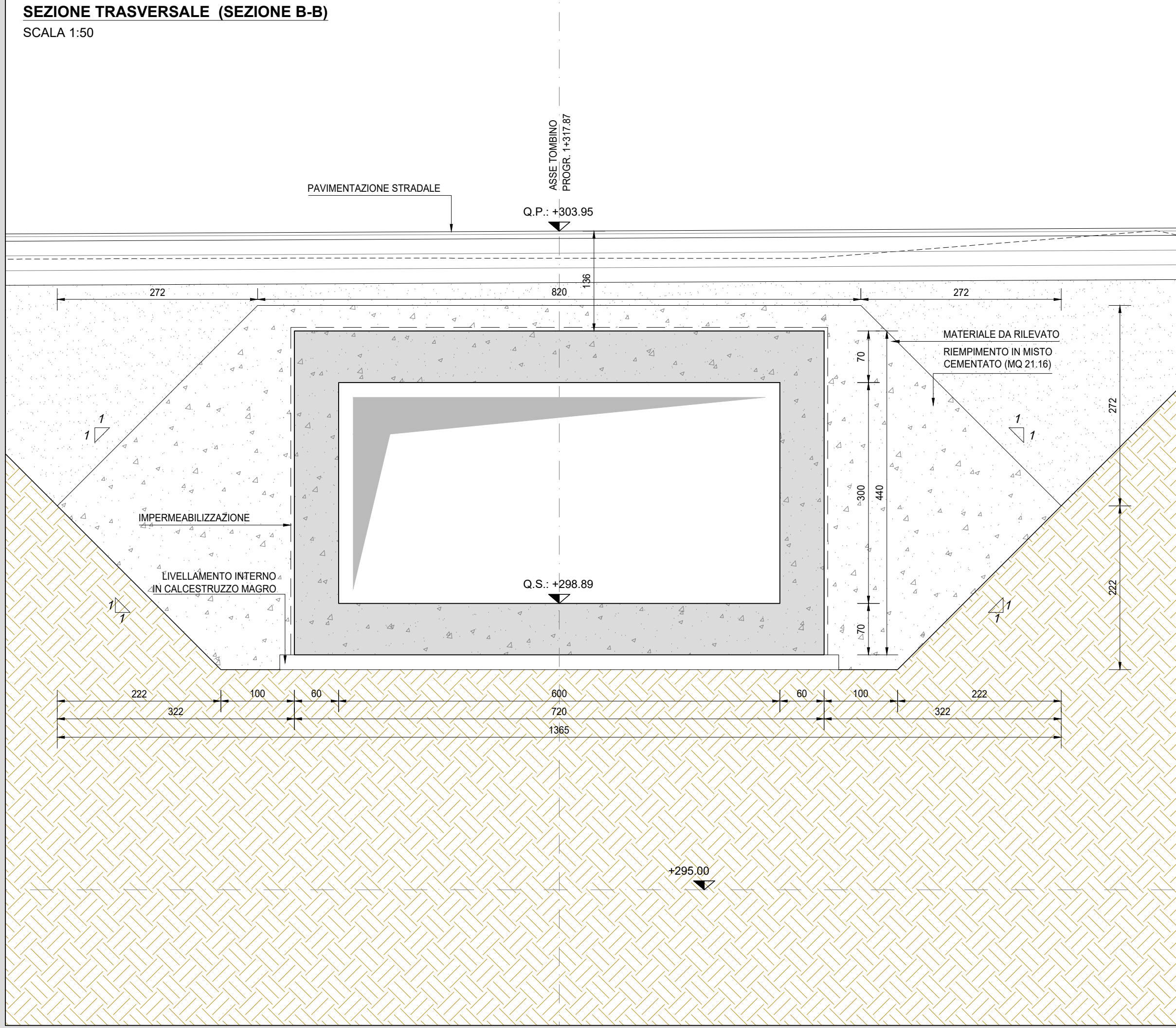
SEZIONE TRASVERSALE (SEZIONE B-B) SCALA 1:50
