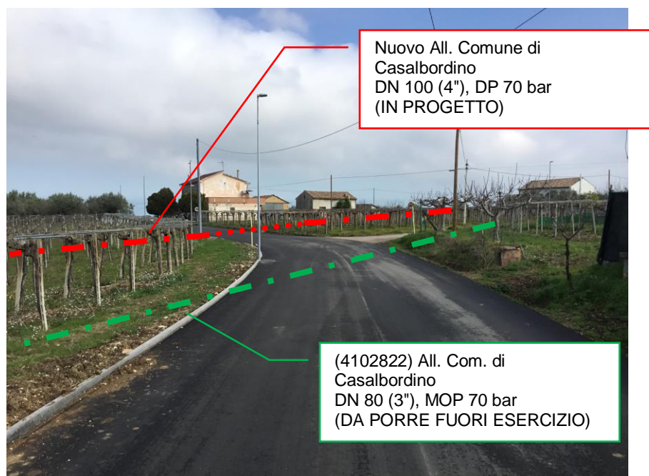
Foto n.4 – Vista metanodotto in progetto con attraversamento e metanodotto da porre fuori esercizio
