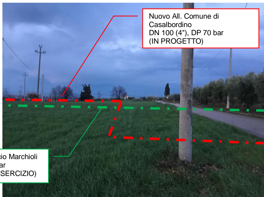
Foto n.2 – Vista metanodotto in progetto e metanodotto da porre fuori esercizio
