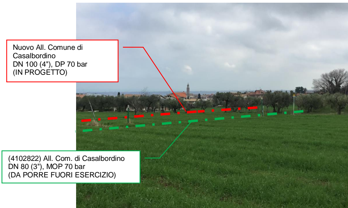
Foto n.6 – Panoramica metanodotto in progetto e metanodotto da porre fuori esercizio
