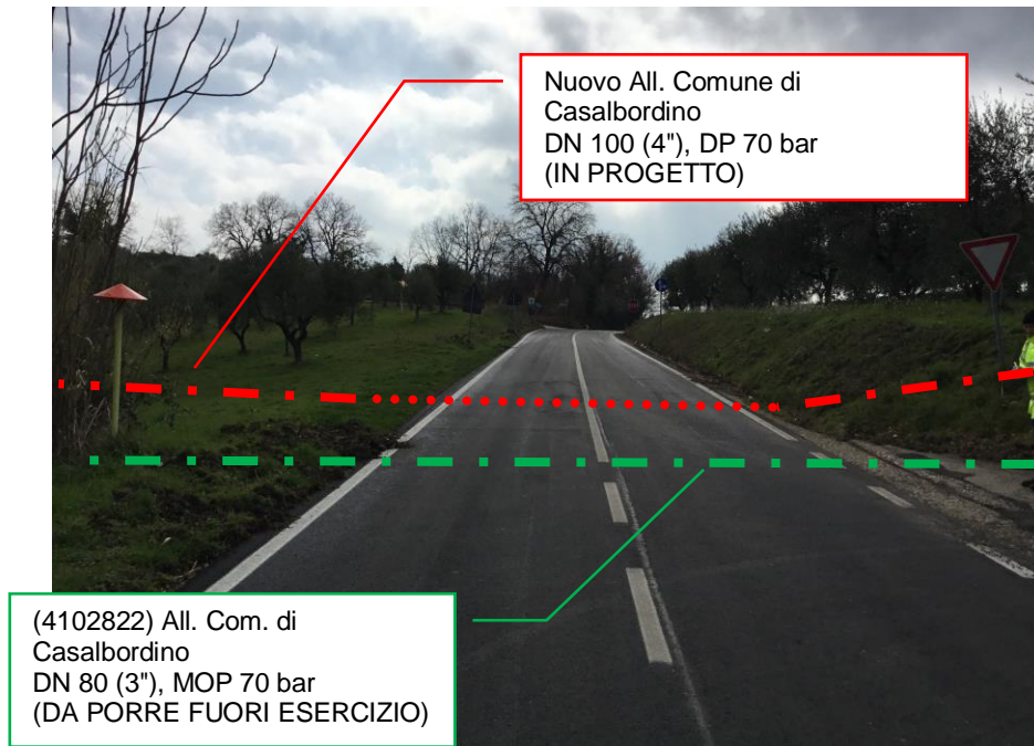
Foto n.5 – Vista metanodotto in progetto con attraversamento e metanodotto da porre fuori esercizio
