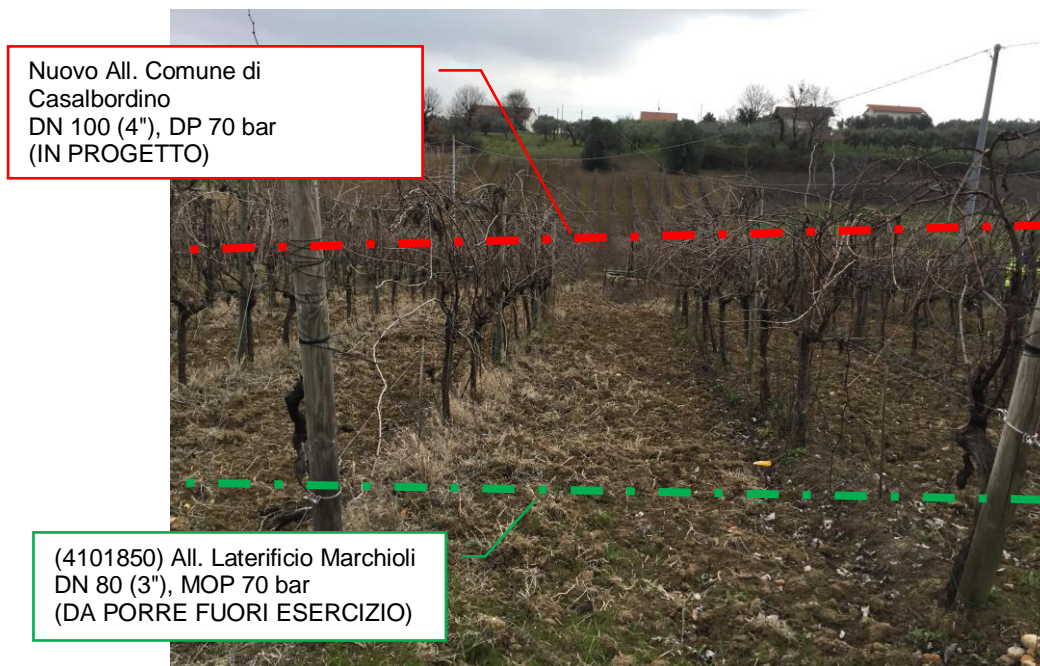
Foto n.3 – Panoramica metanodotti in progetto e metanodotto da porre fuori esercizio
