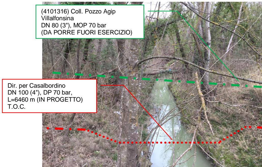
Foto n.5 – Vista Dir. per Casalbordino DN 100 (4") DP 70 bar, (IN PROGETTO) con attraversamento e metanodotto da porre fuori esercizio
