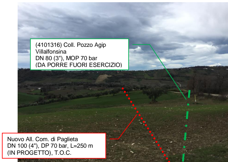
Foto n.4 – Vista Dir. per Casalbordino DN 100 (4") DP 70 bar, (IN PROGETTO) con T.O.C. e metanodotto da porre fuori esercizio
