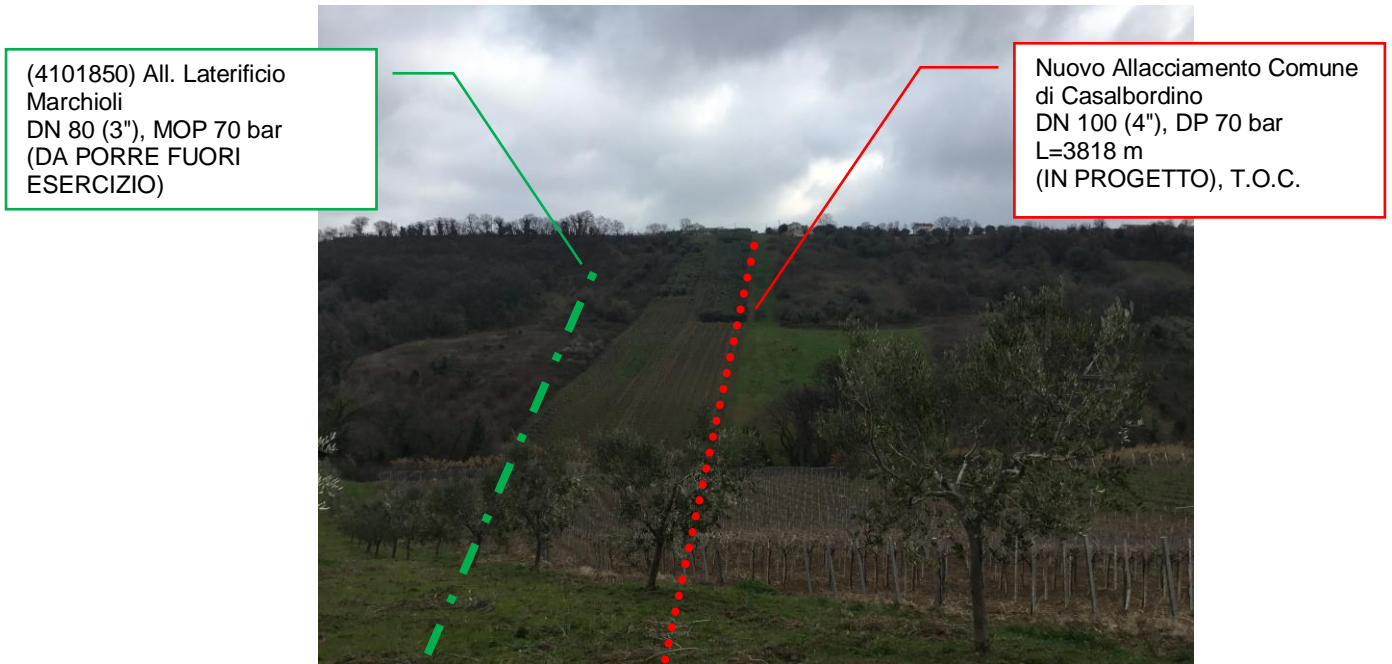
Foto n.7 – Panoramica metanodotto in progetto e metanodotto da porre fuori esercizio
