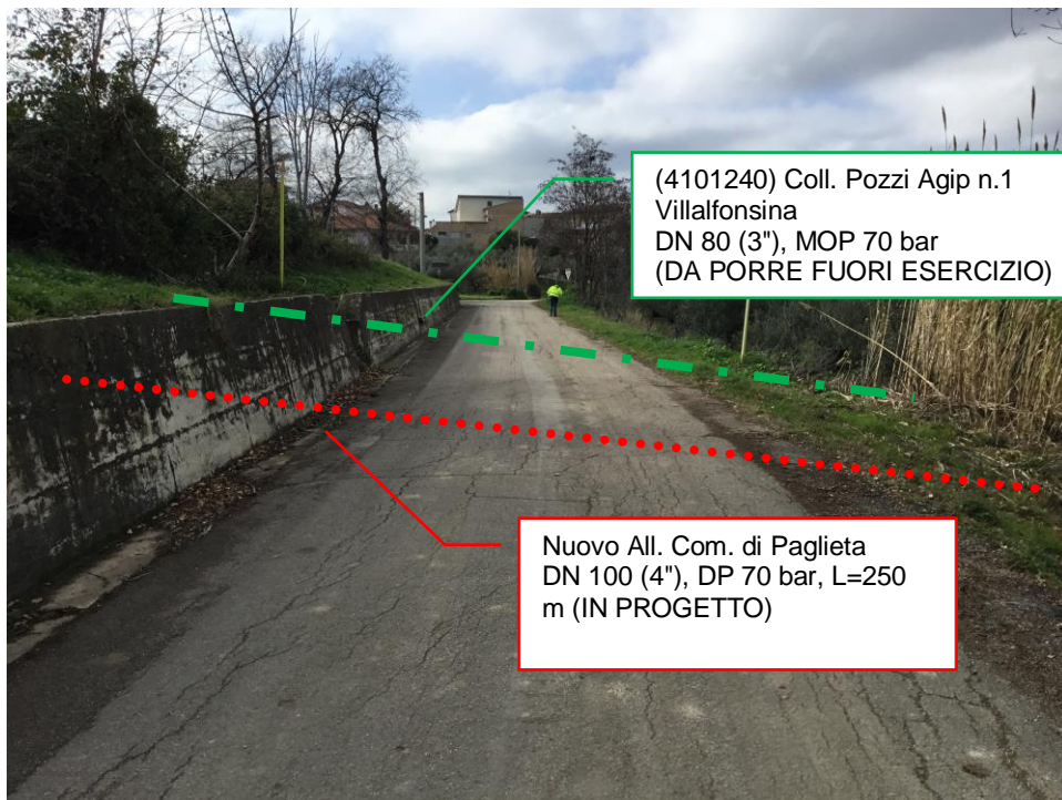
Foto n.3 – Vista metanodotto in progetto con attraversamento stradale e metanodotto da porre fuori esercizio
