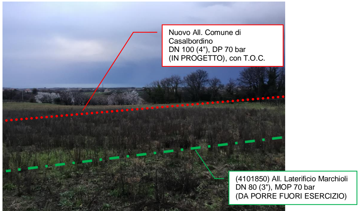
Foto n.1 – Vista Nuovo All. Comune di Casalbordino DN 100(4'') DP 70 bar con T.O.C. (IN PROGETTO)
