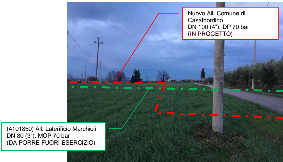
Foto n.2 – Vista metanodotto in progetto e metanodotto da porre fuori esercizio
