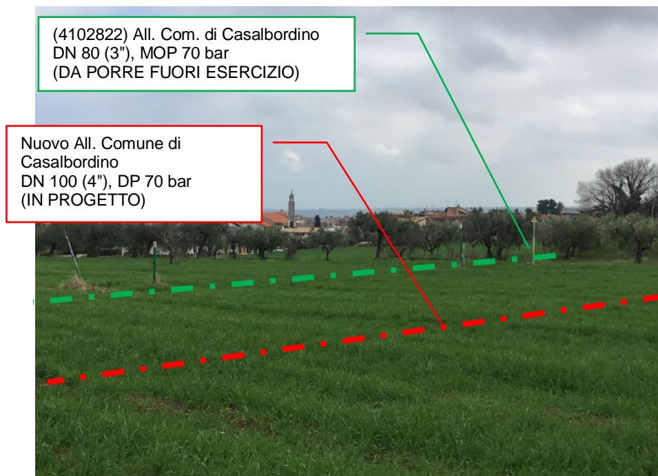
Foto n.6 – Panoramica metanodotto in progetto e metanodotto da porre fuori esercizio
