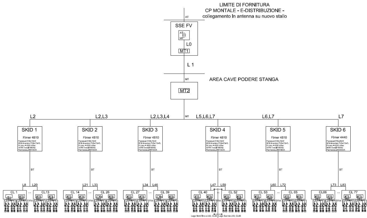
Figura 5. Schema a blocchi rete distribuzione impianto fotovoltaico
