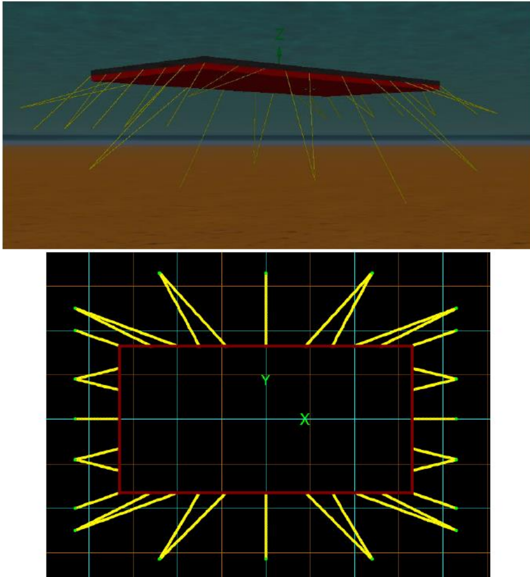
Figura 8. Schema modello di ormeggio
