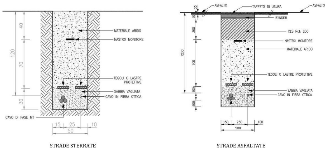
Figura 9. Sezione tipica di posa del cavidotto interrato Mt, in semplice terna, su strade sterrate (a sinistra) e su sede stradale (a destra)
