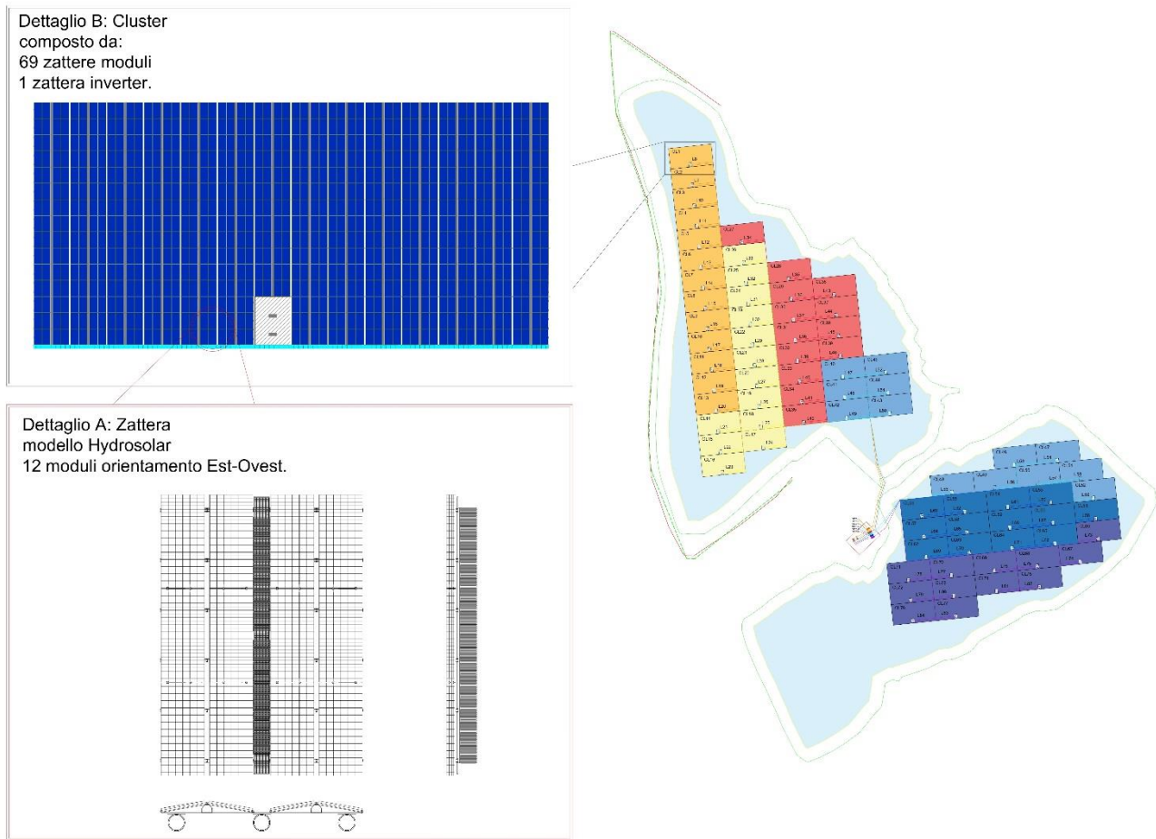
Figura 4. Layout impianto con composizione dei cluster
