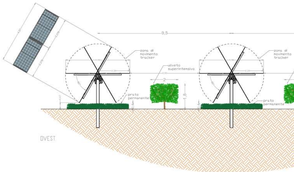
Figura 2-10: Angolo rotazione del tracker
