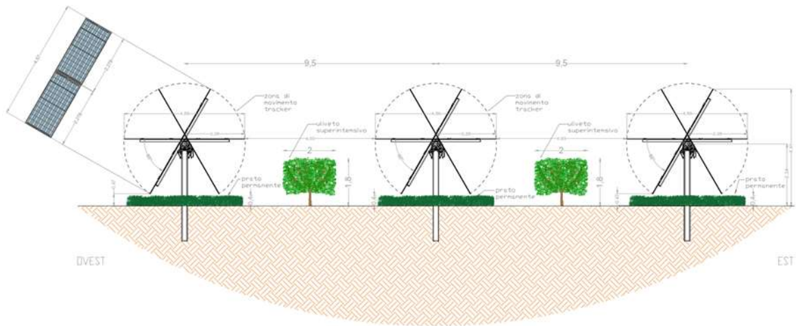
Figura 2-1: Sistema Agro-fotovoltaico
