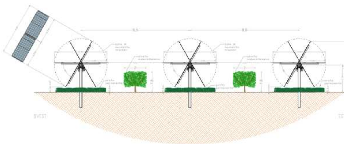
Figura 2-9: Schema impianto tracker – vista laterale
