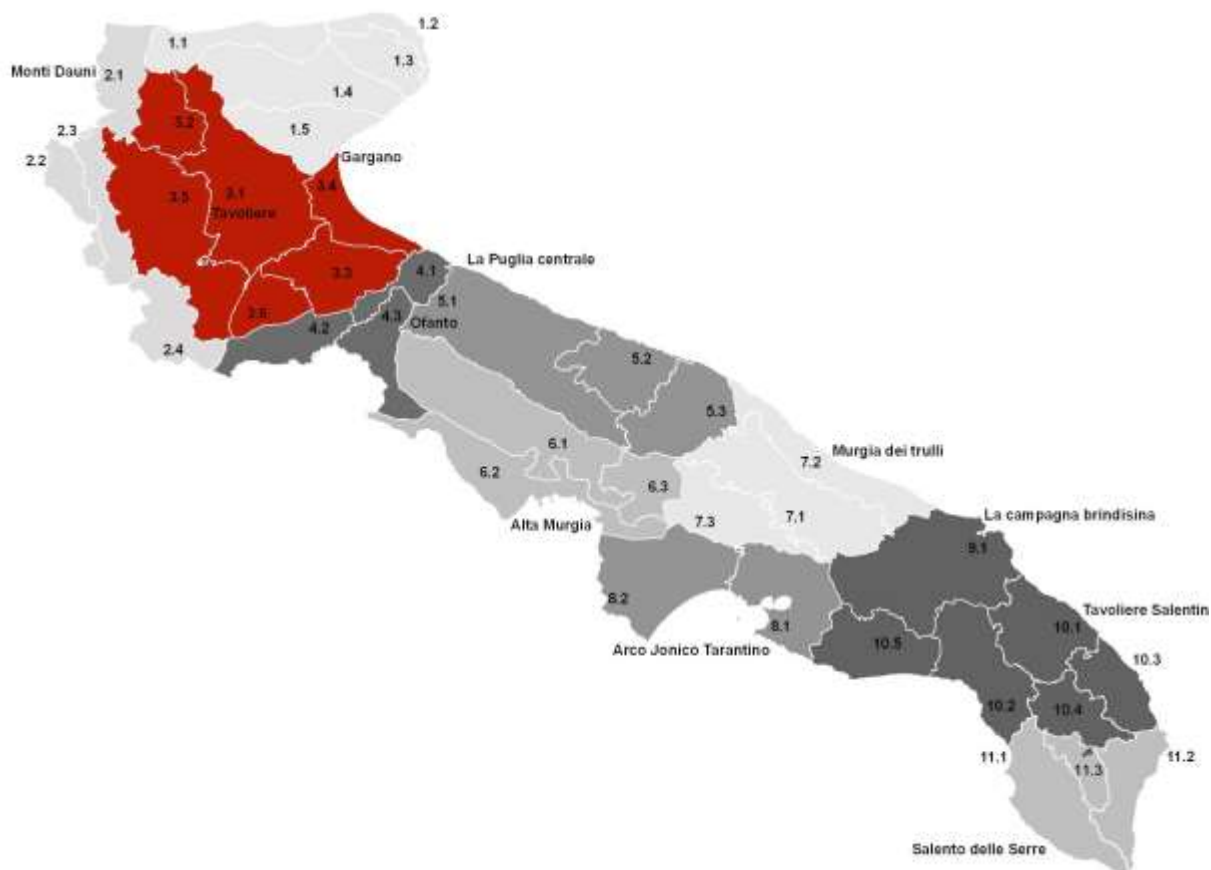
Figura 3-4: Carapelle nell'ambito del Tavoliere
