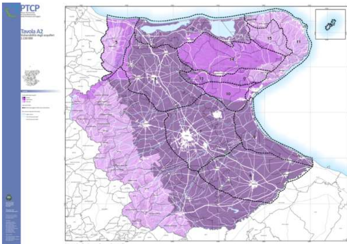
Figura 4-19: Vulnerabilità degli Acquiferi
