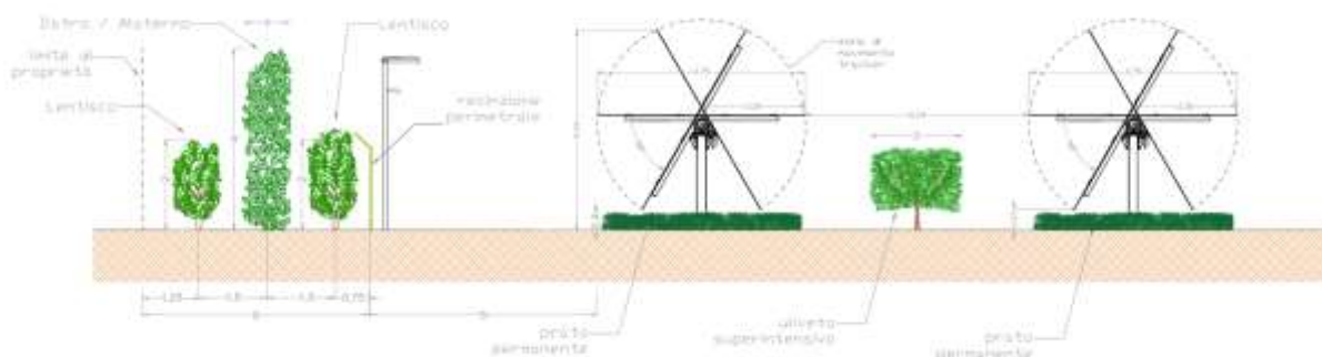
Figura 2-3: Layout misura mitigativa dell'impianto agro-fotovoltaico
