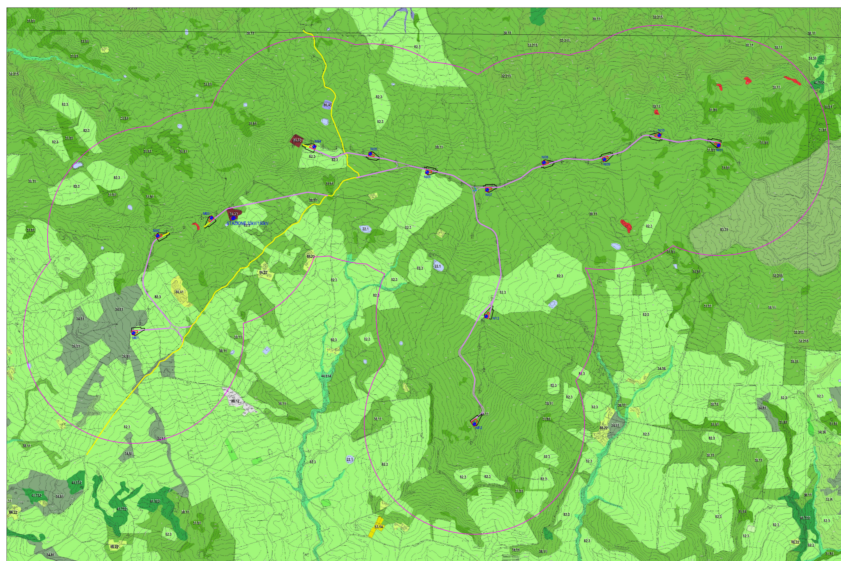
Carta degli habitat secondo Corine Biotopes. Scala 1:20.000
