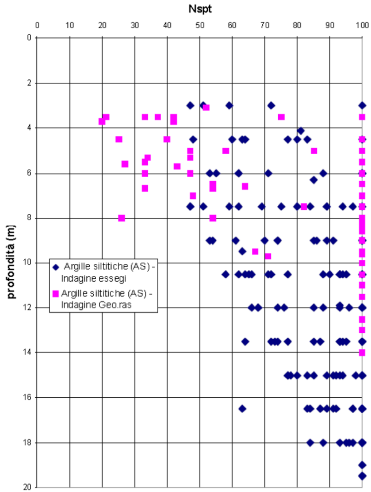
Figura 7-10: Risultati delle prove SPT nelle Argille slittiche
