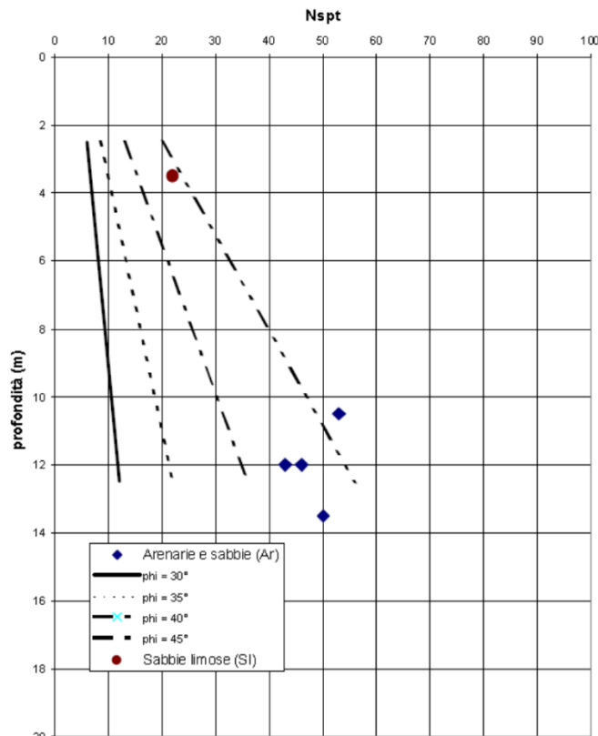
Figura 7-11: Risultati delle prove SPT nelle Arenaria e nelle Sabbie limose
