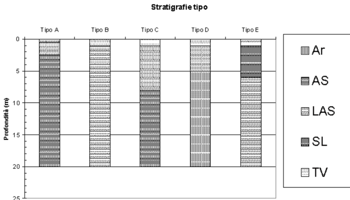
Figura 7-3: Stratigrafie tipo sito di Nicosia
