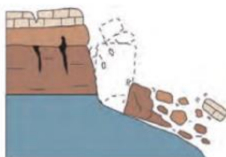
Figura 3-2: Esempio del processo di formazione dei depositi al piede dei versanti
