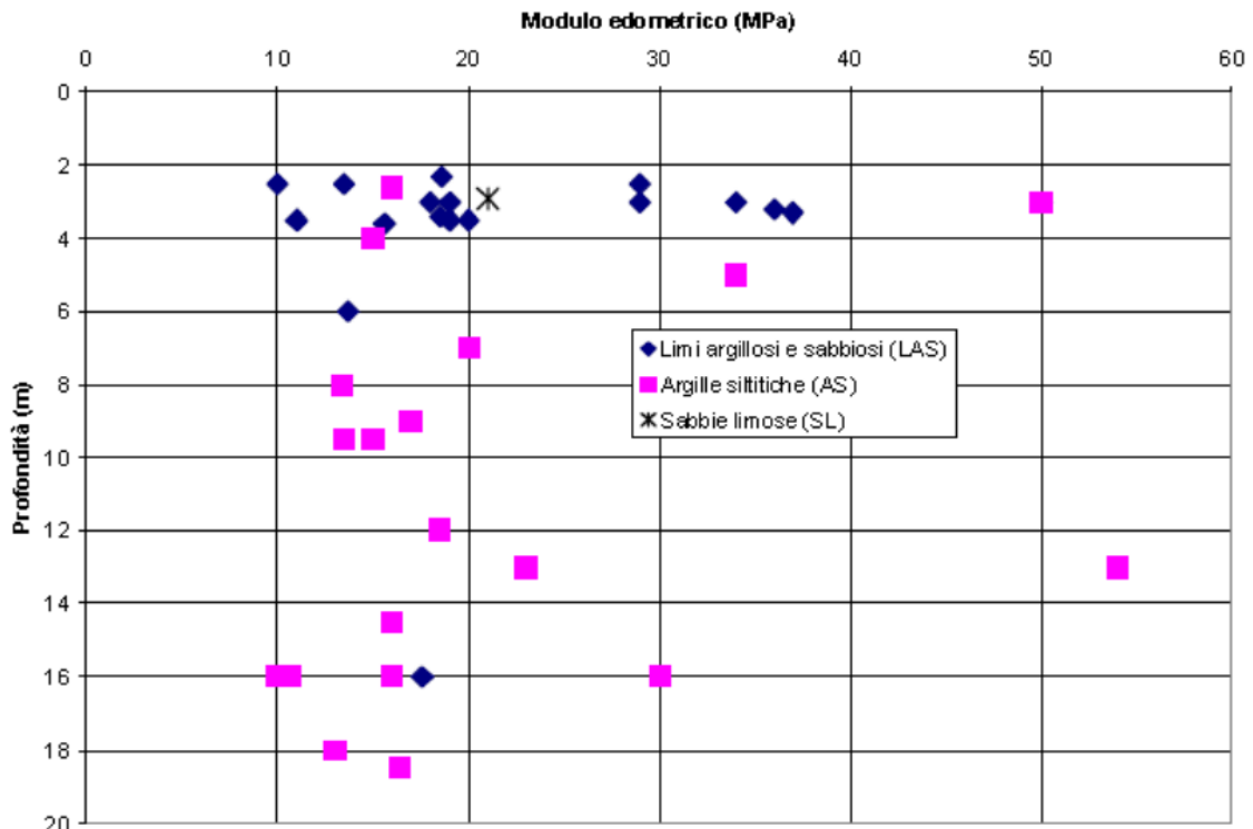
Figura 7-8: Moduli edometrici. Limi argillosi, Argille siltitiche, Sabbie limose
