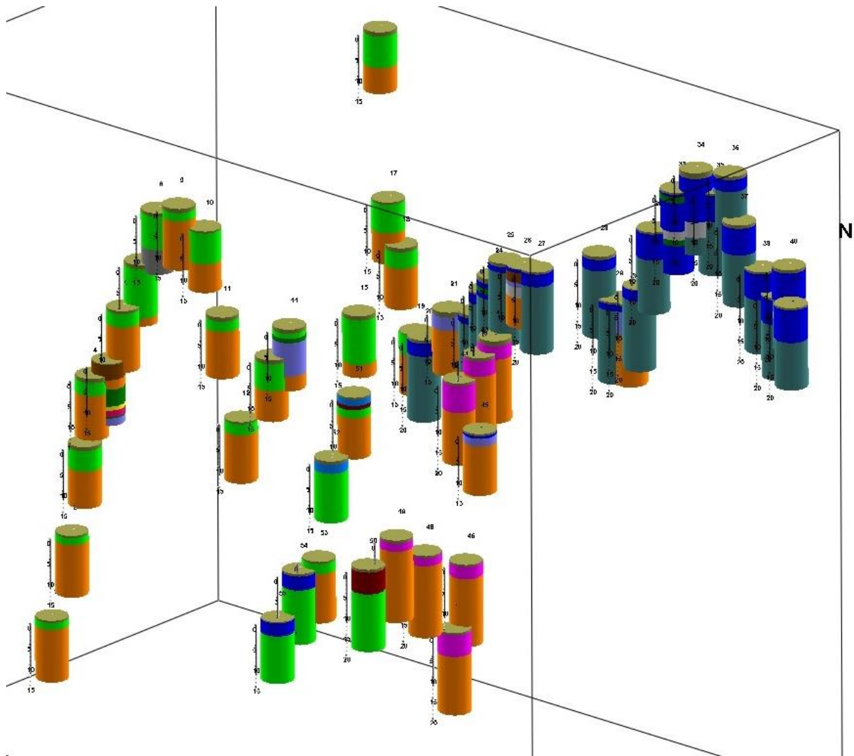
Figura 6-1: Visualizzazione 3D di tutti i carotaggi eseguiti
