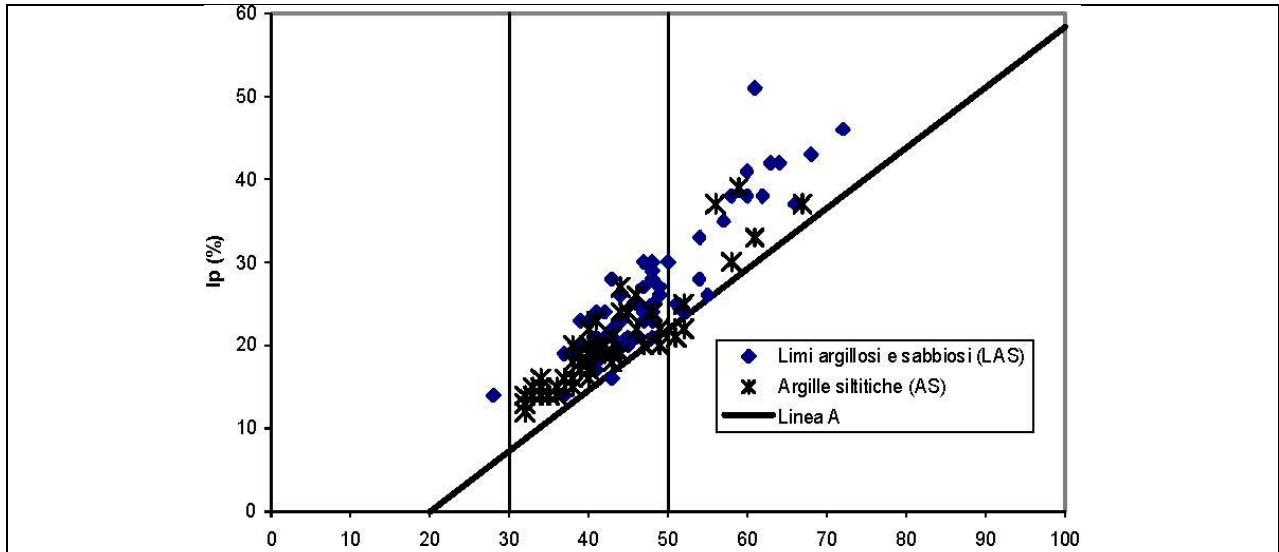
Figura 7-4: Carta di Casagrande: Limi argillosi e sabbiosi e Argille siltitiche
