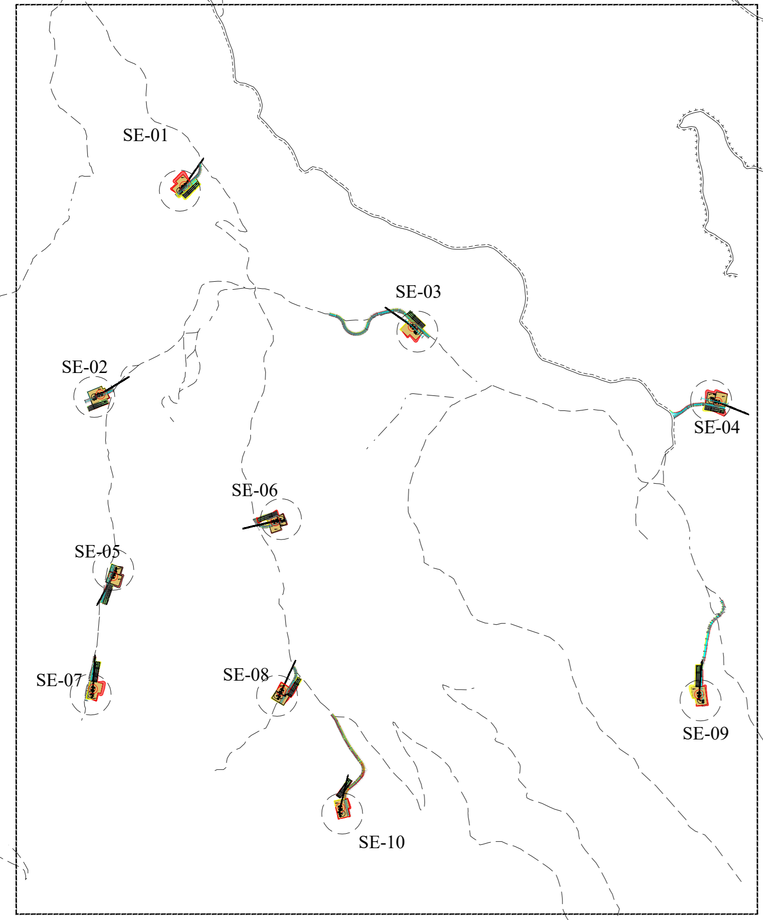
KEY PLAN IMPIANTO - AREA NORD: WTG DA SE-01 A SE-10
