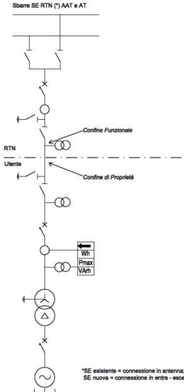
Esempio tipologico del collegamento con SSE di Terna per utenti attivi
