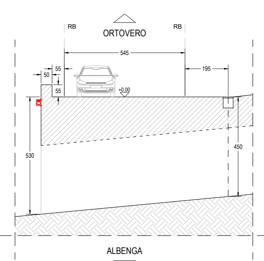
Sezione trasversale - 1:100
