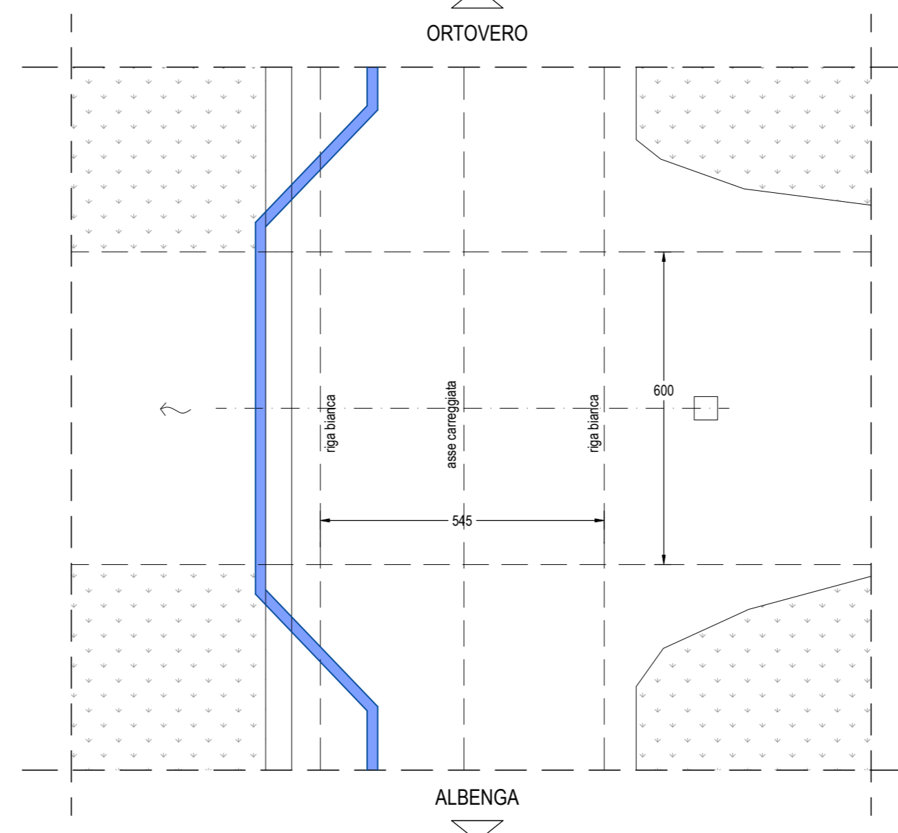
Planimetria generale attraversamento - 1:100
