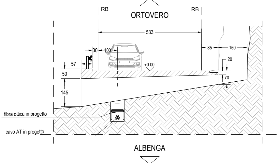
Sezione trasversale - 1:100
