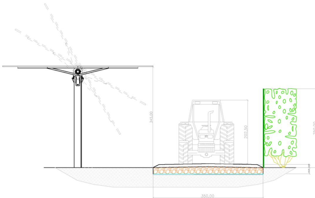
Figura 6: Sezione tipo strada perimetrale impianto.
