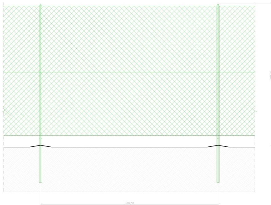
Figura 7: Prospetto tipo recinzione perimetrale.
