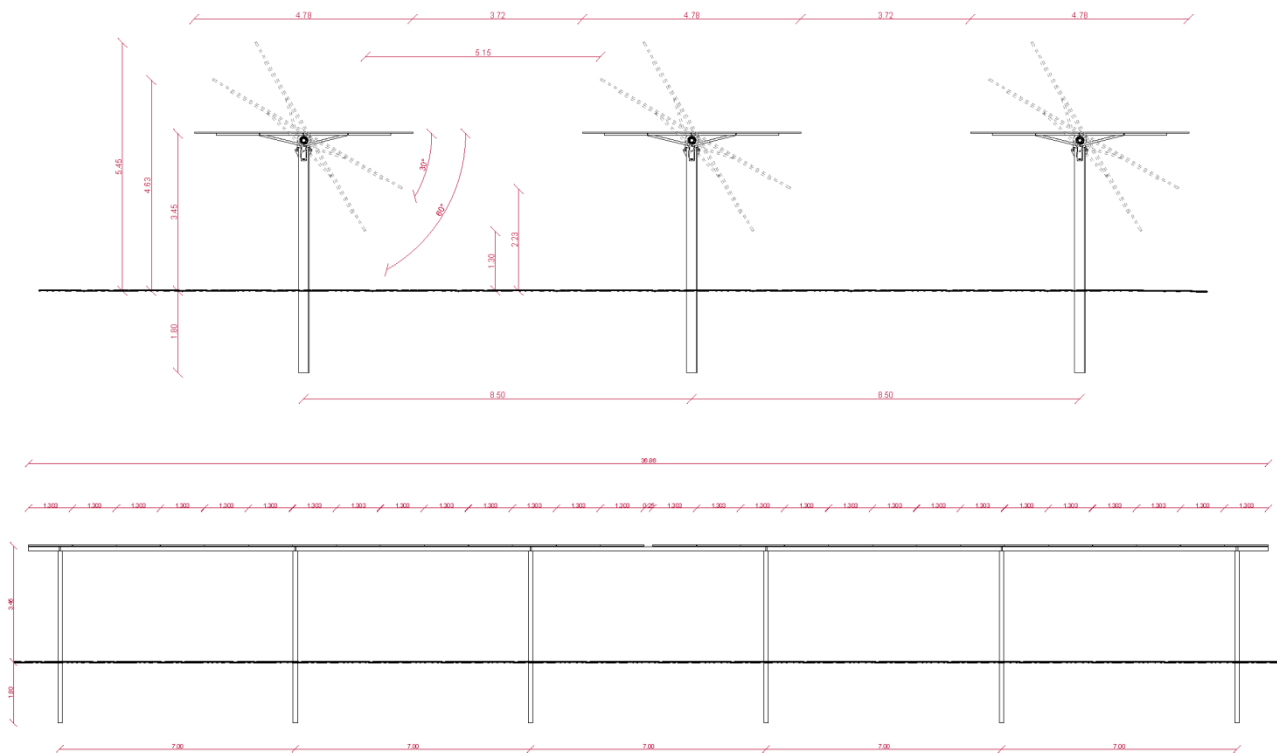
Figura 2: Sezioni tipo inseguitori monoassiali (trasversale – longitudinale).
