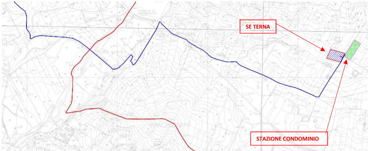
Figura 2 - Inquadramento di dettaglio della Stazione Elettrica (SE) e della Stazione Utente (SU) su cartografia CTR
