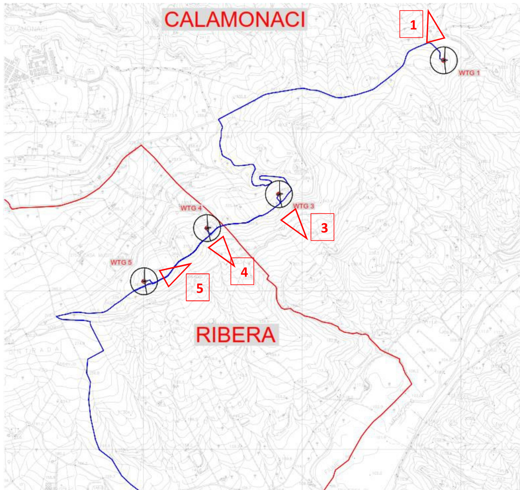
Figura 1 - Layout di progetto su CTR
