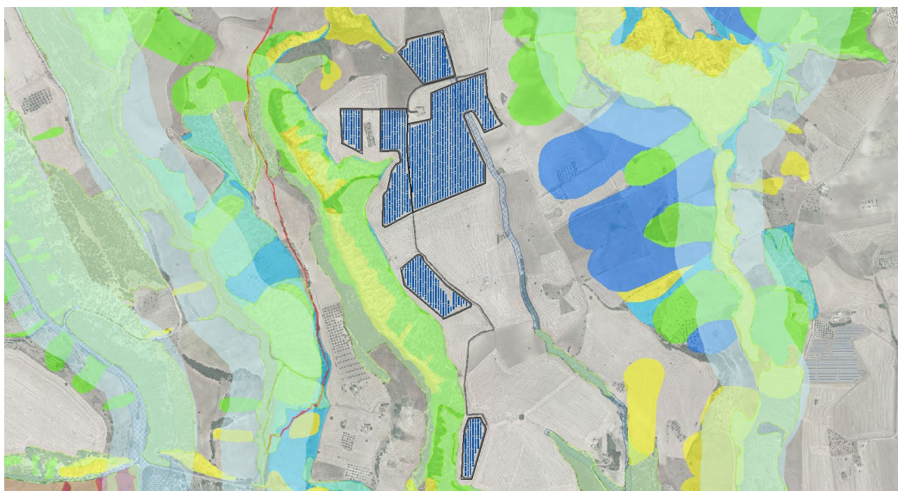
Figura 2 Aree di progetto in relazione ai vincoli e alle aree a rischio del PAI
