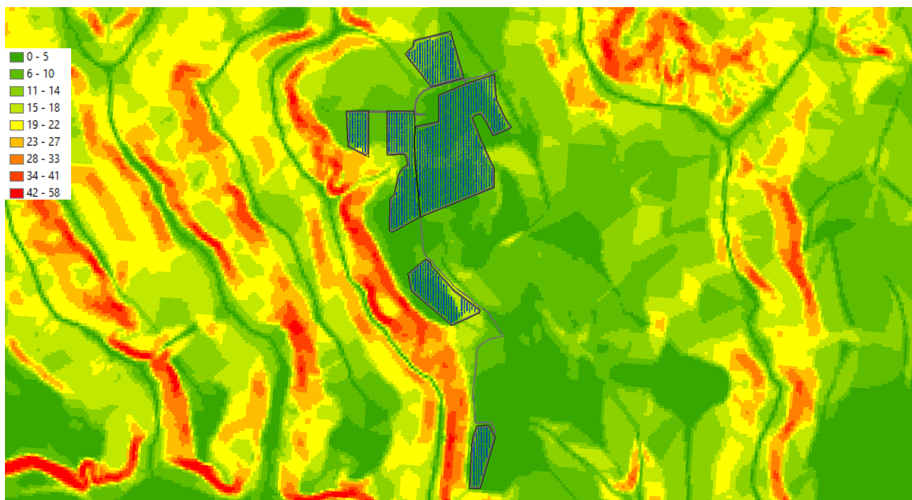
Figura 3 Aree di progetto in relazione alla Pendenza dei Versanti
