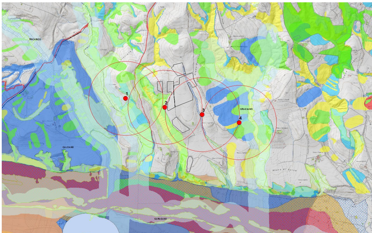
Figura 5 Ipotesi di utilizzo di aerogeneratori da 5MW su CTR
