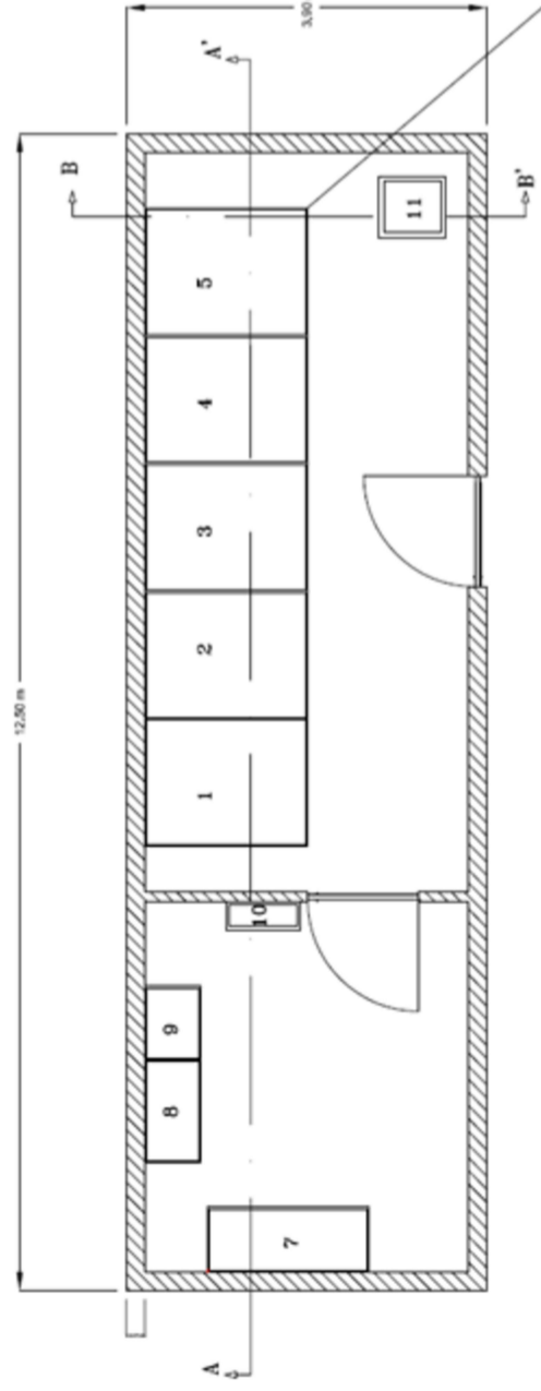
Sezione Pianta
