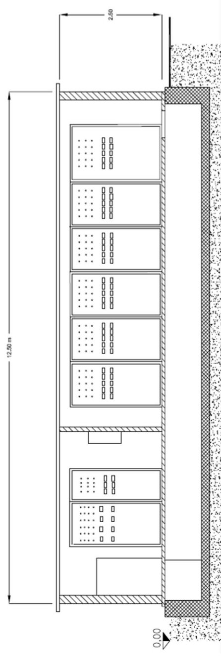
Sezione A-A
