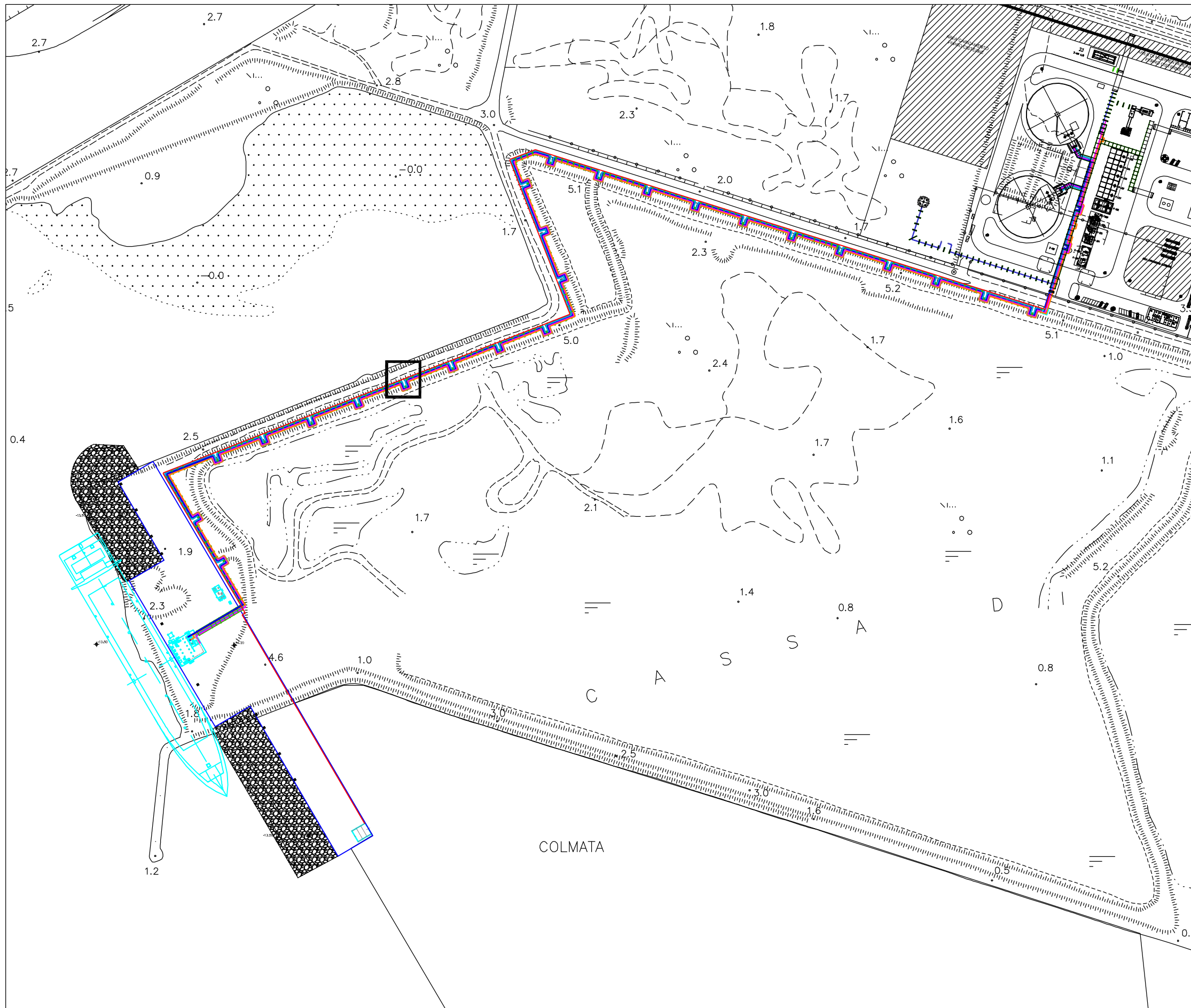
TRACCIATO CONDOTTE DI PROCESSO E ANTINCENDIO (COLLEGAMENTO BANCHINA - TERMINALE GNL)
