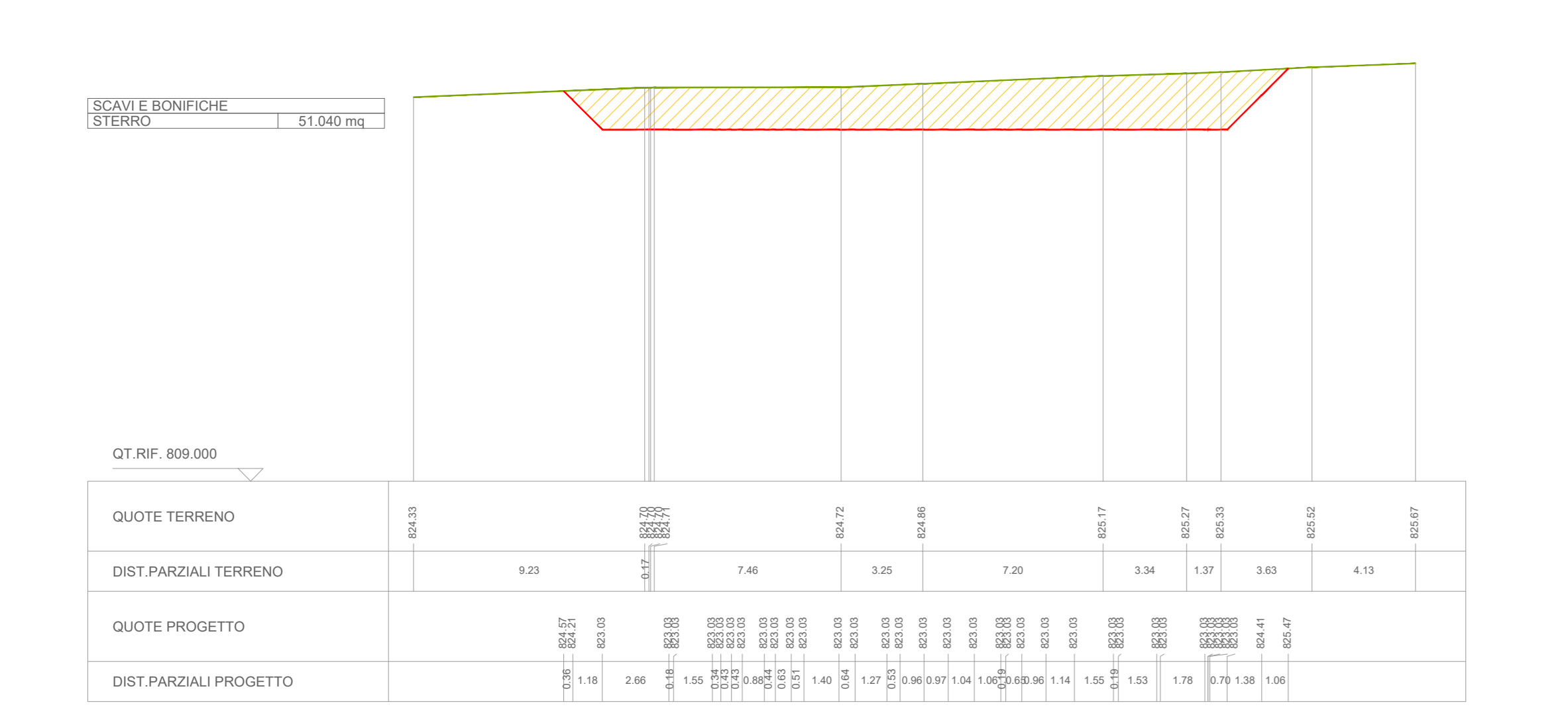
SEZIONI TRASVERSALI SCAVO DI FONDAZIONE RAL01 - SCALA 1:200
