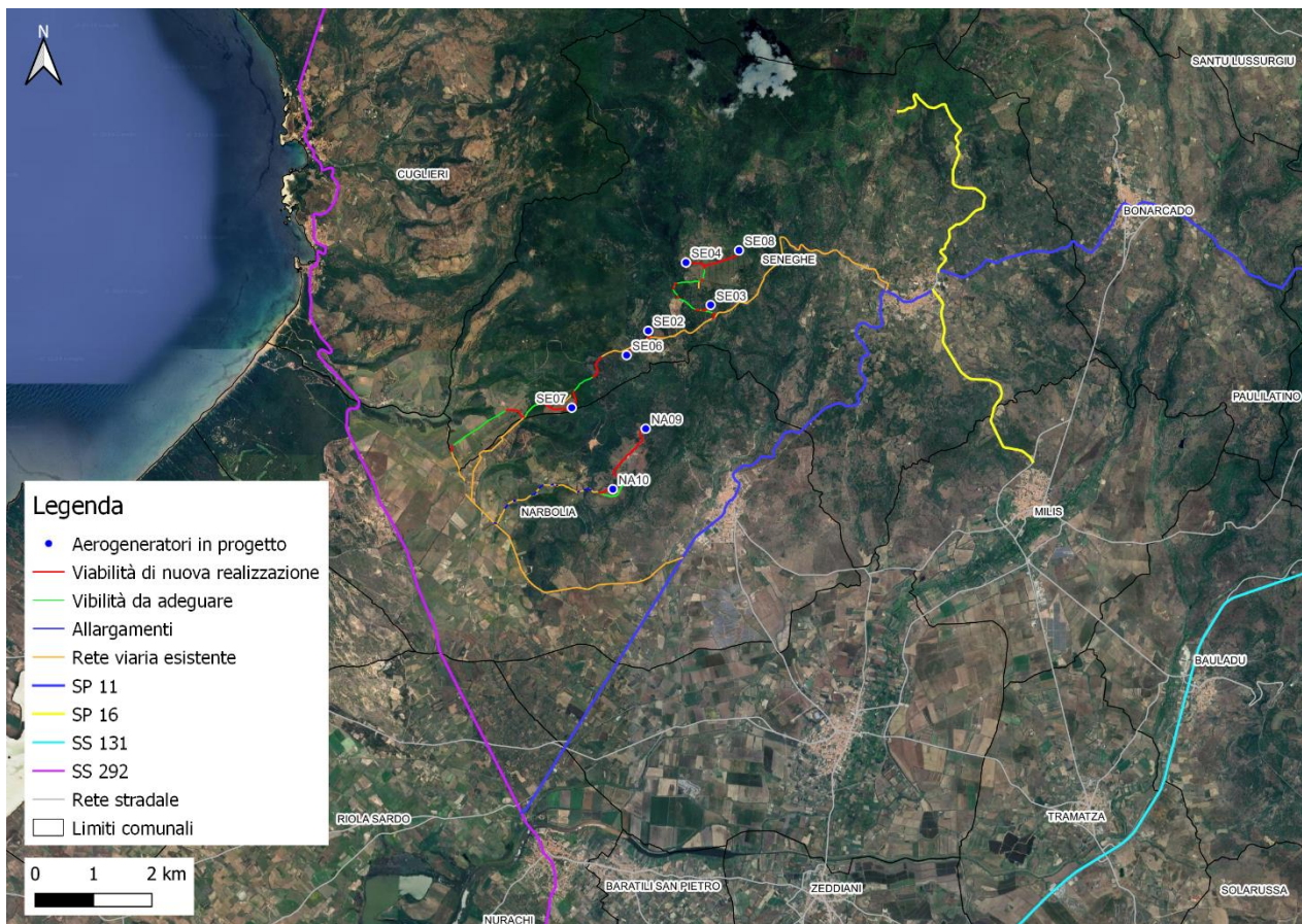
Figura 4.6 - Sistema della viabilità di accesso all'impianto e assi viari principali
