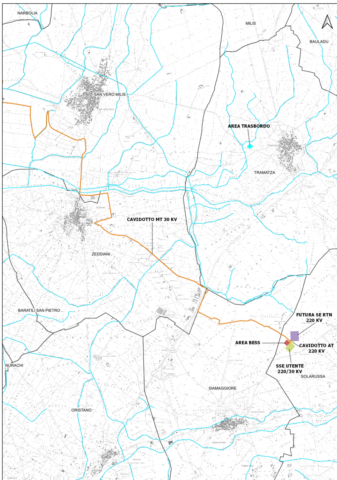
Figura 4.4 - Inquadramento geografico del cavidotto MT, dell'area trasbordo, dell'area BESS, della Futura SE RTN e della SSE Utente su CTR 1:10000
