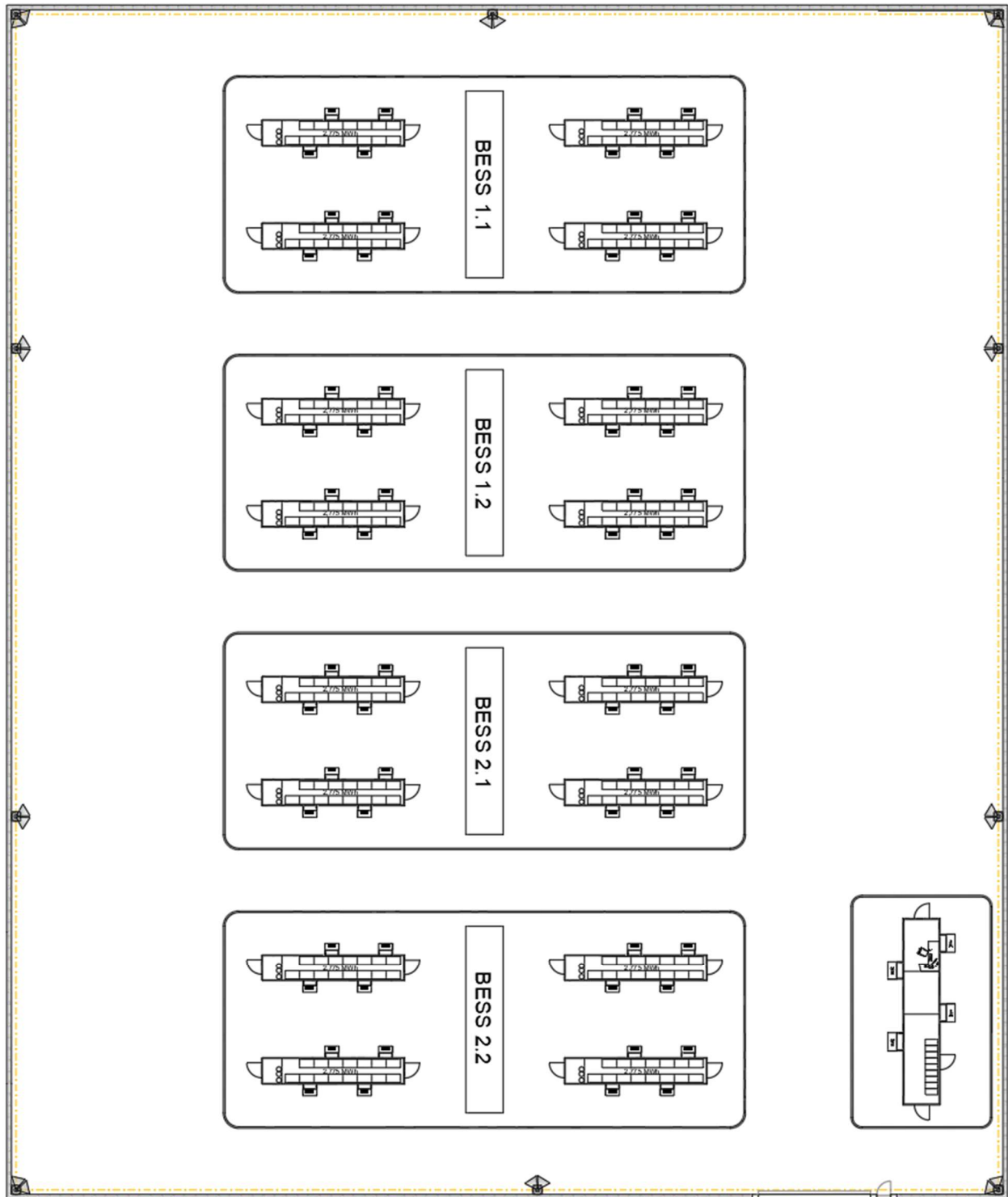
Figura 2.5 – Layout dell'impianto BESS all'interno dell'area dedicata
