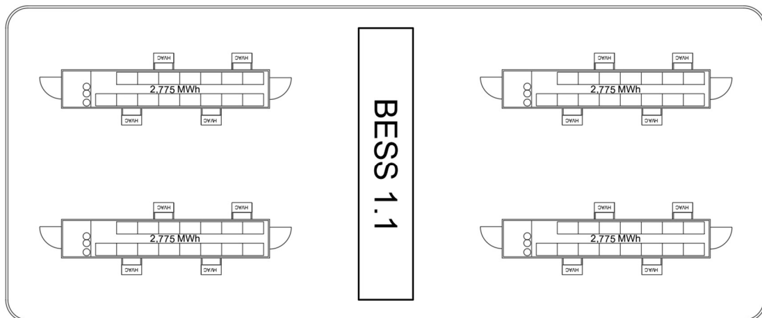
Figura 2.4 - Layout singolo battery block
