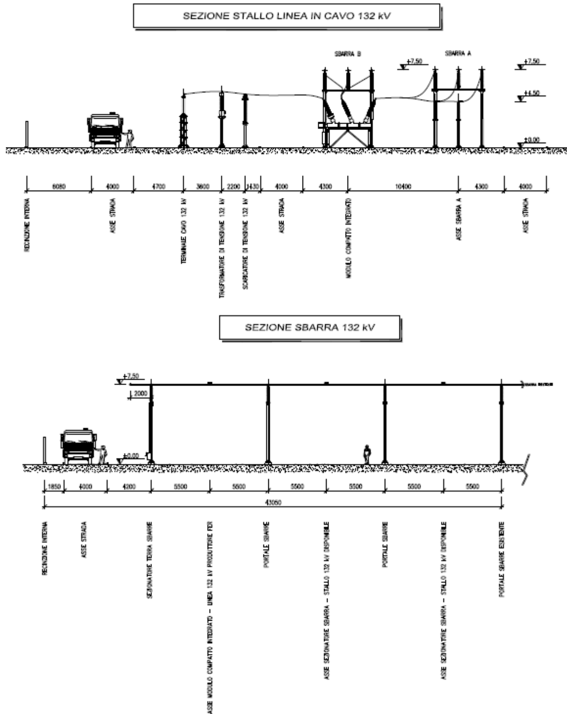
Figura 2 – Sezioni ampliamento SE Alfonsine SC estratte da documento No. 407453
