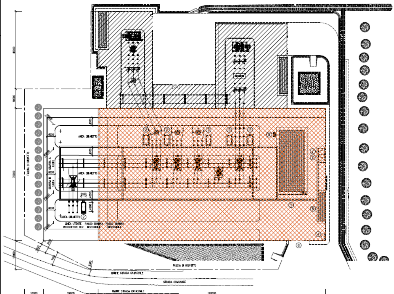
Figura 1 – Planimetria SE Alfonsine SC estratta da documento No. 407452 1
