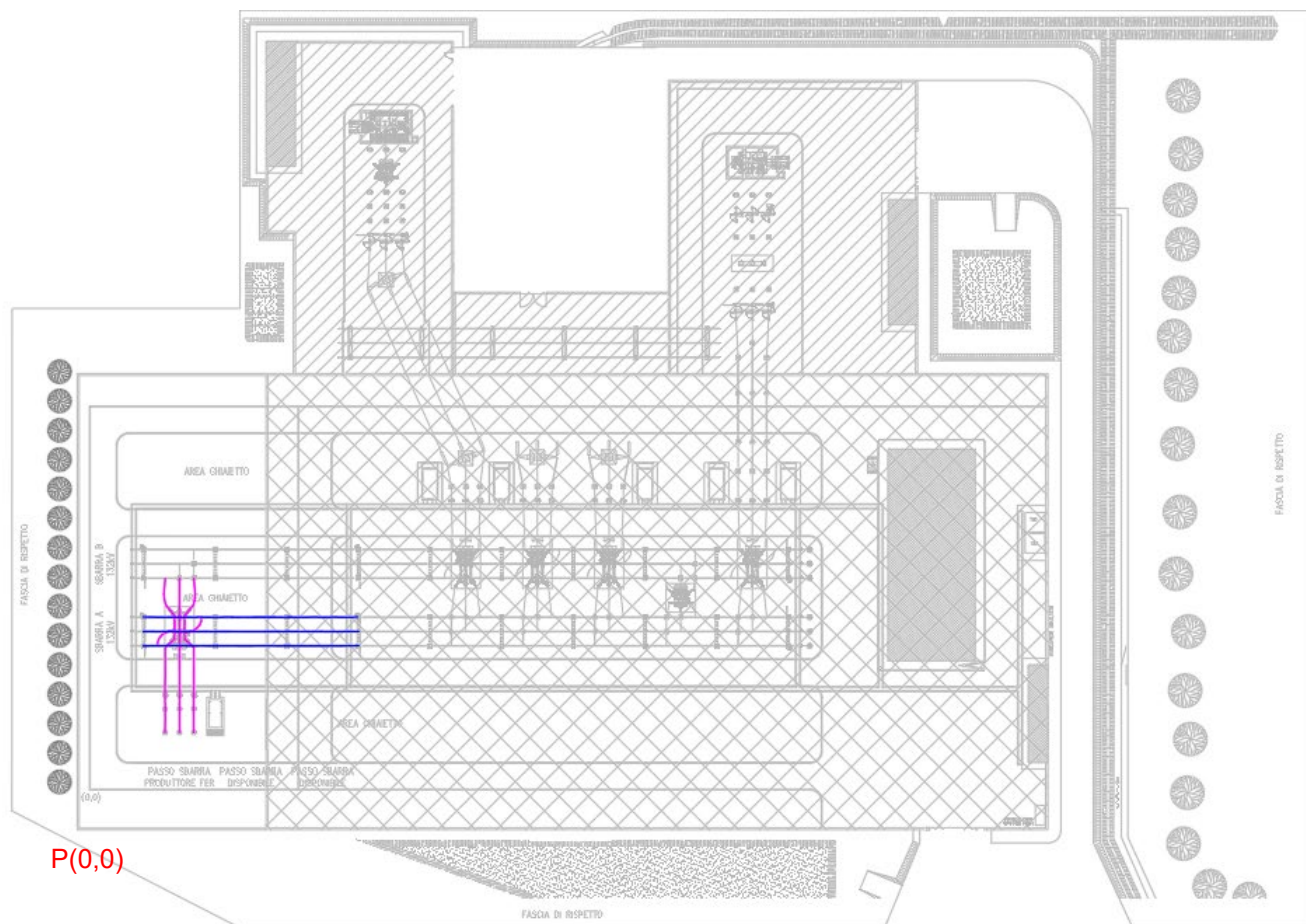
Figura 3 – Elementi attivi all'interno della planimetria
