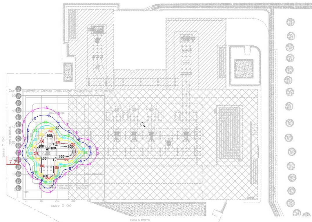
Figura 6 – Livelli di campo magnetico a 5 m dal piano di calpestio di stazione
