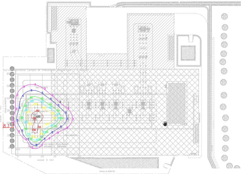
Figura 5 – Livelli di campo magnetico a 1 m dal piano di calpestio di stazione
