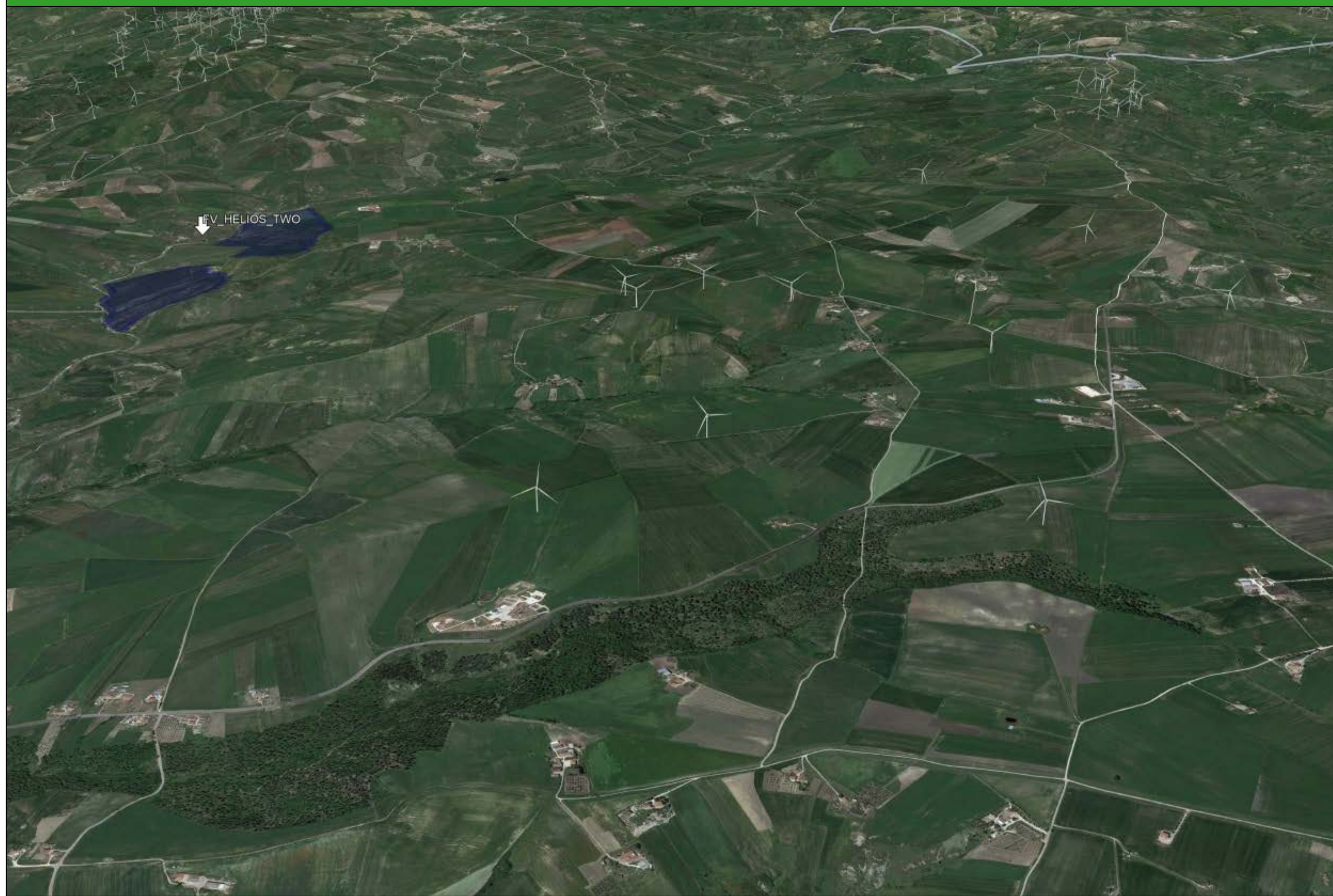
MODELLO 3D DELL'IMPIANTO ANTE OPERA VISTA NORD
