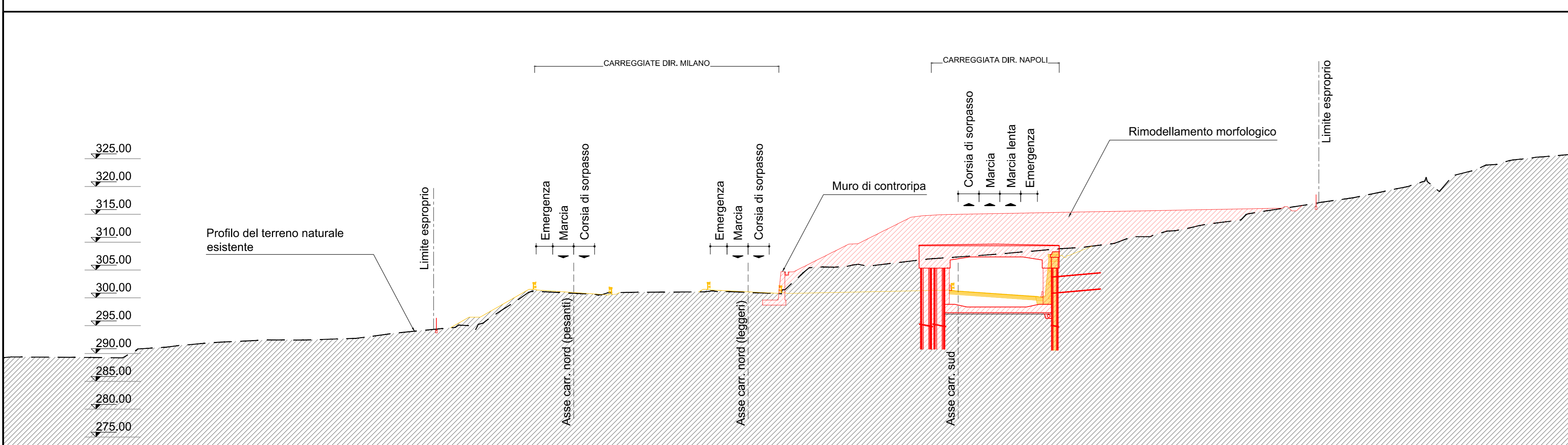
SEZIONE DI PROGETTO CON GALLERIA (S 142 - pk 10+200) SCALA 1:1000
