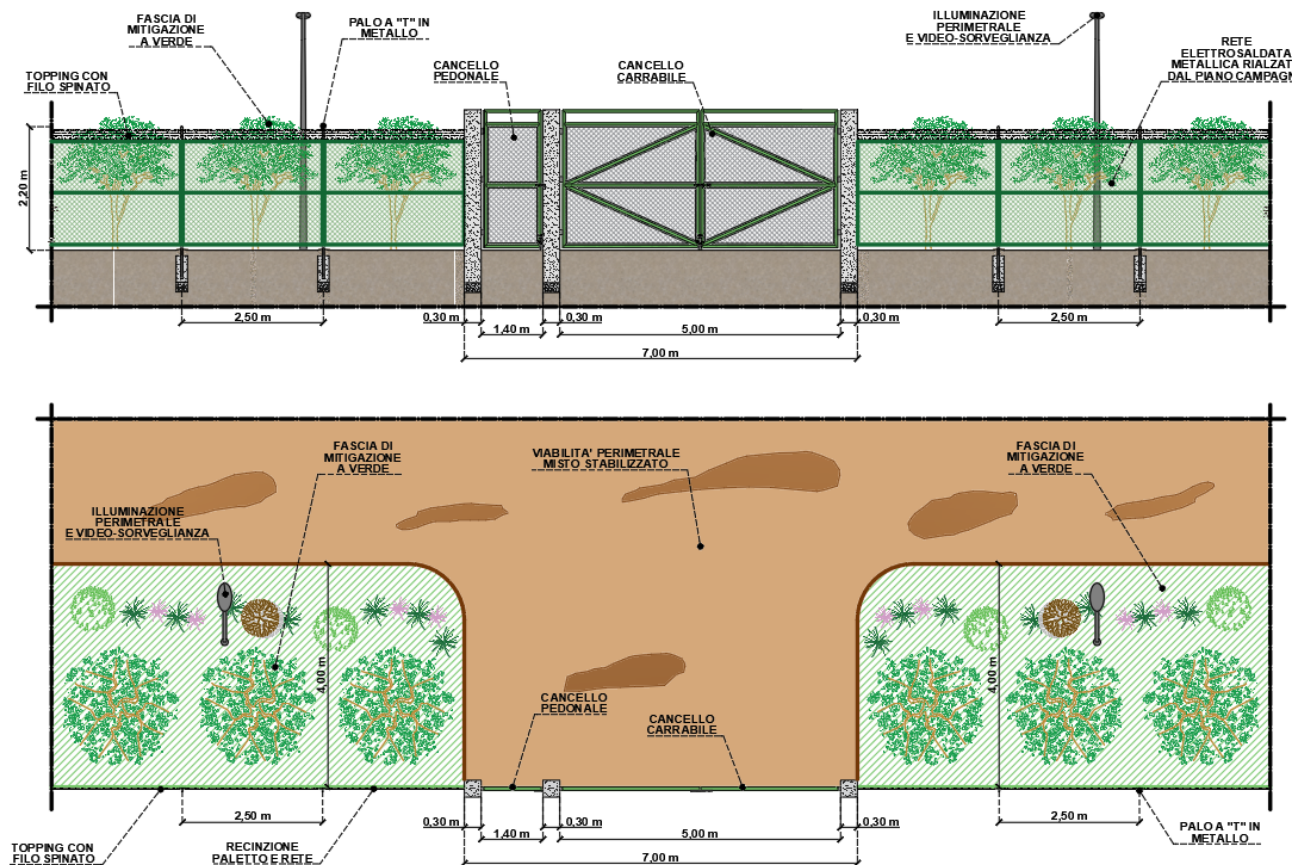
Figura 42: Dettagli Costruttivi Recinzione, Opere di Mitigazione e Viabilità perimetrale
