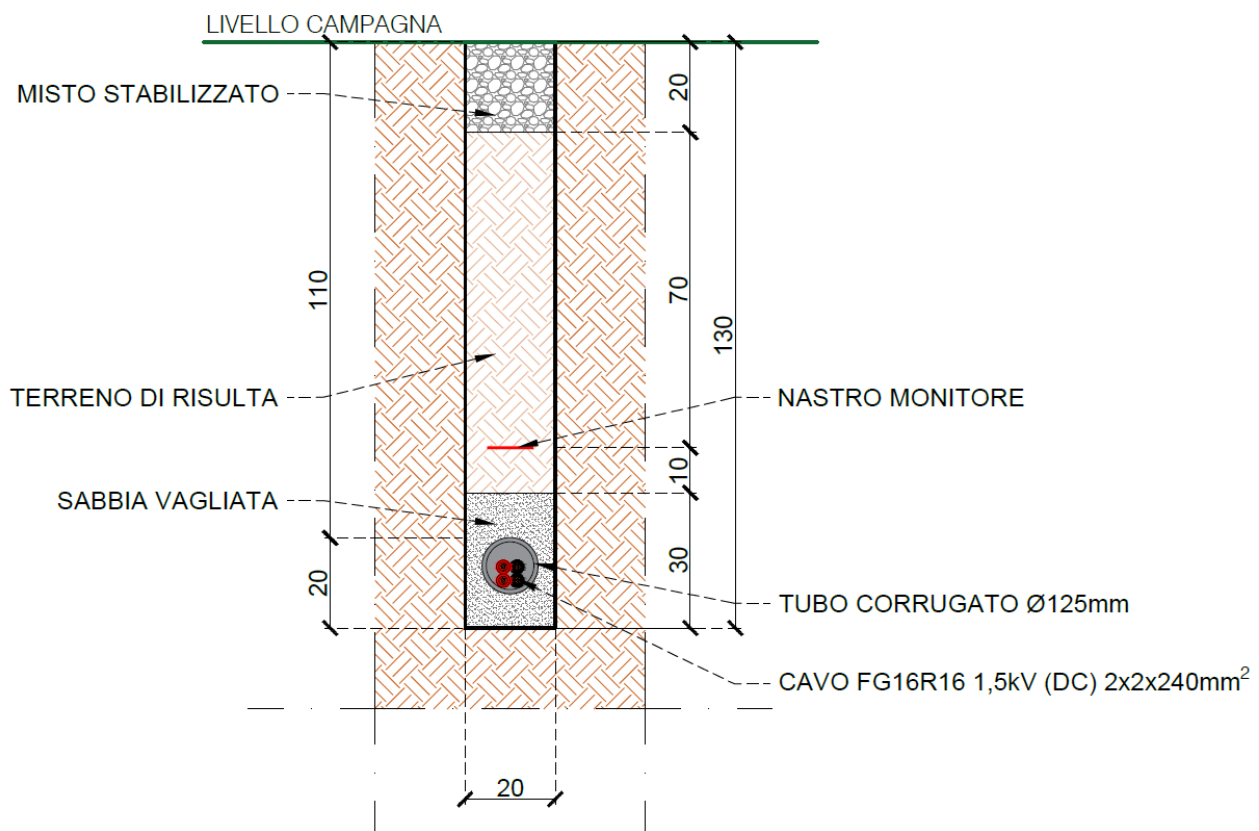
Figura 20: Sezione di scavo cavidotto BT DC (1 linea)
