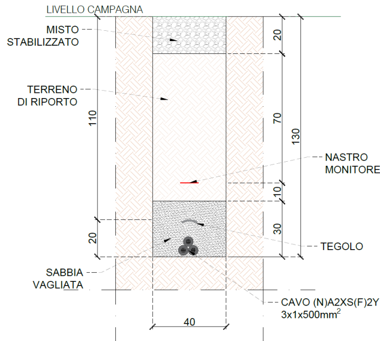
Figura 22: Sezione di scavo cavidotto AT AC
