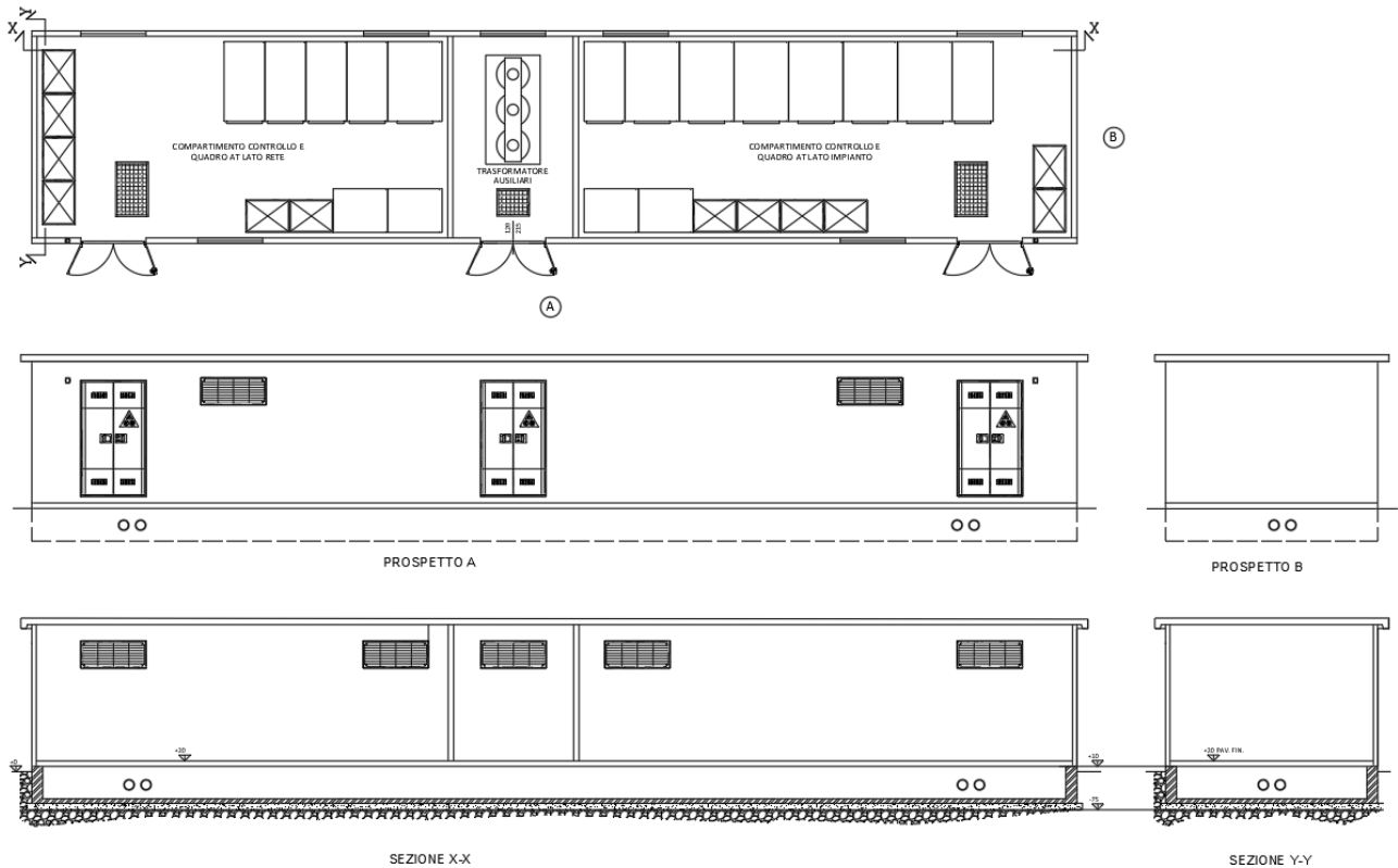
Figura 28: Pianta, Prospetti e Sezioni Cabina di Raccolta
