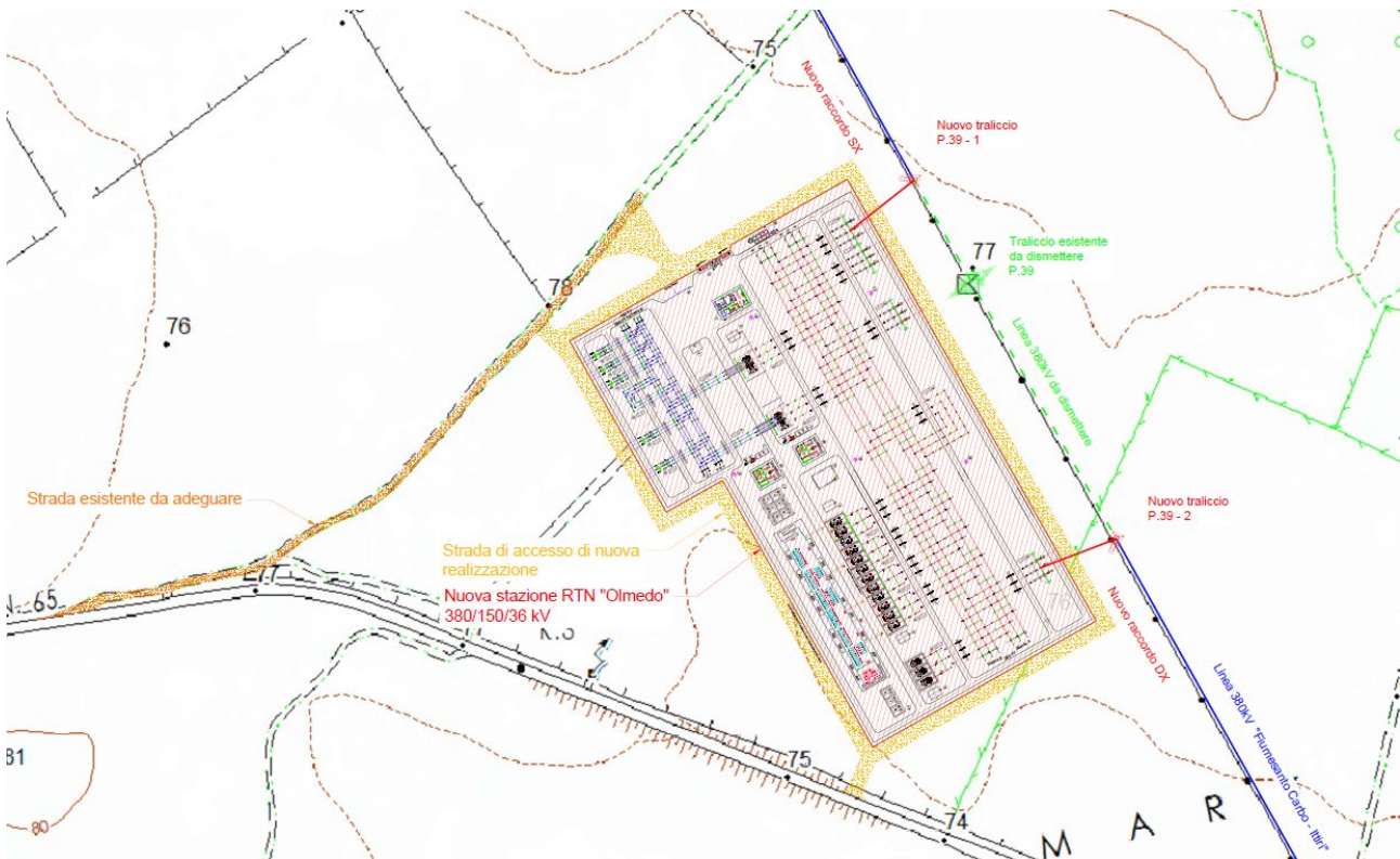
Figura 33: SE Olmedo 380 e raccordi linea 380 Kv Elaborato di riferimento "2022_Z_Tav.02b Inquadramento generale su CTR"
