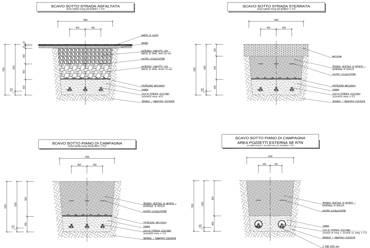
Figura 38: Sezione di scavo Connessione
