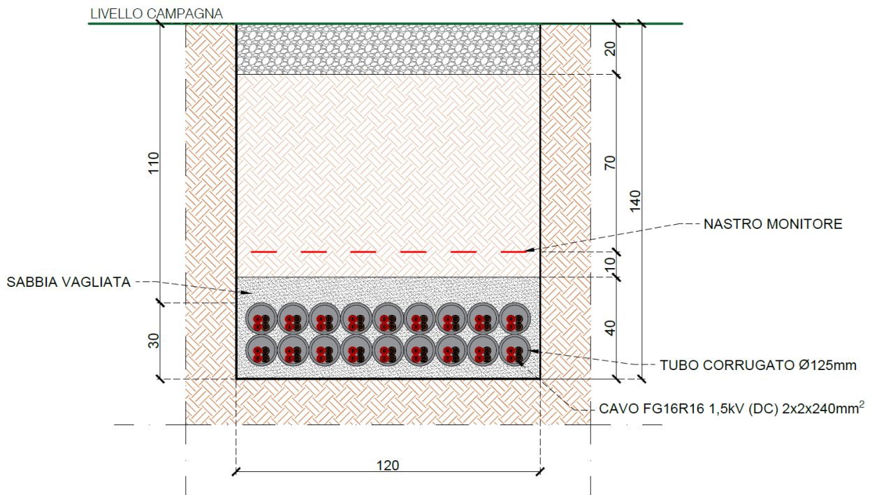
Figura 21: Sezione di scavo cavidotto BT DC (18 linee)
