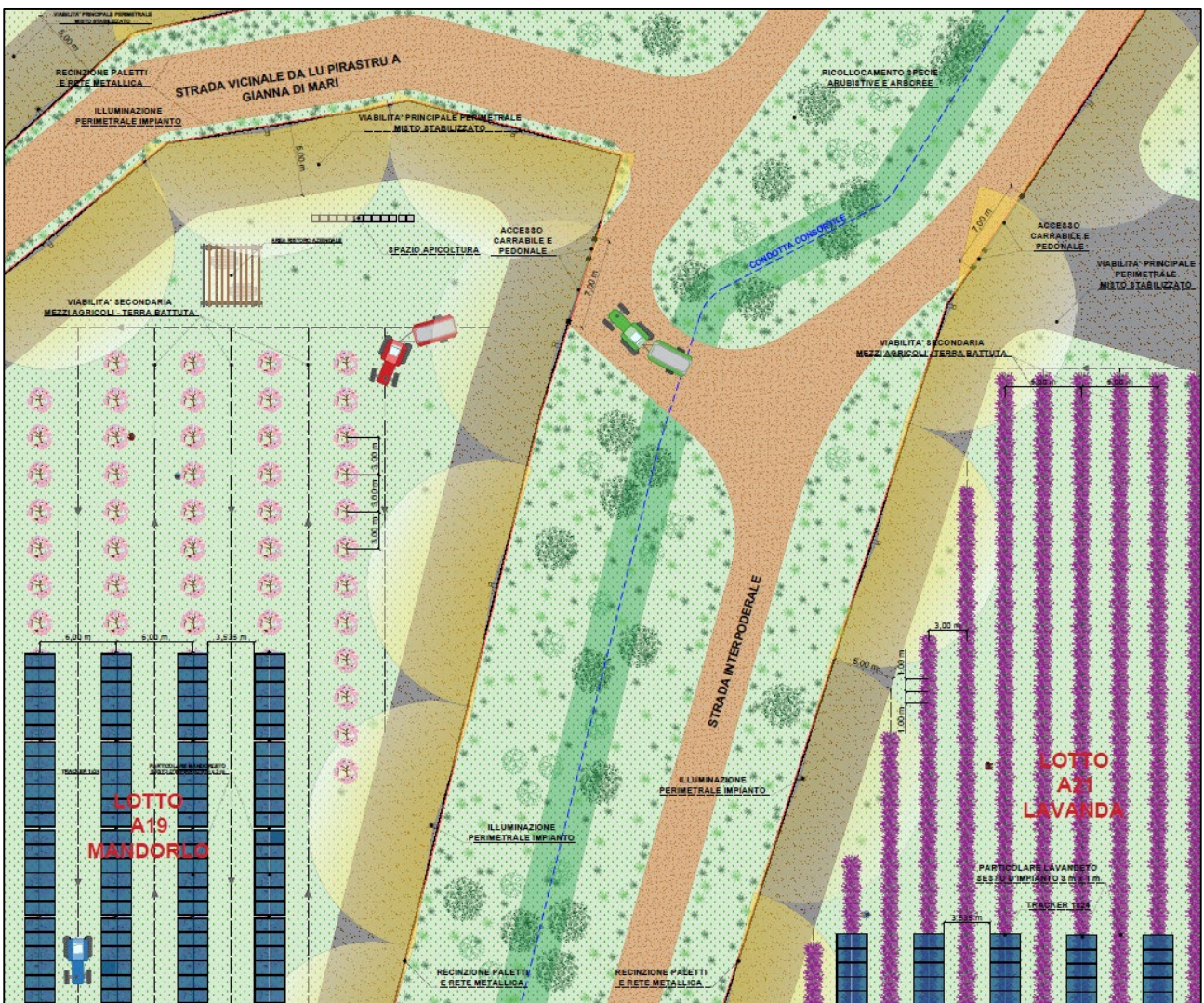
Figura 43: Evidenza del sistema viario interno e dell'integrazione tra sistema agricolo e fotovoltaico Riferimento Elaborato Grafico "2202_T.P.11_Stralcio planimetria di dettaglio impianto agrivoltaico"
