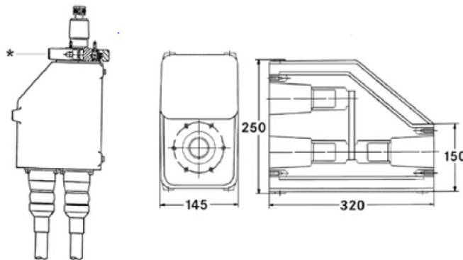
Figura 37: Sezione tipo del giunto "Y" previsto
