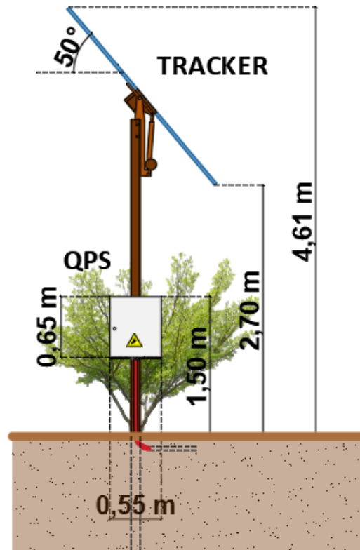
Figura 18: Particolare posizionamento QPS su tracker inclinato a 50°
