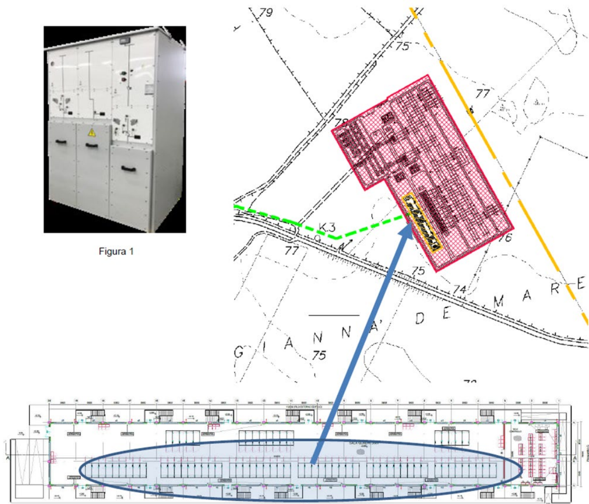
Figura 34: Quadri arrivo produttore – Fabbricato 36 kV in SE Olmedo 380 Elaborato di riferimento "2022_Z_Tav.24a Edificio quadri 36 kV Piante e Prospetti"
