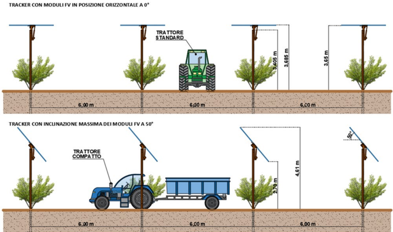
Figura 16: Particolare disposizione moduli su tracker: evidenza altezze dal suolo
