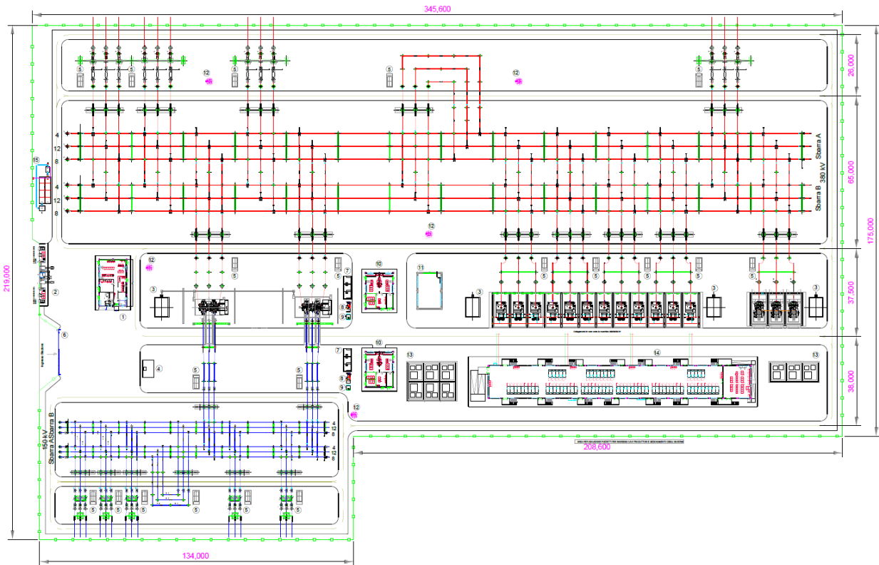
Figura 40: Planimetria SE Olmedo 380/150/36 kV Riferimento elaborato “2202_Z_Tav.09_Planimetria elettromeccanica Stazione RTN”
