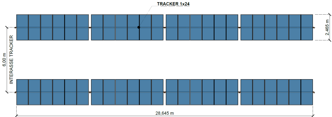
Figura 1: Vista in Pianta delle strutture (c.d. tracker)
