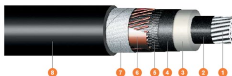
Figura 6: Cavo alluminio AT
