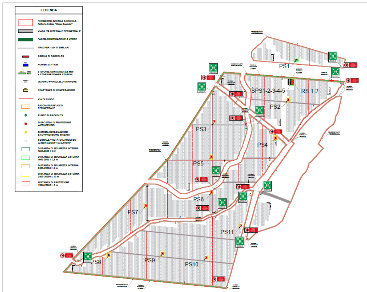
Figura 4: Planimetria antincendio con disposizione apparecchiature Riferimento elaborato grafico - "2202_T.P.24 Planimetria prevenzione incendi"
