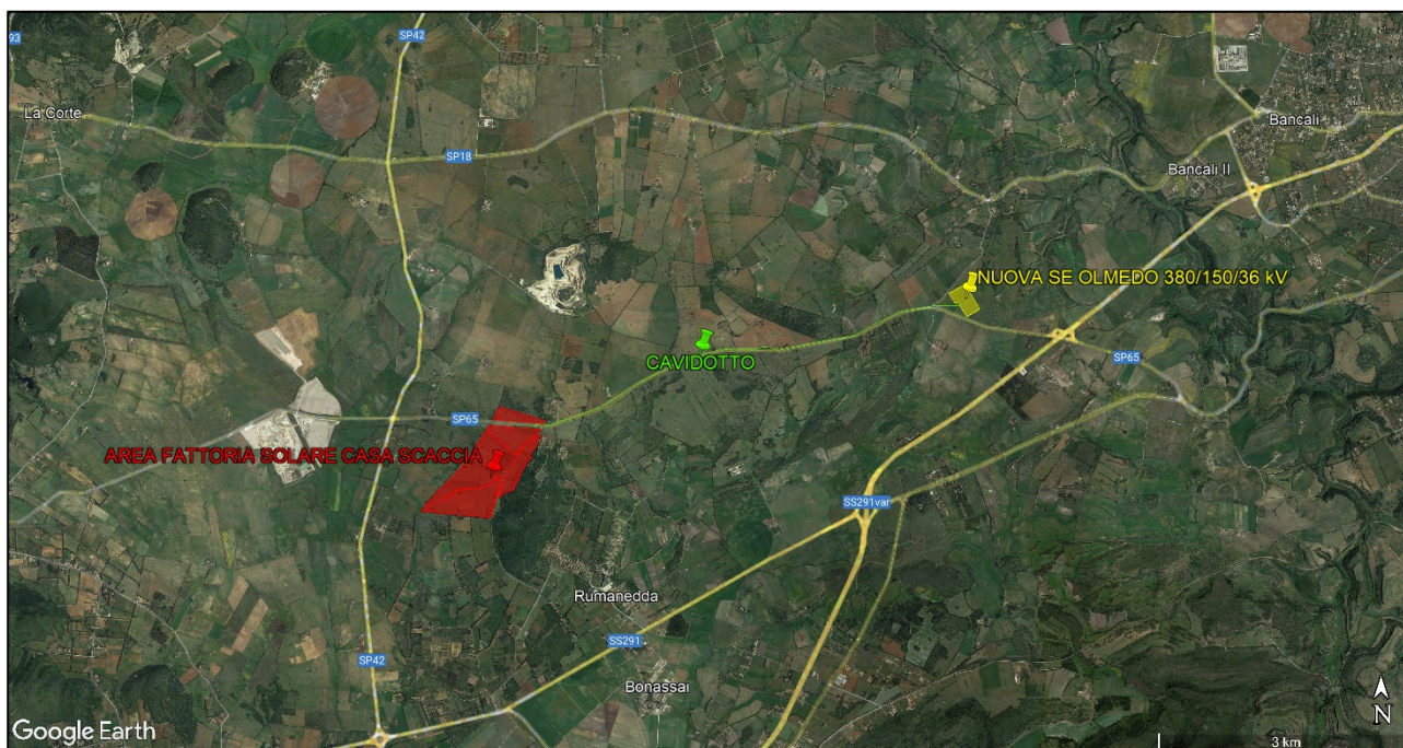
Figura 3: Inquadramento Area impianto, percorso cavidotto e area nuova SE Olmedo su Ortofoto
