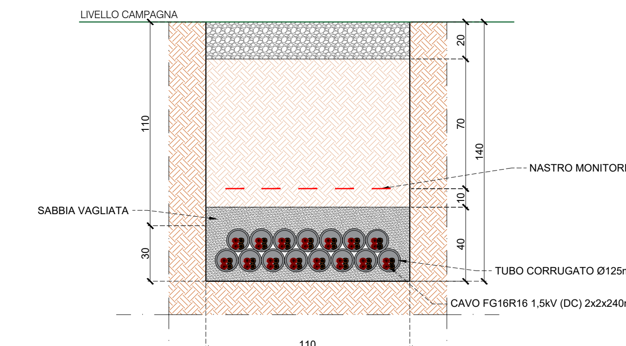
SEZIONE DI SCAVO DC 15
