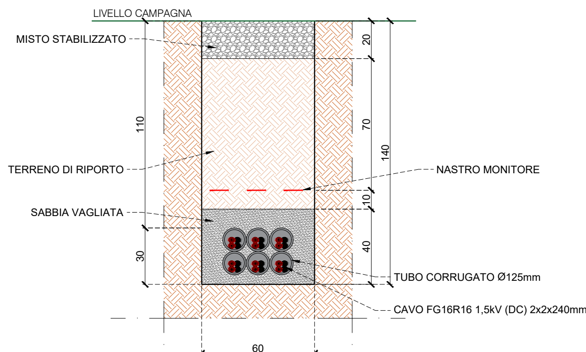
SEZIONE DI SCAVO DC 6
