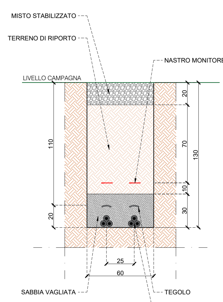
SEZIONE DI SCAVO AC 2
