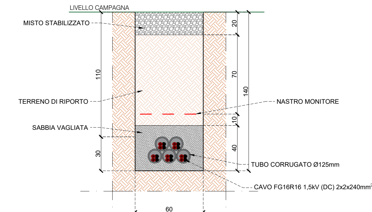
SEZIONE DI SCAVO DC 5
