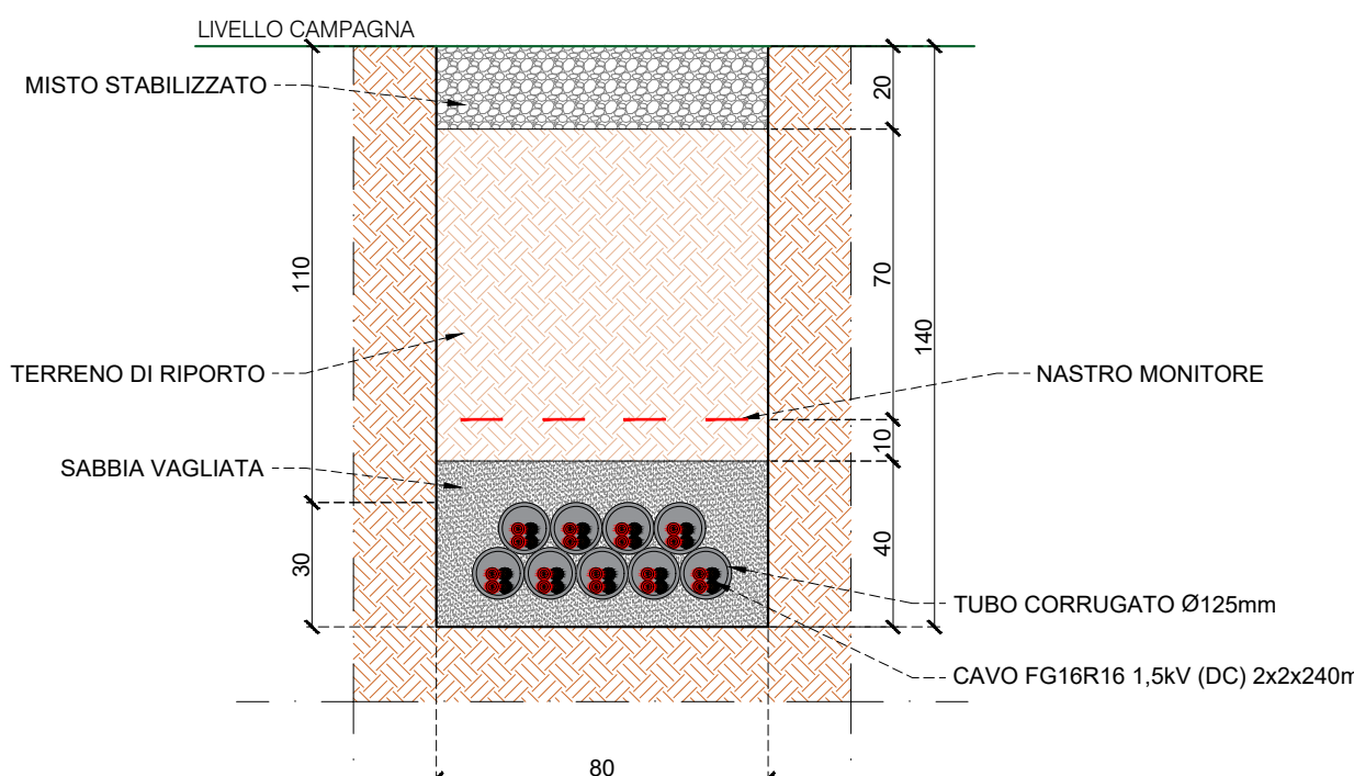
SEZIONE DI SCAVO DC 9
