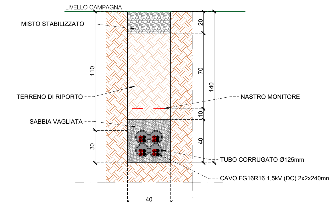
SEZIONE DI SCAVO DC 4
