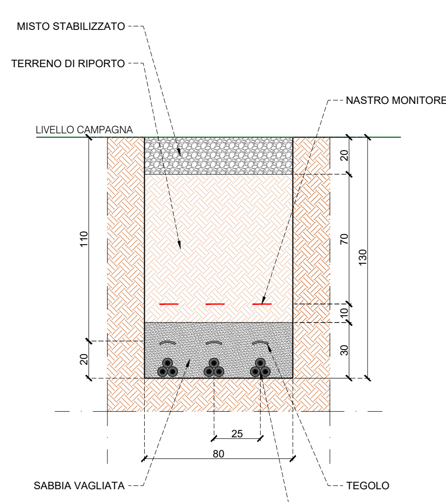
SEZIONE DI SCAVO AC 3
