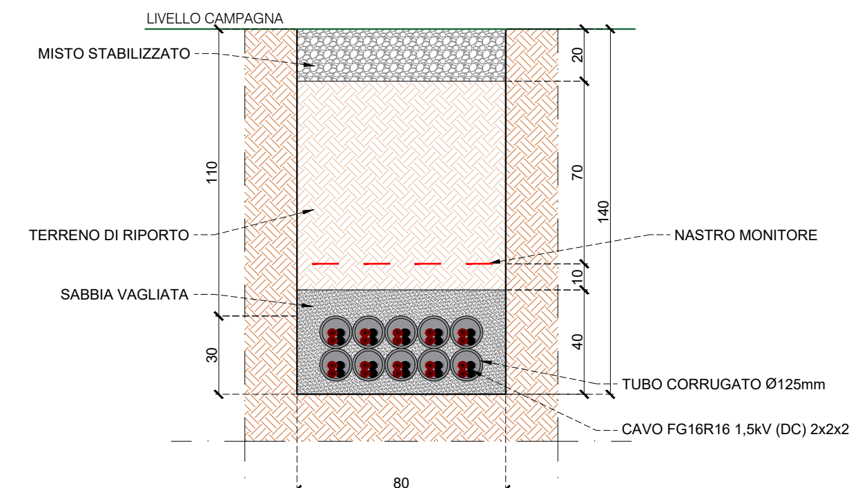
SEZIONE DI SCAVO DC 10
