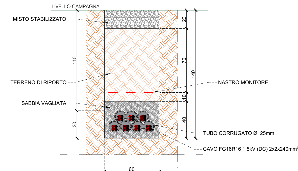
SEZIONE DI SCAVO DC 7
