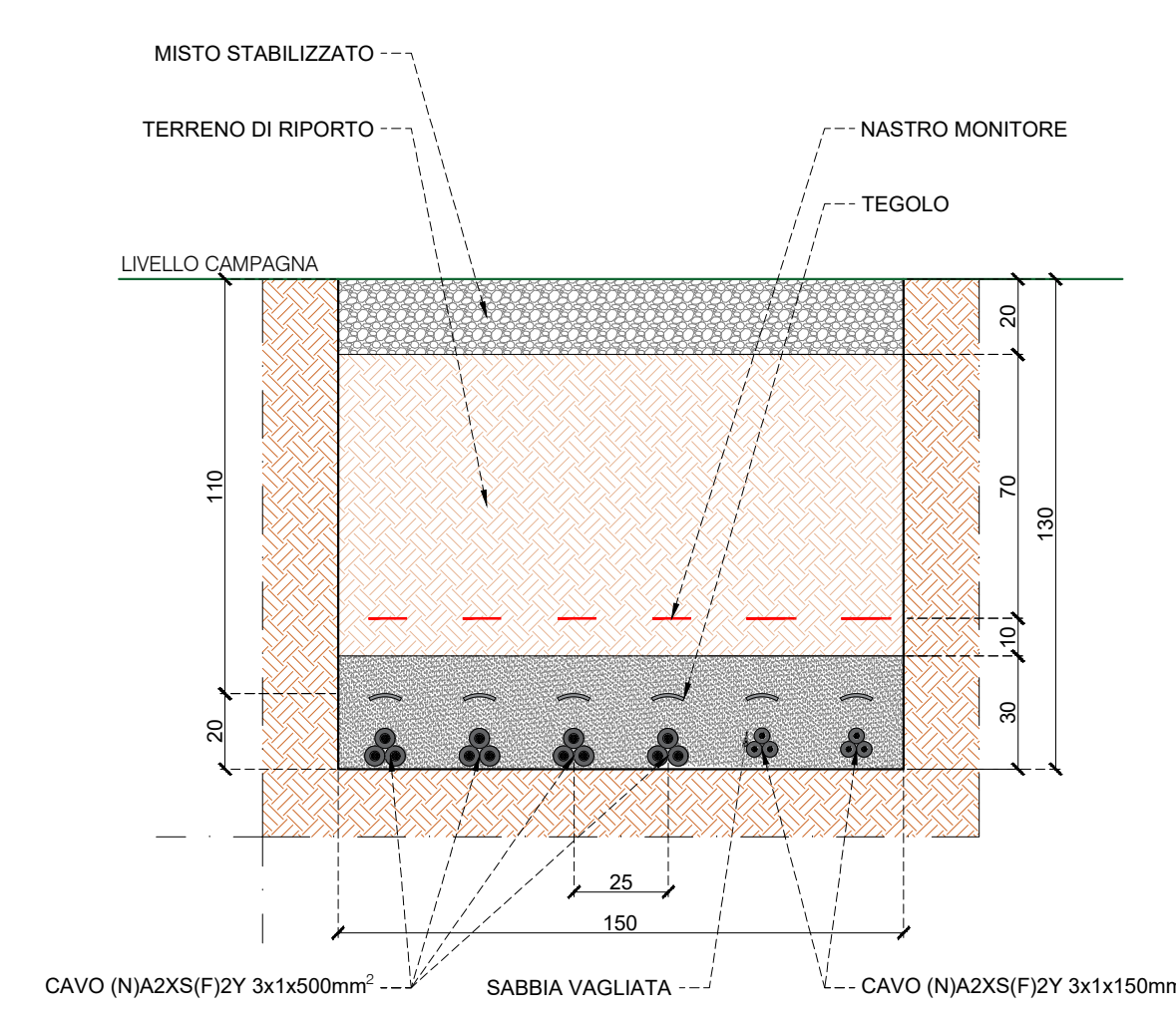
SEZIONE DI SCAVO AC 6
