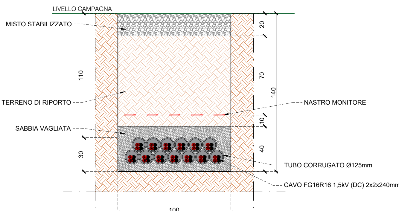
SEZIONE DI SCAVO DC 13
