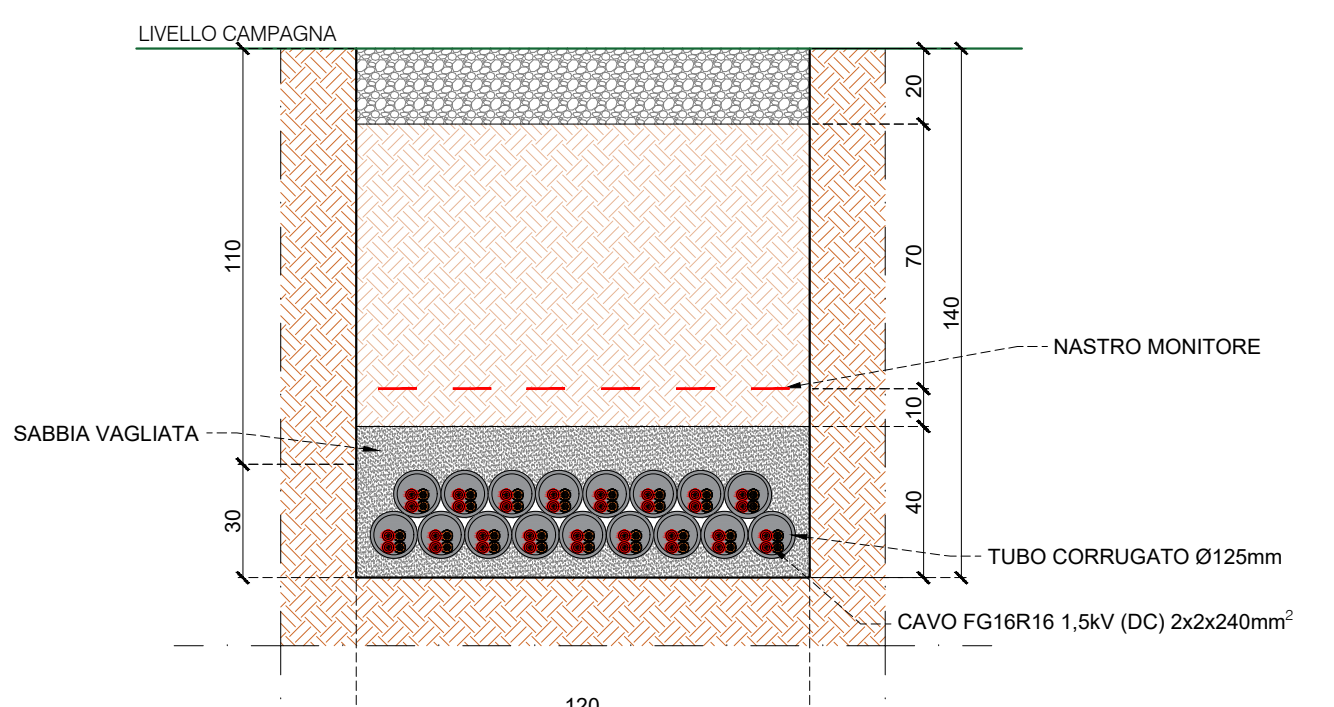
SEZIONE DI SCAVO DC 17
