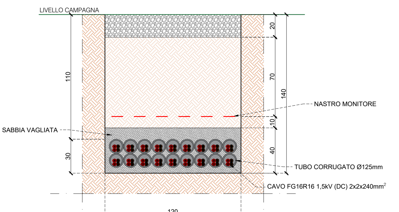
SEZIONE DI SCAVO DC 18
