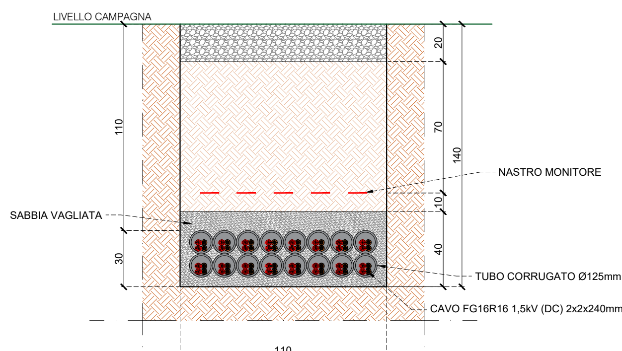
SEZIONE DI SCAVO DC 16
