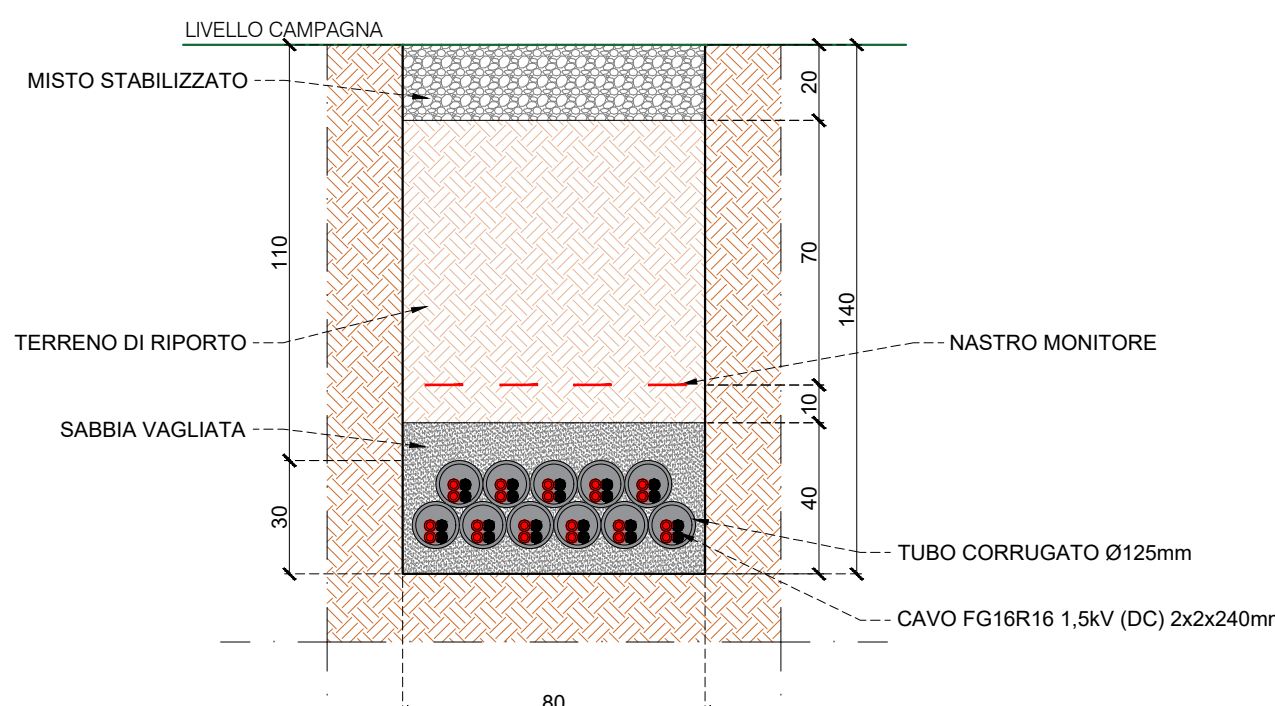
SEZIONE DI SCAVO DC 11
