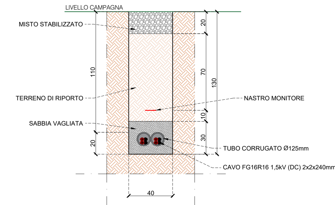
SEZIONE DI SCAVO DC 2
