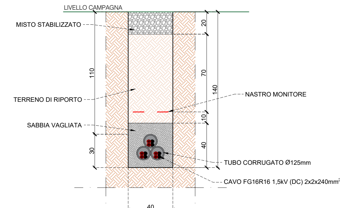
SEZIONE DI SCAVO DC 3
