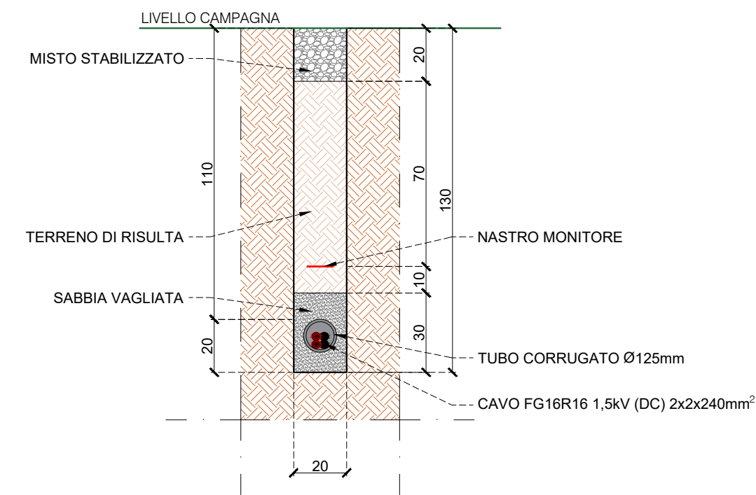
SEZIONE DI SCAVO DC 1
