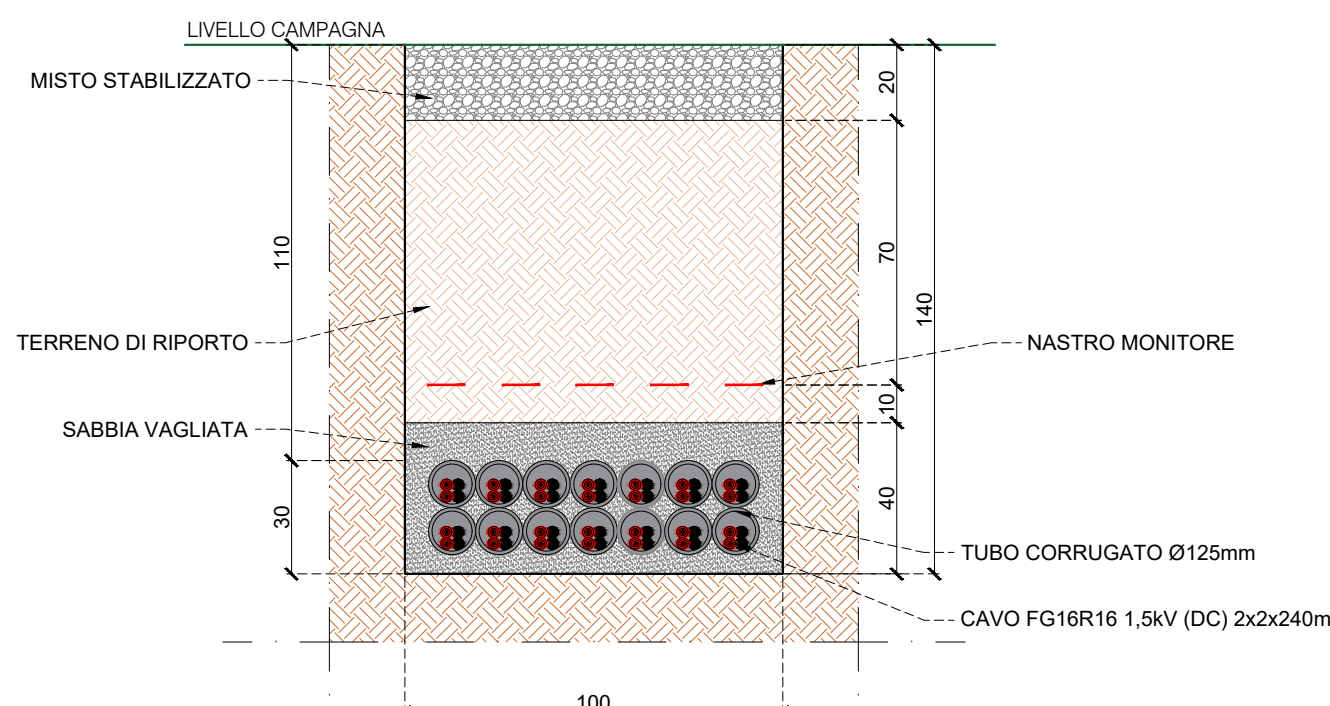
SEZIONE DI SCAVO DC 14
