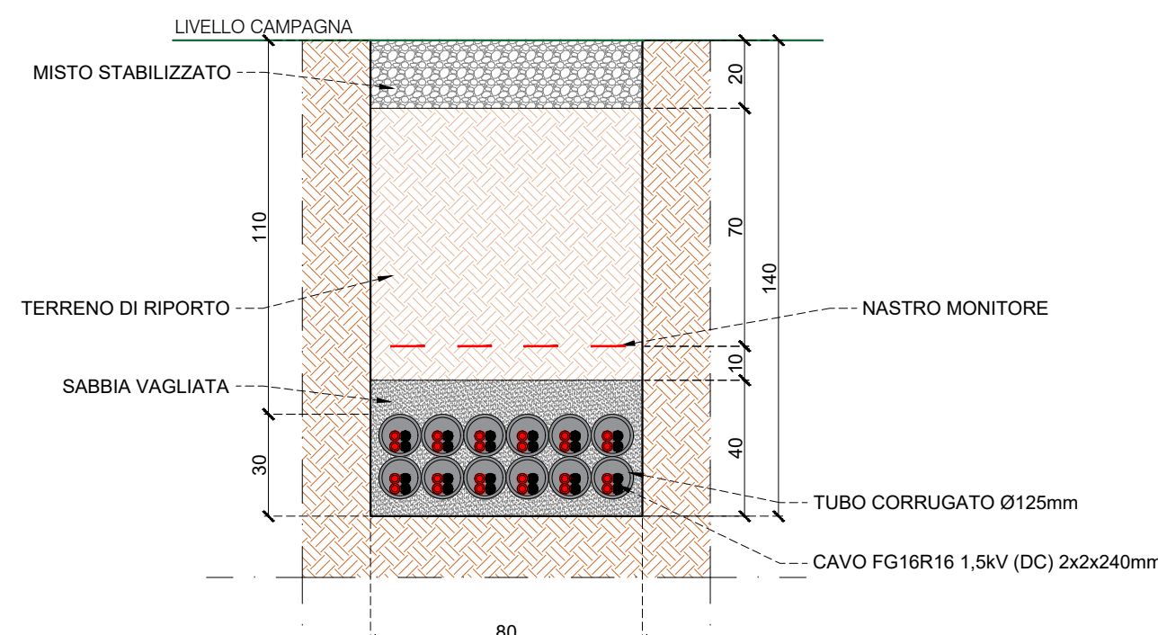
SEZIONE DI SCAVO DC 12
