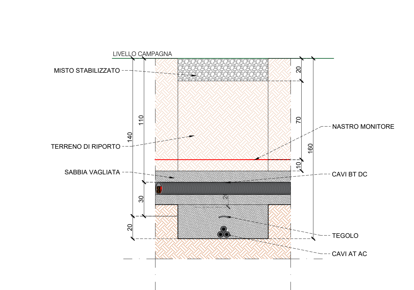
VISTA SEZIONE DI SCAVO AT AC
