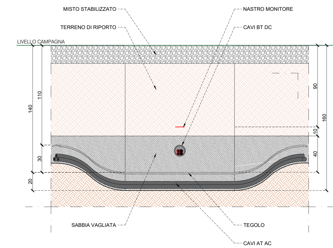
VISTA SEZIONE DI SCAVO BT DC
