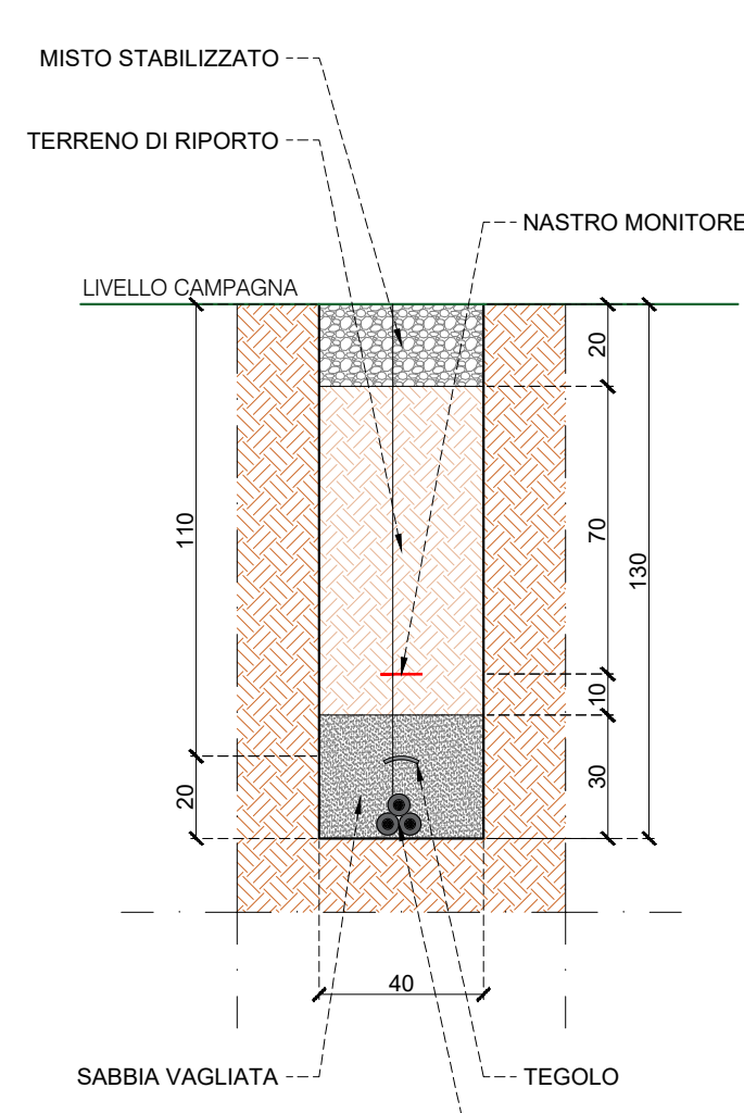
SEZIONE DI SCAVO AC 1
