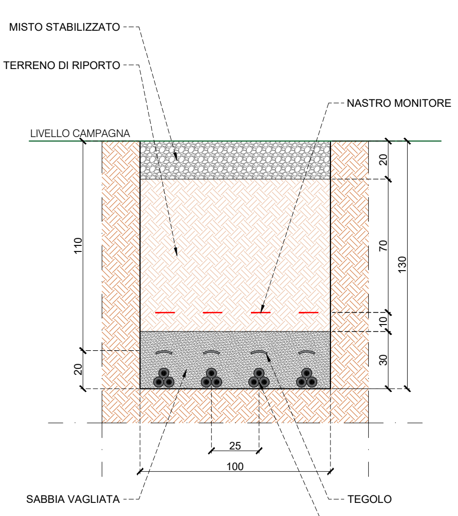
SEZIONE DI SCAVO AC 4
