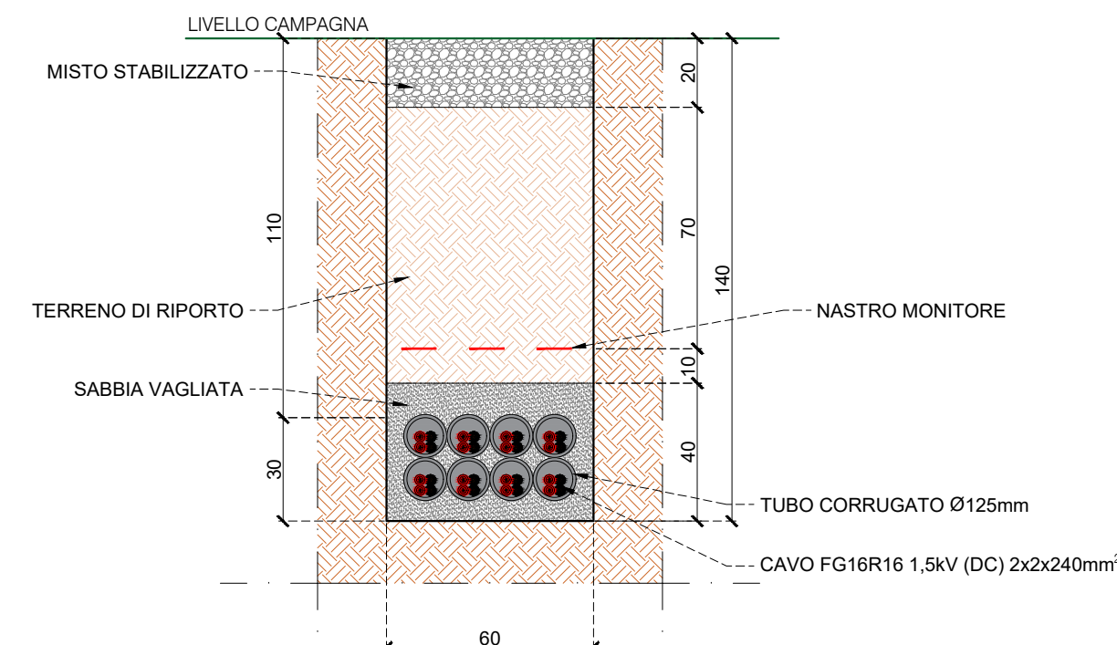
SEZIONE DI SCAVO DC 8
