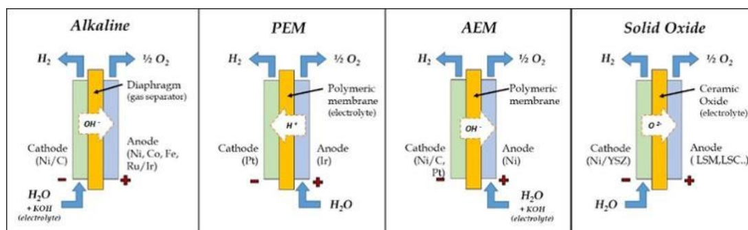
Figura 1 - Struttura della cella per le quattro principali tecnologie di elettrolisi. Fonte: S.Campanari, P. Colbataldo, G. Guandalini "Power to Hydrogen", in: Small Scale Power Generation Handbook , Elsevier, in press.
