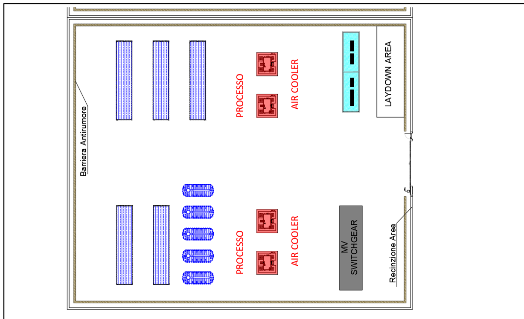
Figura 5 - Vista del sistema di accumulo idrogeno verde
