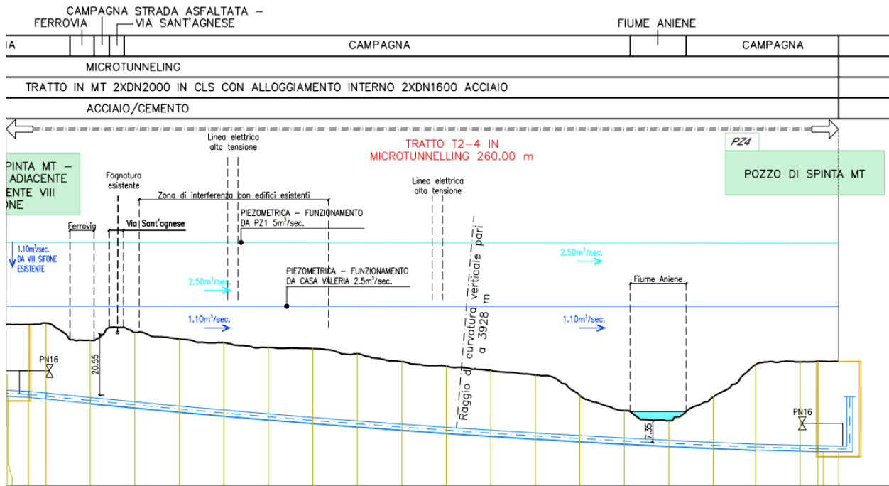
Figura 3.2 – Profilo in asse al tratto T2-4 in microtunneling
