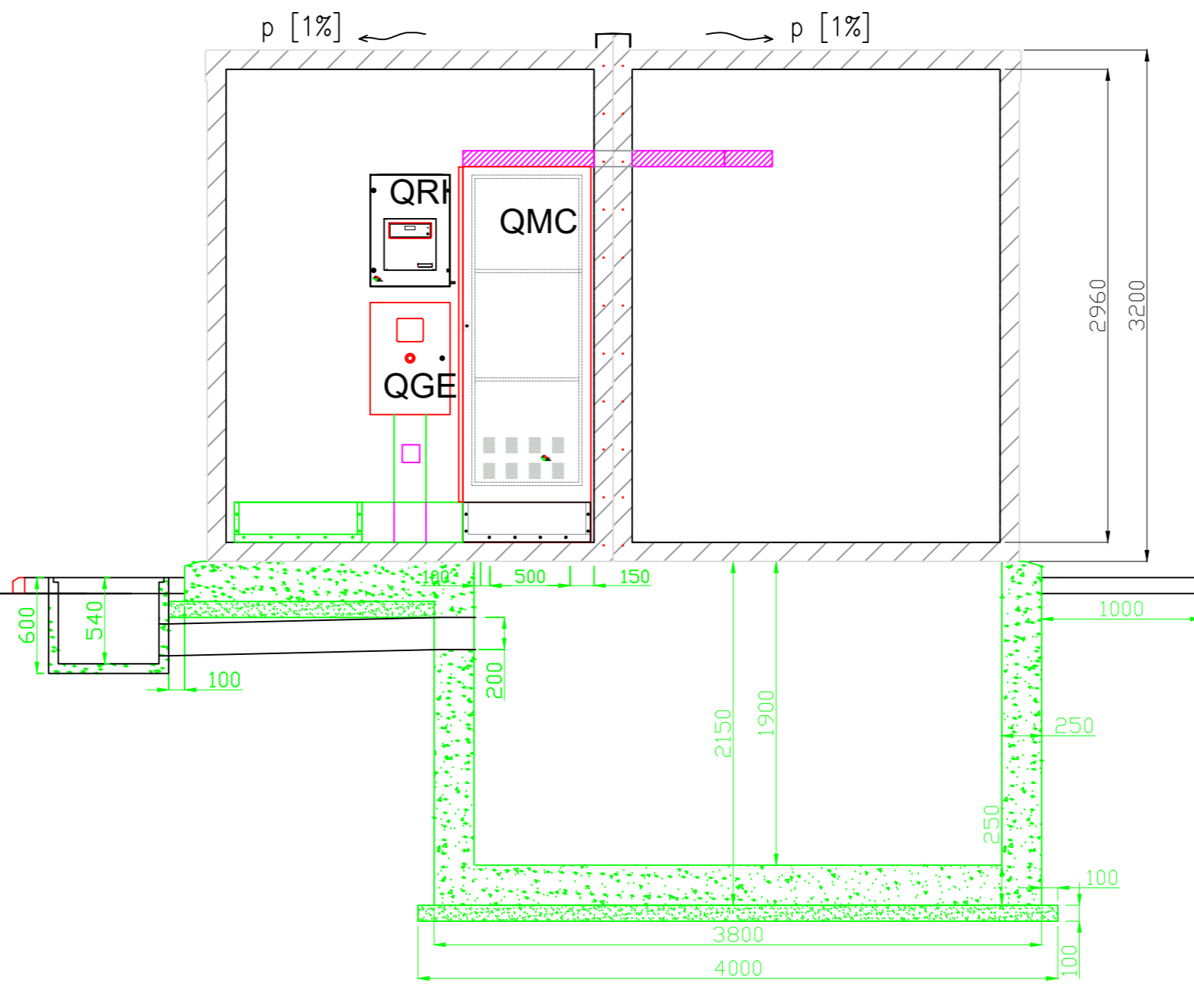
SEZIONE CC'
