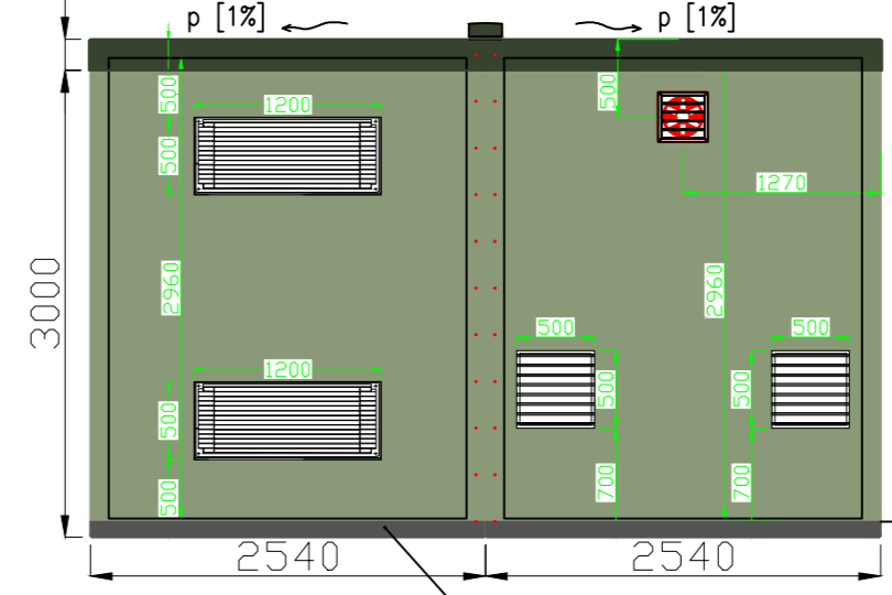
PROSPETTO FRONTALE LATO BOX MT
