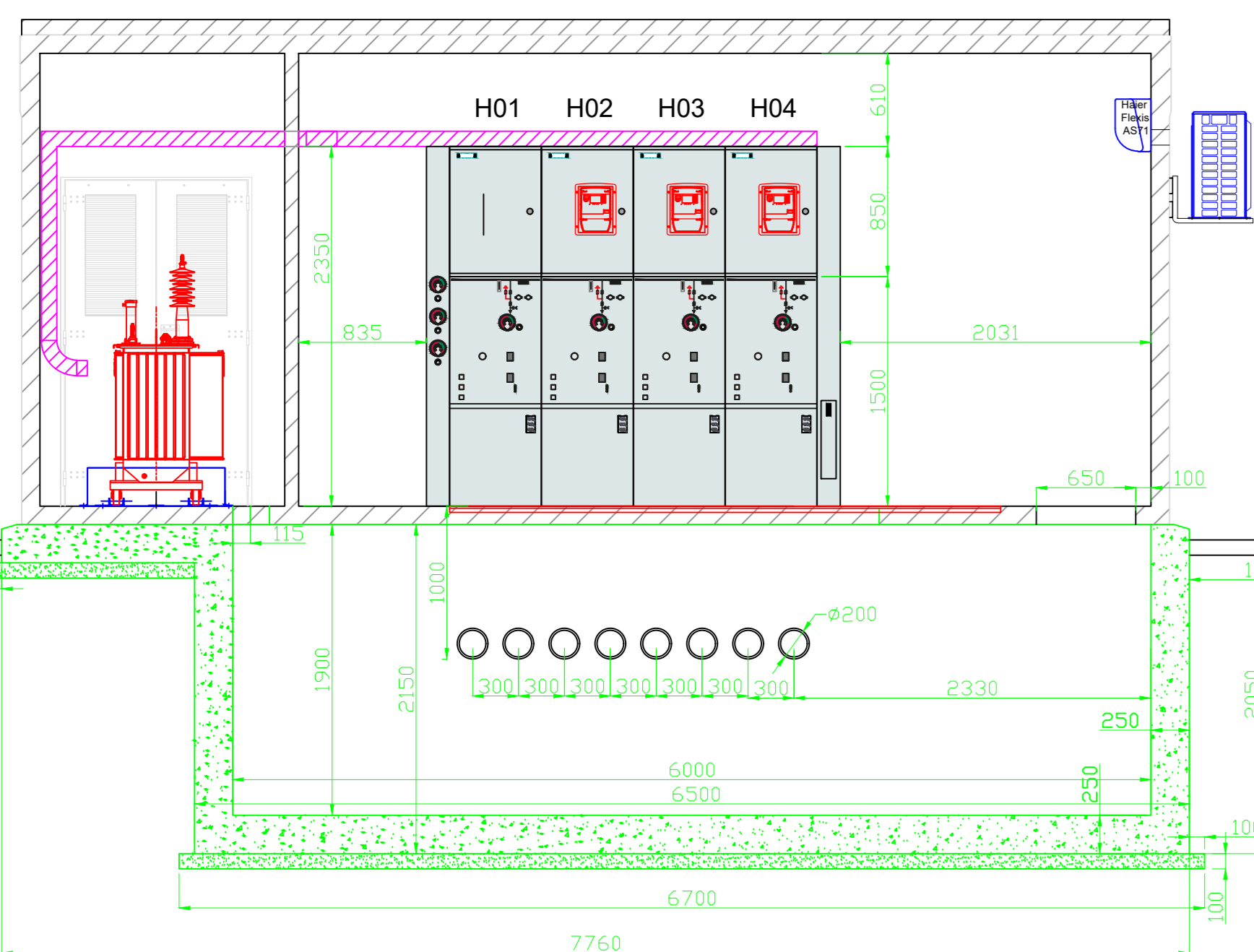
SEZIONE AA'
