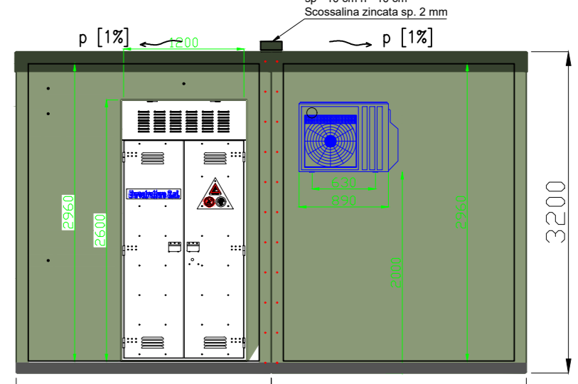
PROSPETTO LATERALE DX
