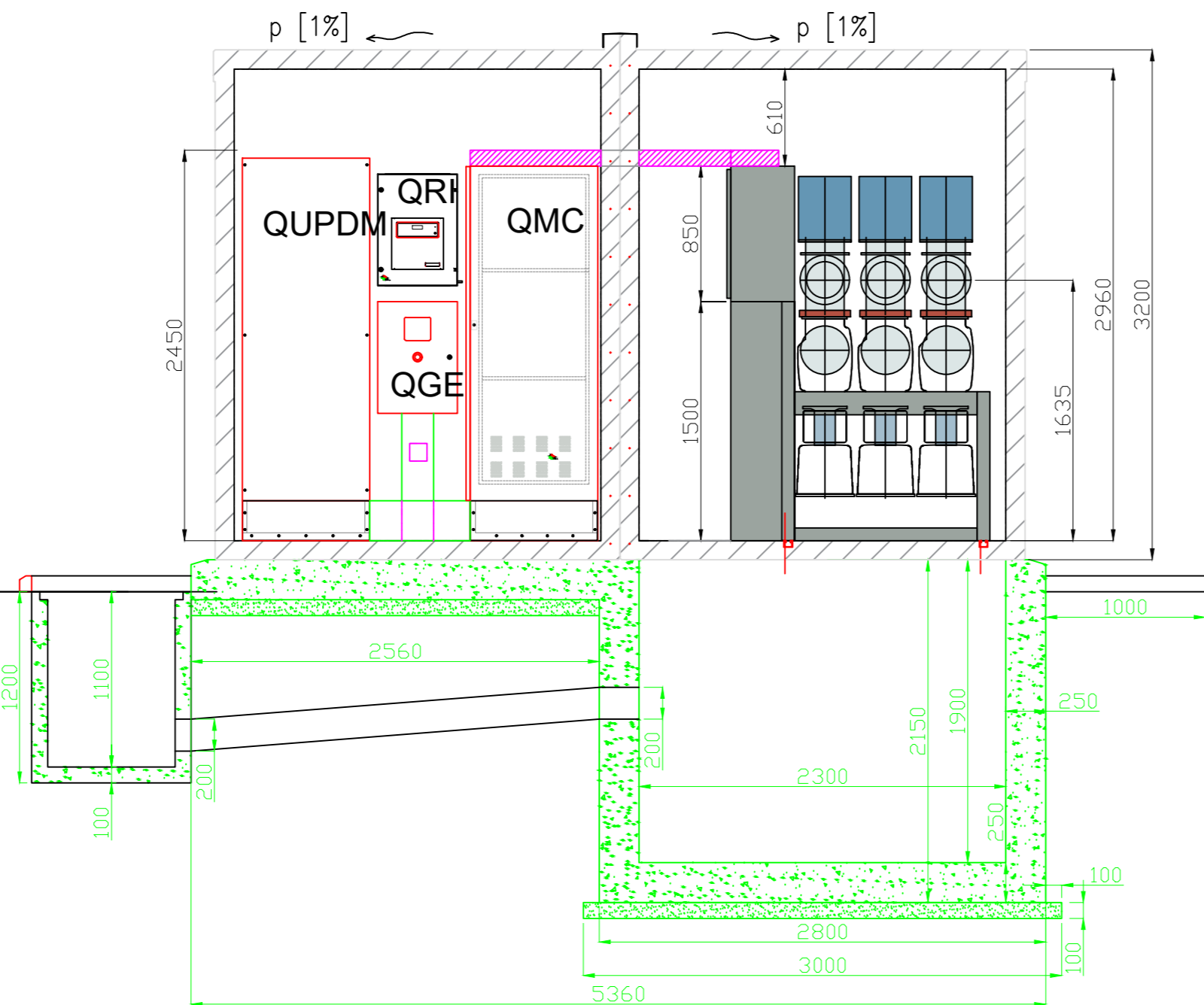
SEZIONE BB'
