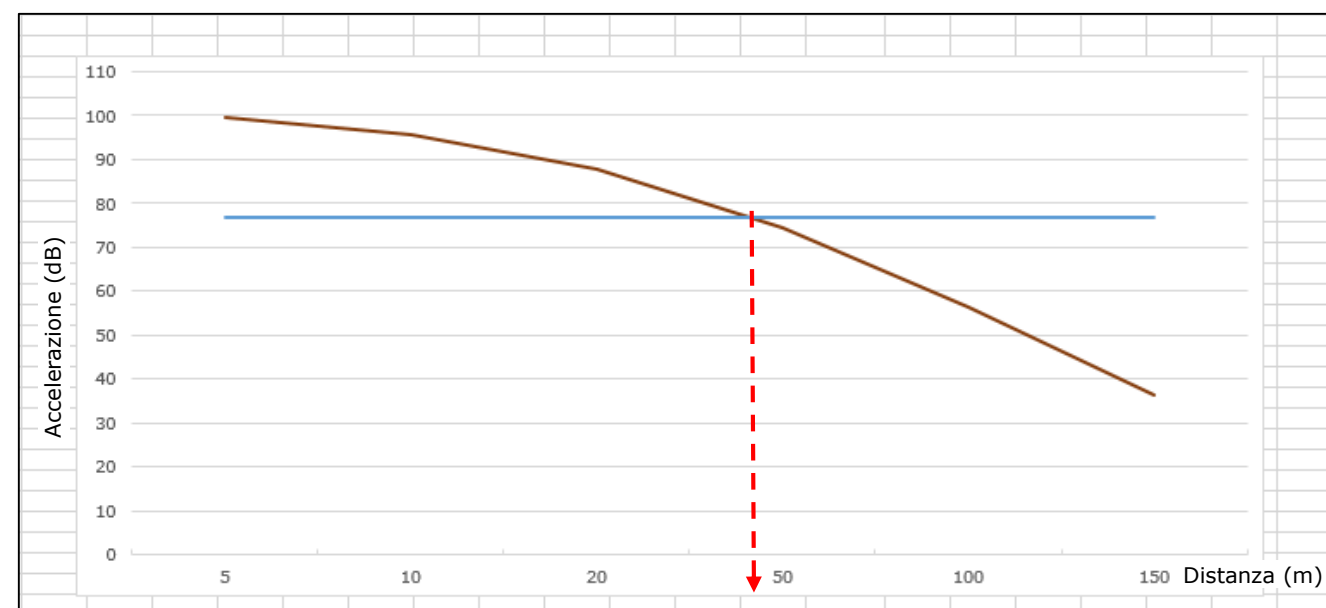
— Livelli stimati — Valore limite (UNI 9614)
