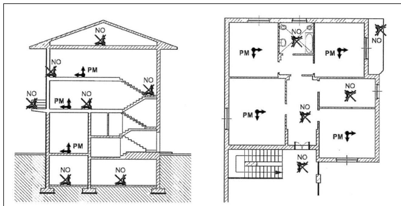
Fig.4 - Individuazione corretta e non corretta dei punti di misura
