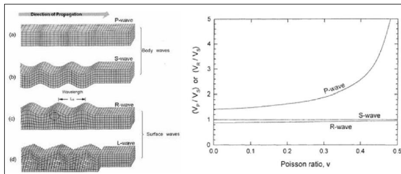
Fig.6 - Tipi di onda di volume e di superficie (a sinistra) e velocità relative delle onde P, R rispetto onde S (a destra)
