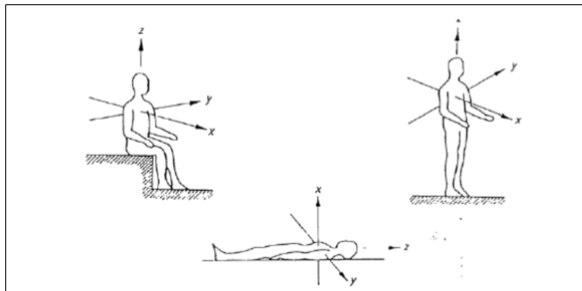
Fig.2 - Assi standard di propagazione delle vibrazioni per le varie posture
