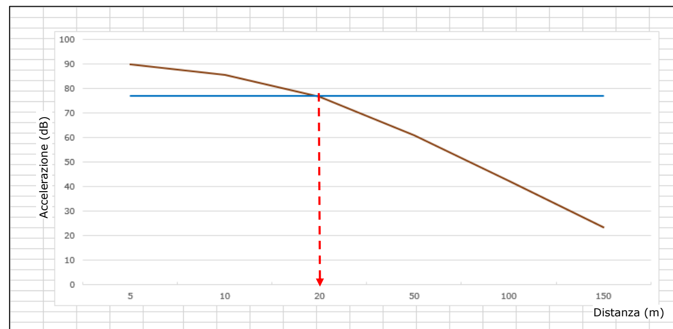
— Livelli stimati — Valore limite (UNI 9614)
