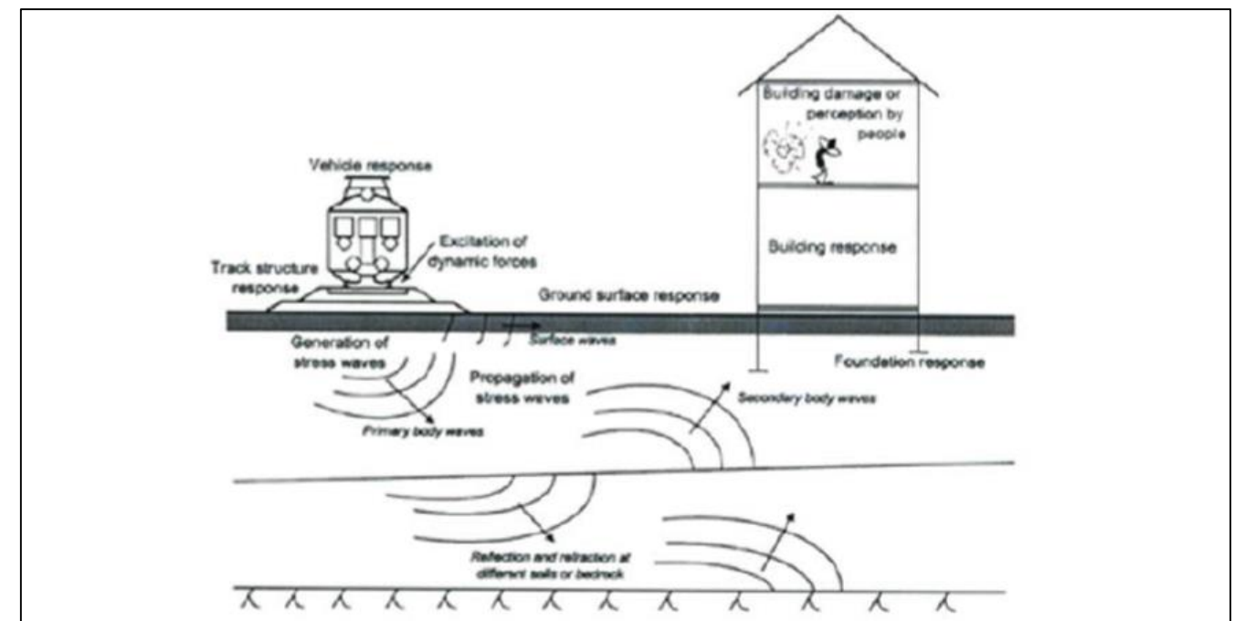
Fig.1 - Schematizzazione della generazione e propagazione di fenomeni vibratorii
