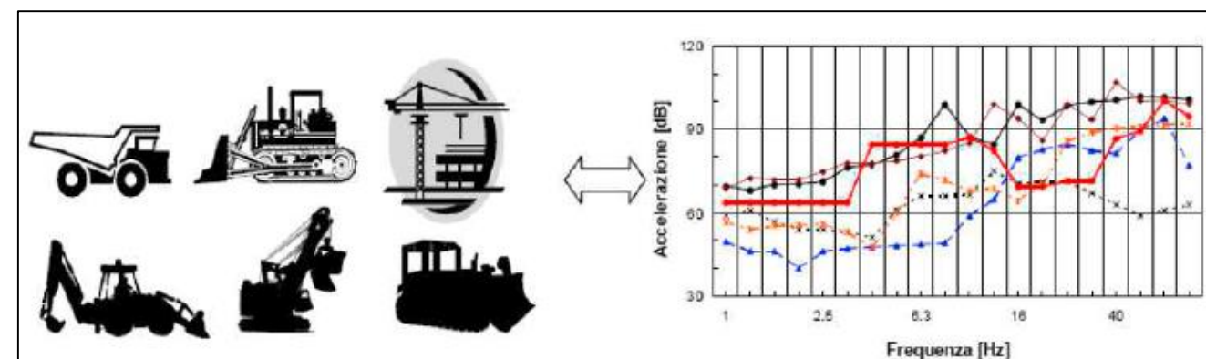
Fig.5 - Relazione tra mezzi d'opera e spettro di emissione delle vibrazioni
