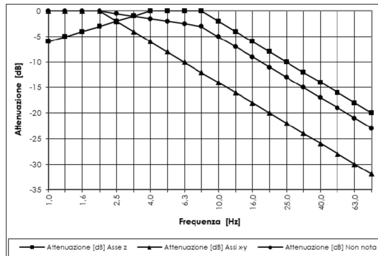
Fig.3 - Curve di ponderazione delle vibrazioni
