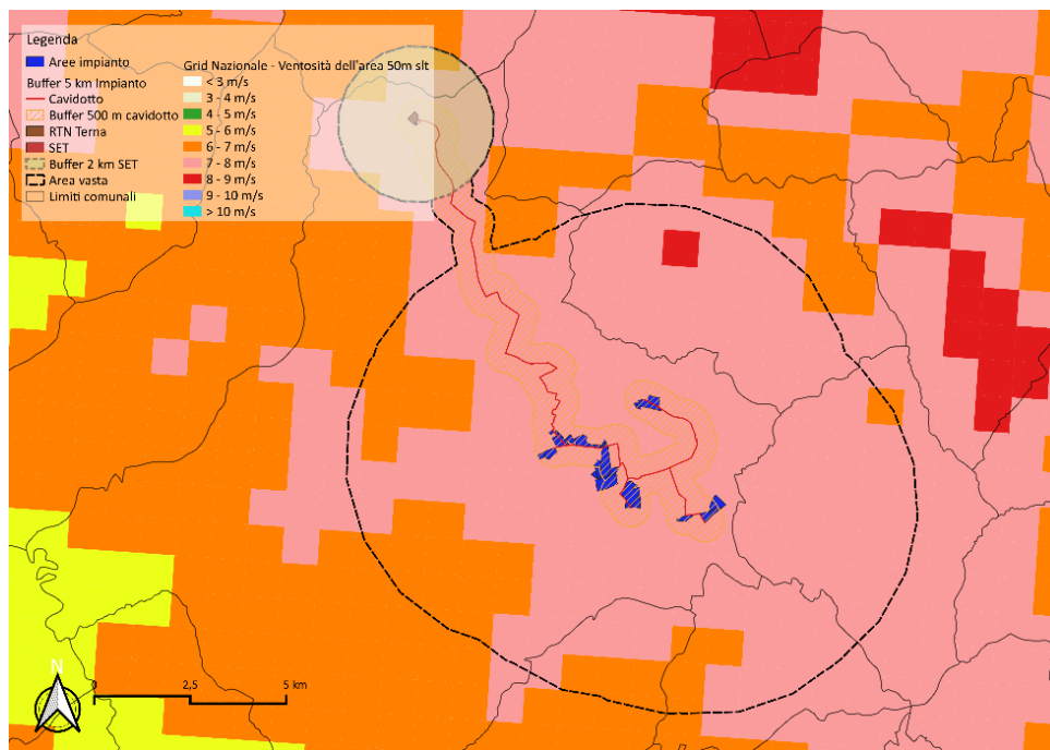
Figura 3: Ventosità dell'area - 50 m s.l.t.
