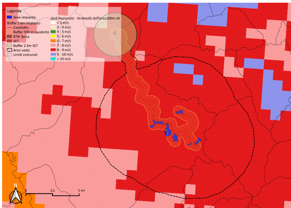
Figura 5: Ventosità dell'area - 100 m s.l.t.
