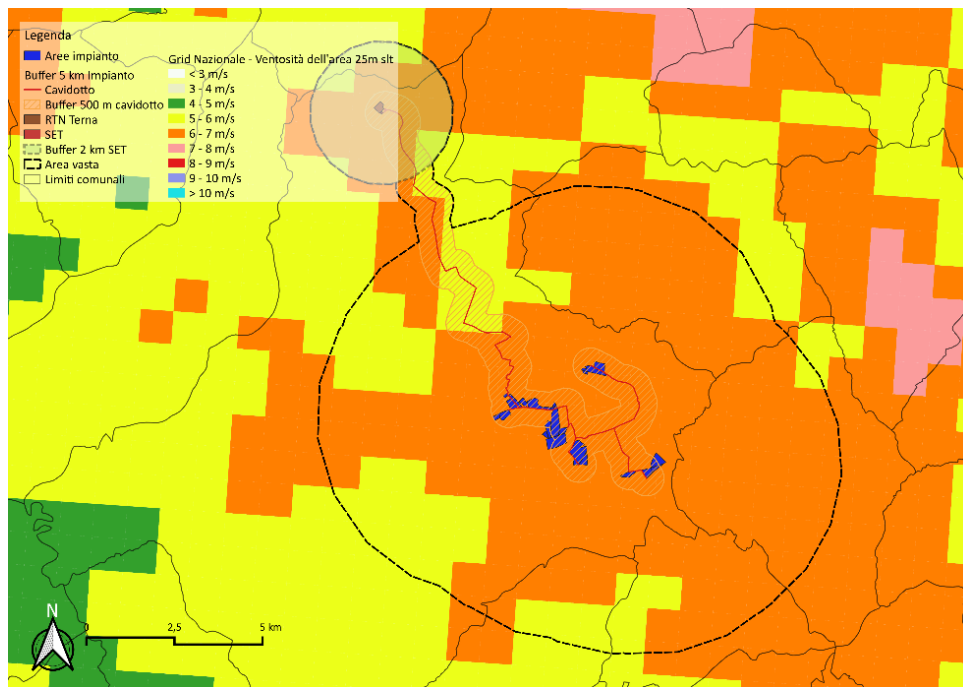
Figura 2: Ventosità dell'area - 25 m s.l.t.
