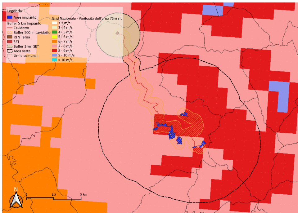
Figura 4: Ventosità dell'area - 75 m s.l.t.
