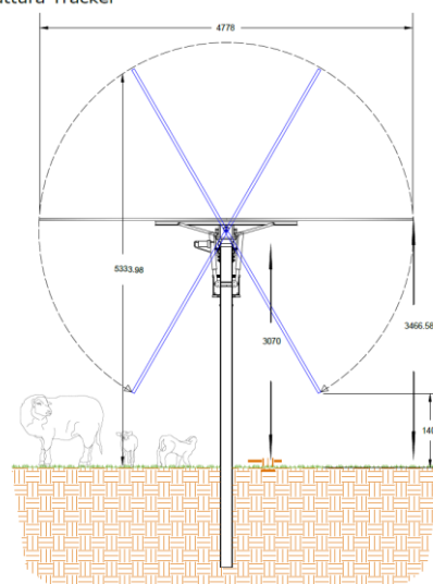
Particolari Struttura Tracker
