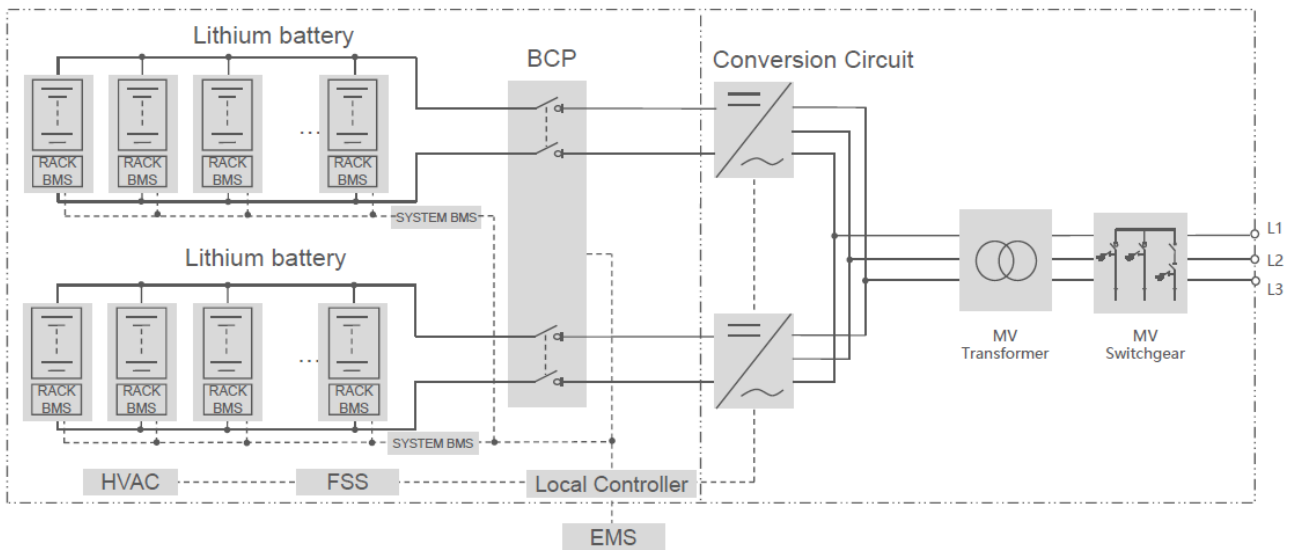
Figura 7 – Schema Elettrico di Collegamento
