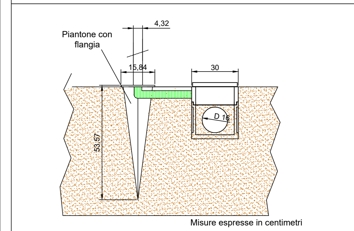
Particolare ancoraggio palo + pozzetto
