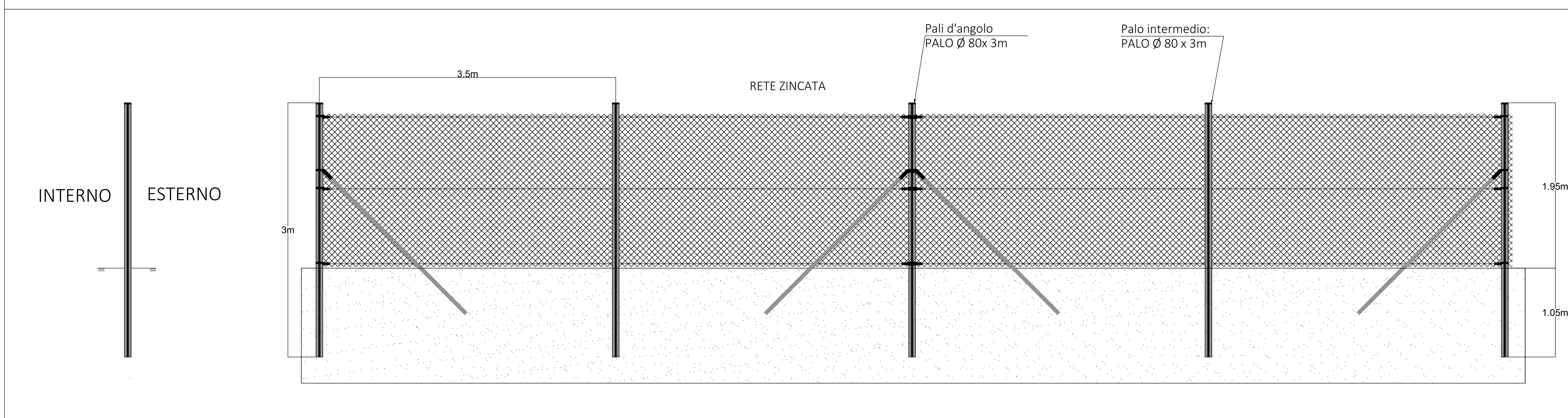
Particolare recinzione
