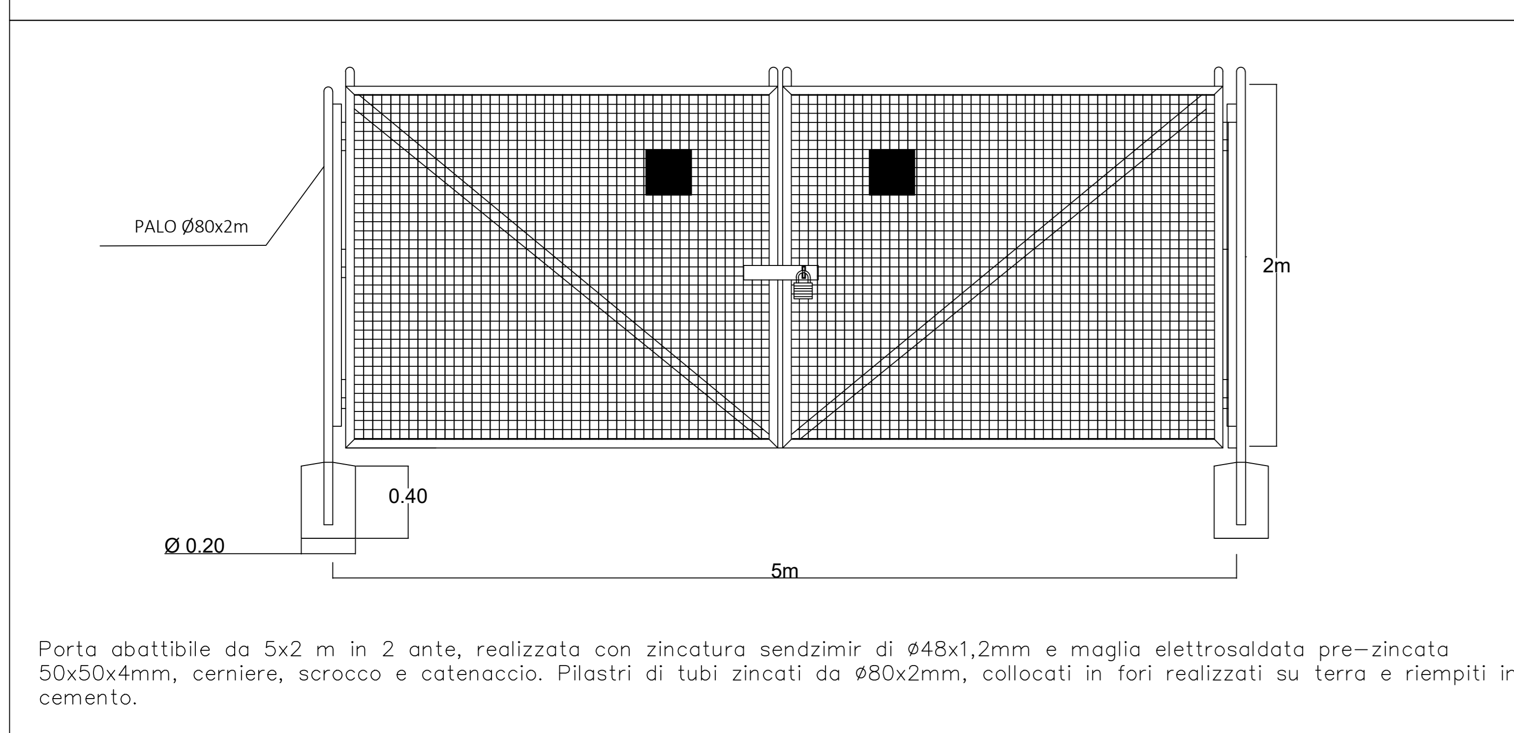
Particolare cancello
