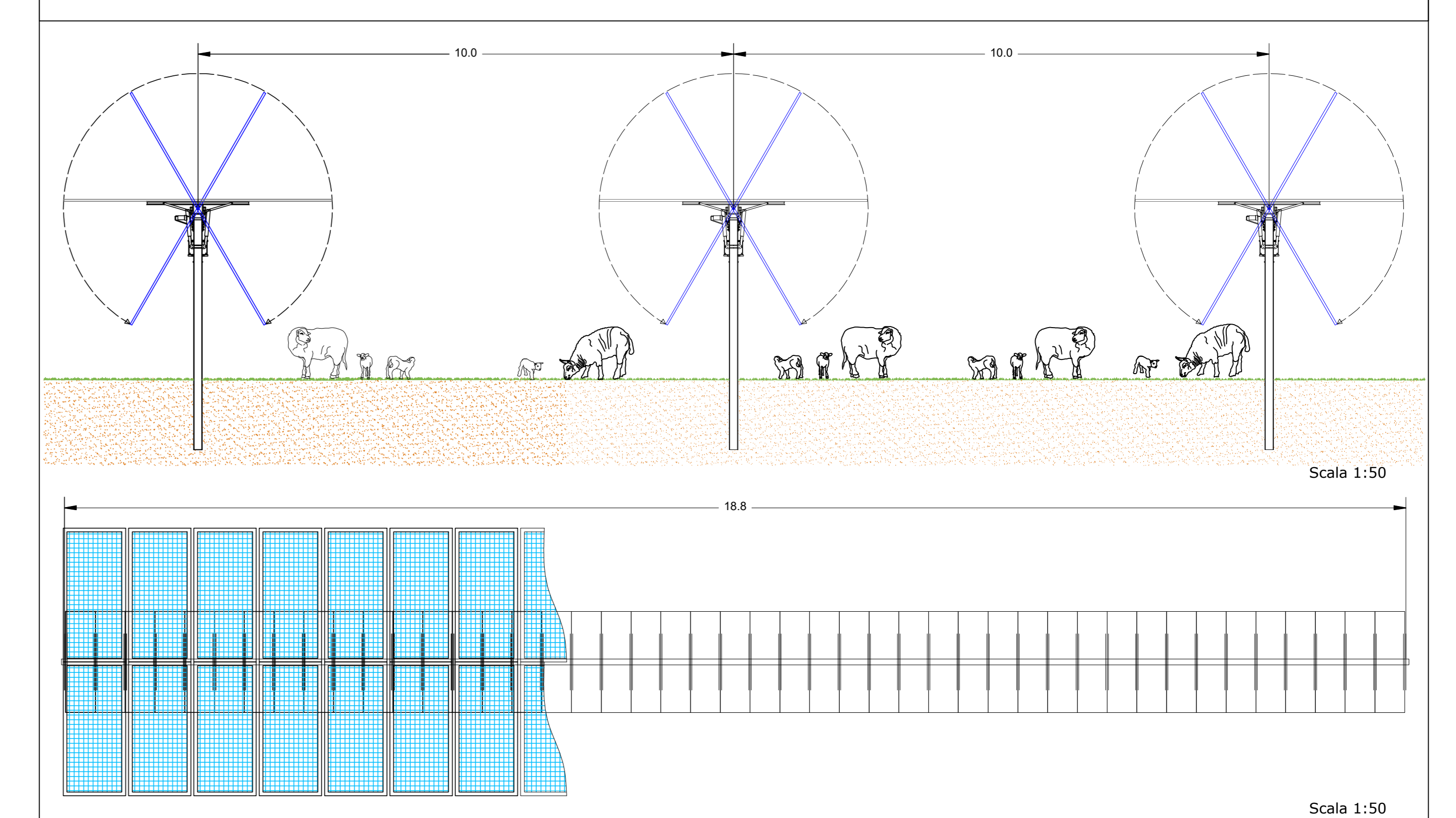
Particolari struttura Tracker
