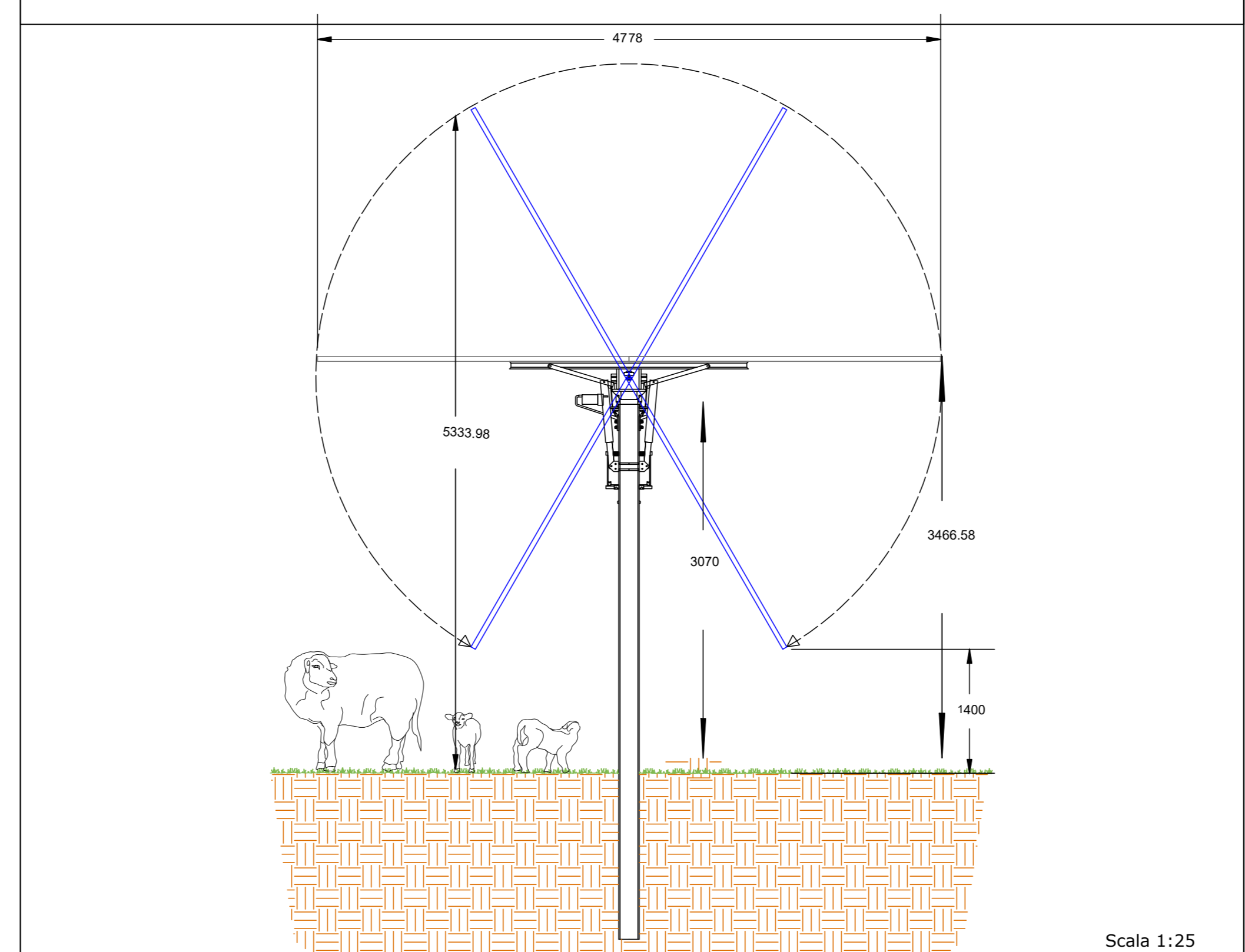
Particolari struttura Tracker
