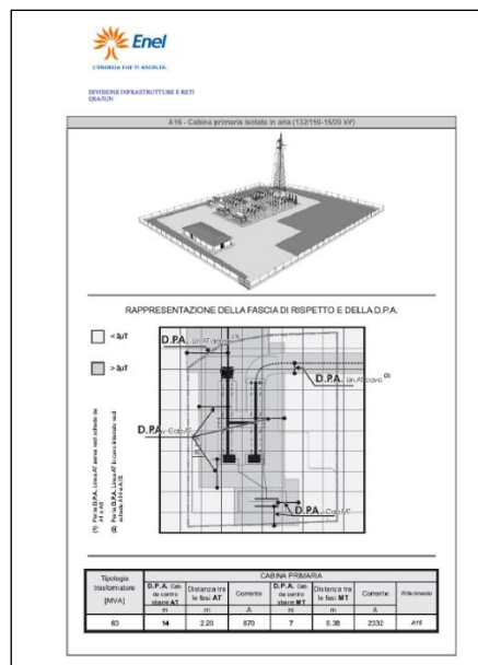
Figura 21: DPA Cabine Primarie Enel equipaggiate con n° 2 trasformatori da 63 MVA
