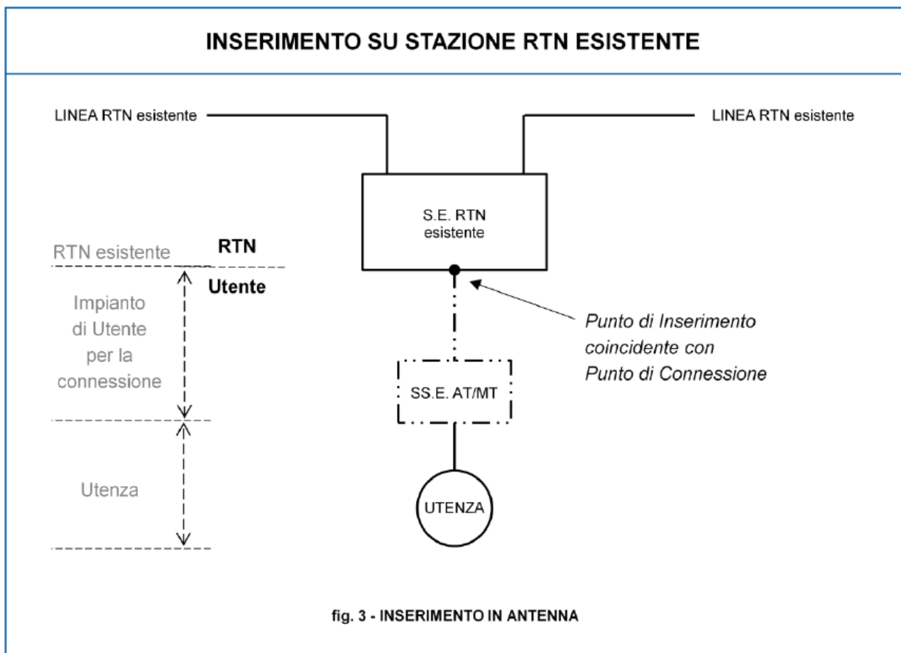
Figura 2: schema di inserimento in antenna con la sezione a 150 kV di una Stazione Elettrica RTN
