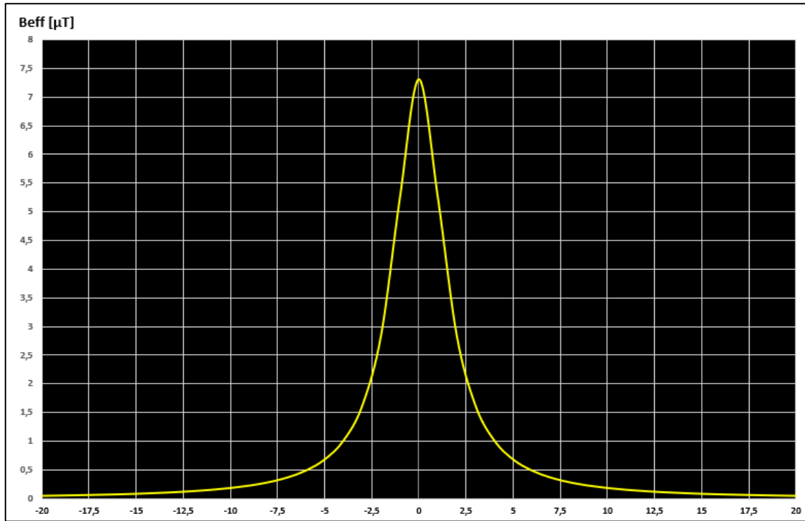
Figura 23: Induzione Magnetica generata dal cavo durante l'esercizio, valutata lungo l'asse della linea in corrispondenza della superficie del suolo
