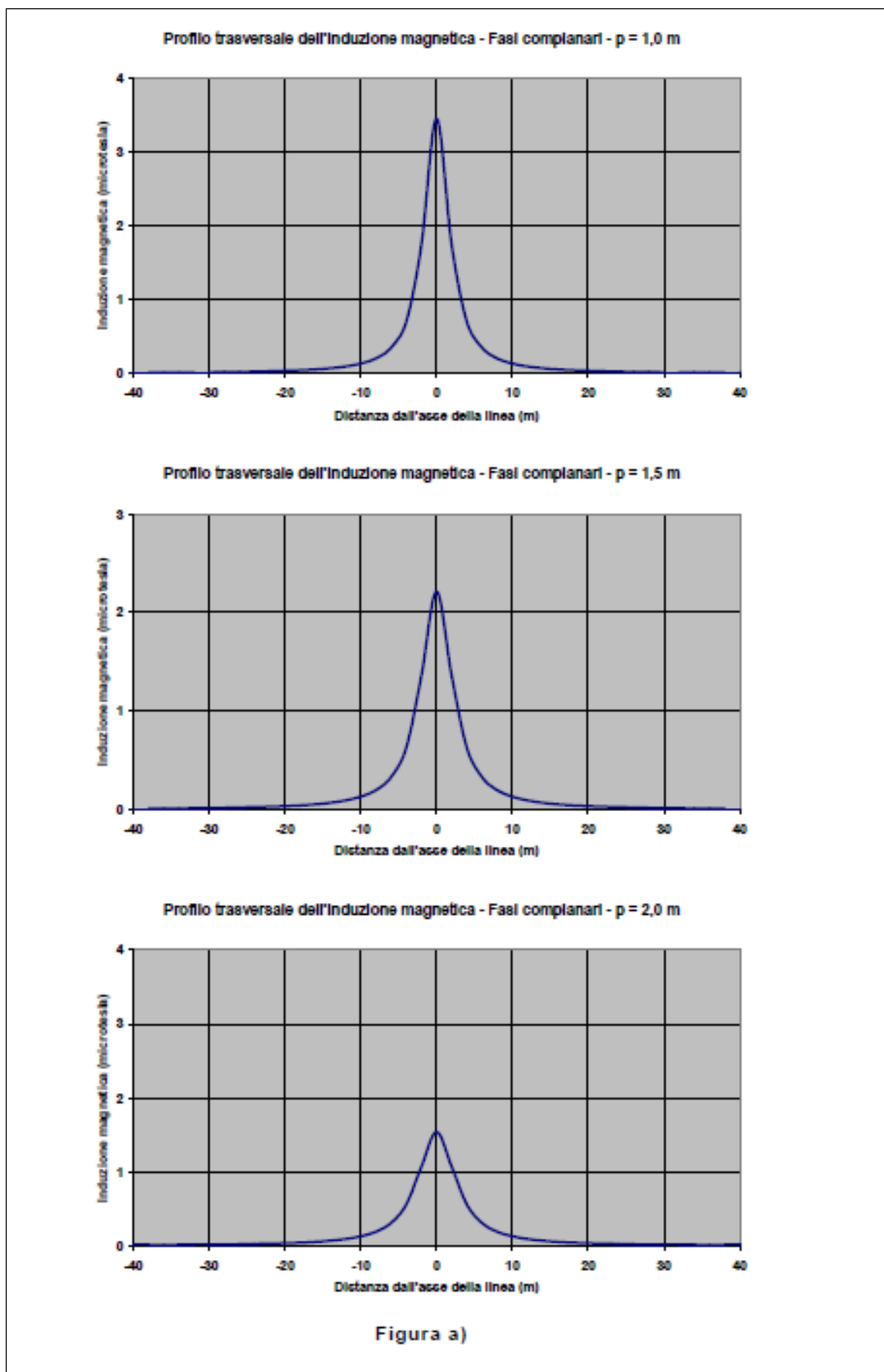
Figura 17: andamento del Campo Induzione Magnetica generata a livello del suolo sulla verticale del cavo – linea trifase con conduttori distanziati di 0,20 m posati rispettivamente a 1,00 m, 1,50 m e 2,00 m di profondità, paralleli tra loro e alla superficie di calpestio; corrente di ogni fase pari a 200 A.
