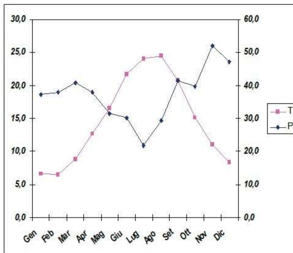
Figura - Diagramma bioclimatico di Bagnouls & Gaussen relativo alla stazione di Foggia.
